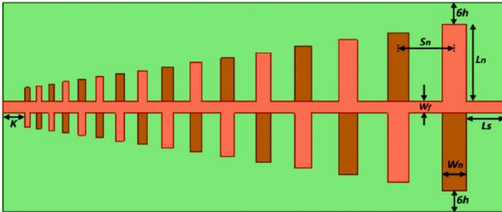
Şekil 7.1. Mikroşerit log-periyodik dipol anten dizisi
