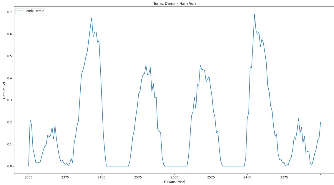
Şekil 4.2. Temiz inşaat çeliği cevap işareti grafiği
