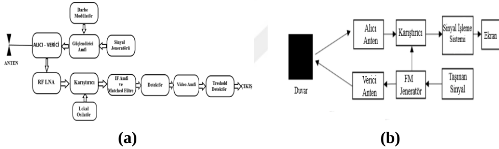
Şekil 2.4. a) SD radar blok diyagram; b) FMSD radar blok diyagram
