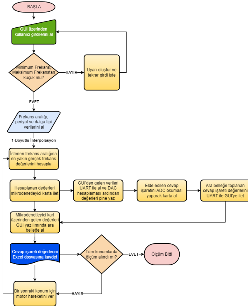
Şekil 3.12. FMSD radar yazılımı akış diyagramı
