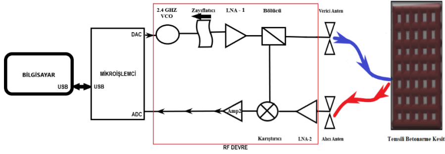
Şekil 2.7. FMSD radar blok şeması
