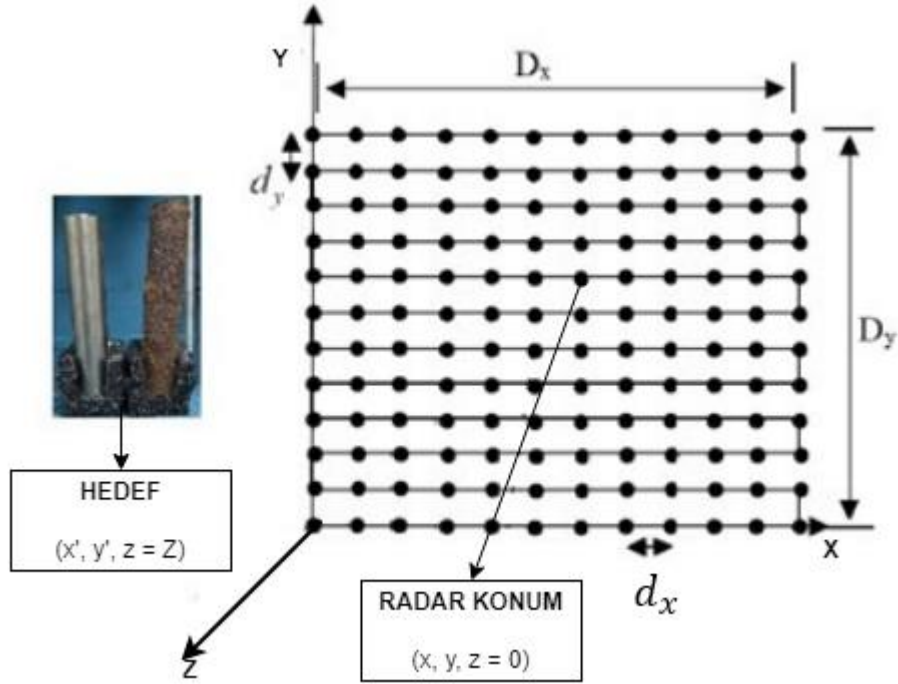
Şekil 3.8. İki boyutlu tarama görünümü
