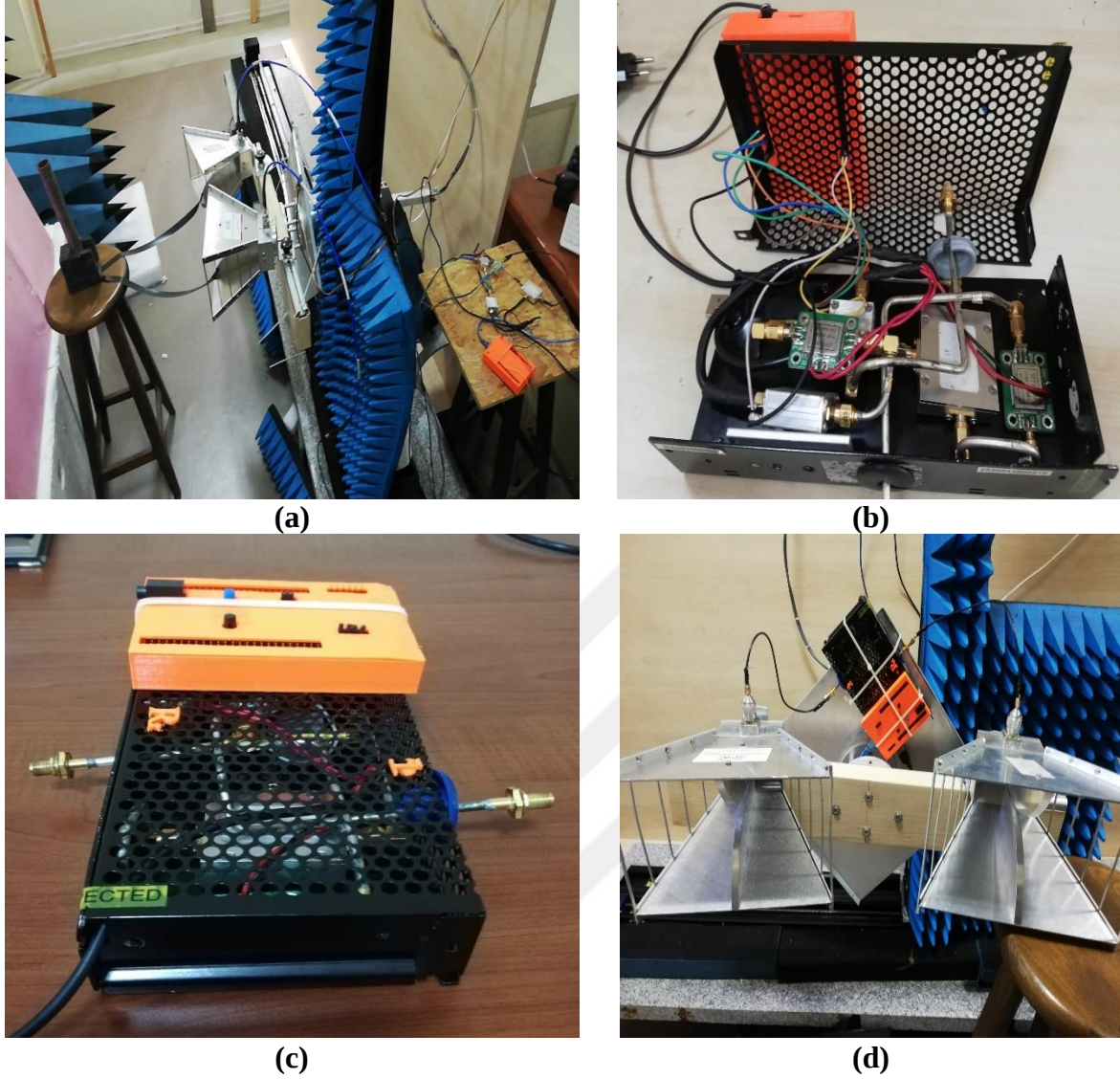
Şekil 3.3. FMSD radar süreçleri; a) Doğrulama ölçümleri; b) RF devre kutulanması; c) FMSD radar son hal; d) FMSD radar anten ve platform bağlantısı
