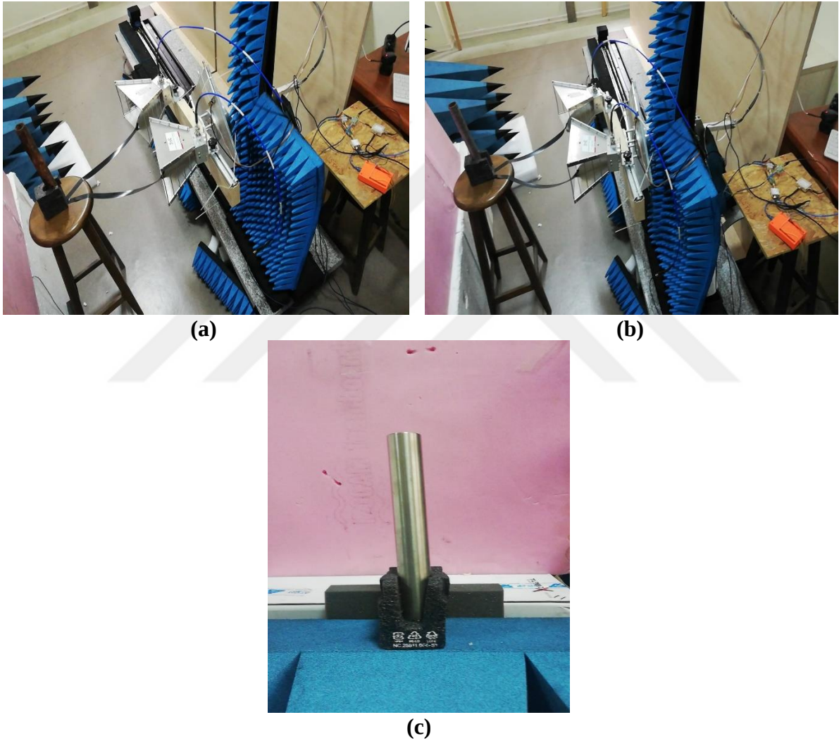
Şekil 3.6. Laboratuvar ölçümleri; a) Yüksek seviye korozyonlu demir silindir ölçümü; b) Orta seviye temiz demir silindir ölçümü; c) Temiz demir silindir ölçümü
