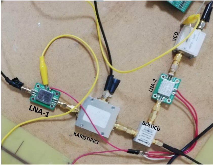
Şekil 3.2. RF devre gerçekleştirilmesi
