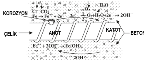
Şekil 1.1. Beton içerisindeki çeliğin korozyona uğrama süreci (Ahmad,2003)
