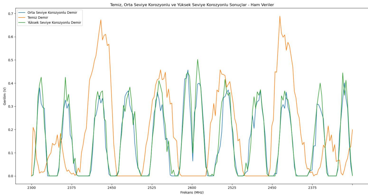
Şekil 4.3. Temiz demir, orta seviye korozyona uğramış demir, yüksek seviye korozyona uğramış demir cevap işaretleri ham verileri arasında karşılaştırma grafiği
