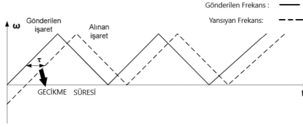
Şekil 2.3. FMSD radar kavramı
