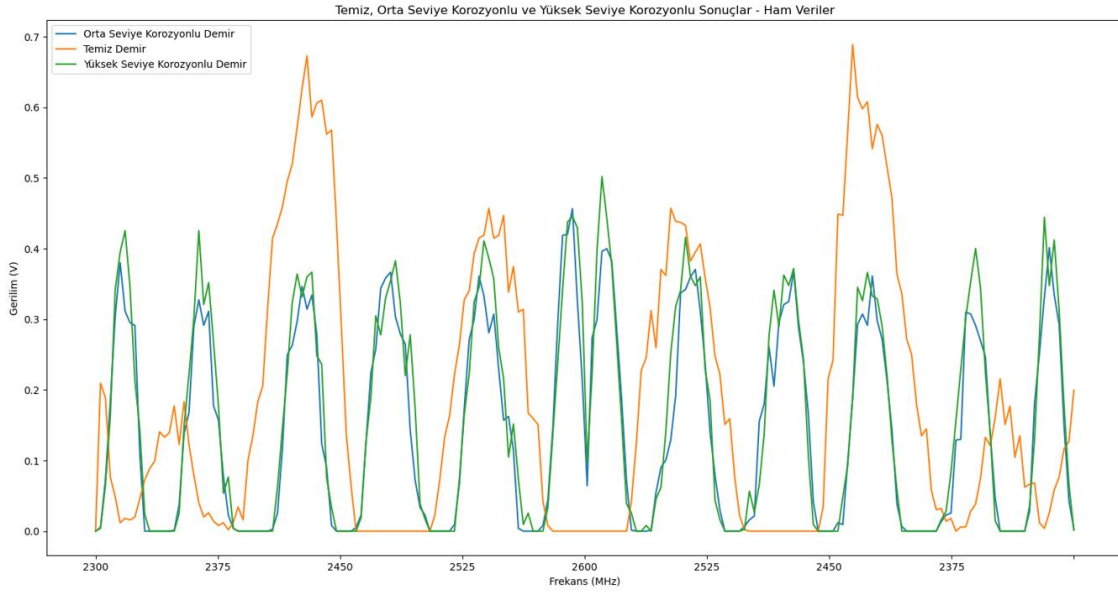
Şekil 3.7. Tek nokta ölçüm sonucu
