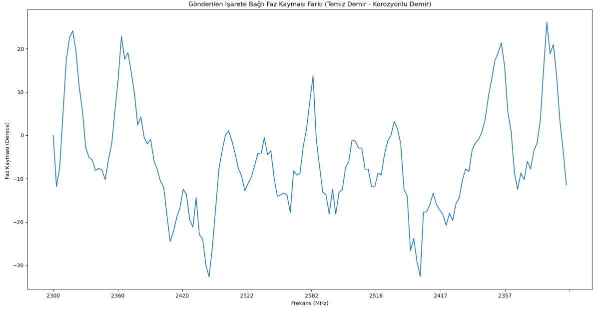
Şekil 4.7. Korozyona uğramış inşaat çeliği ve temiz durumdaki inşaat çeliği arasında faz kayması fark sonuçları
