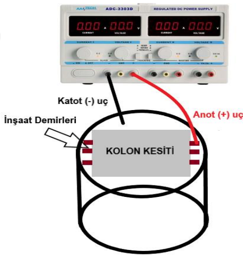
Şekil 2.9. HKT düzeneği
