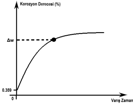
Şekil 2.5. Zamana bağlı korozyon derecesi
