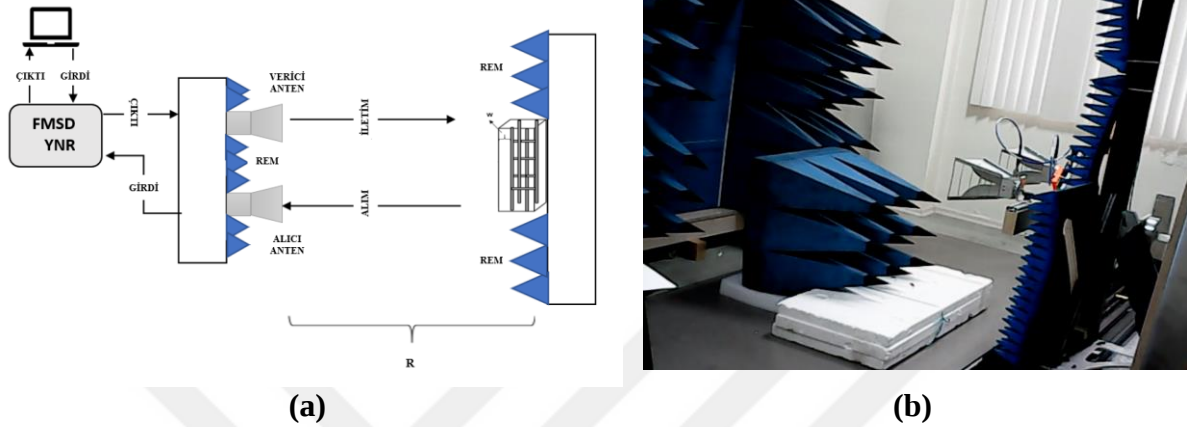
Şekil 3.4. Ölçüm düzeneği; a) Ölçüm düzeneği blok şeması; b) Ölçüm düzeneği laboratuvar ortamı
