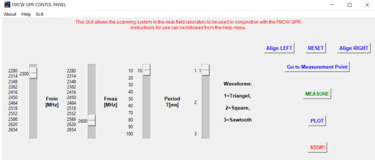
Şekil 3.10. 2-boyulu tarama arayüzü
