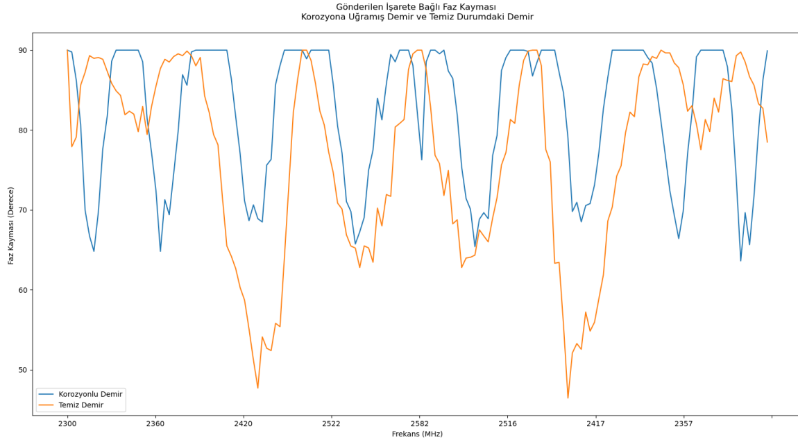
Şekil 4.6. Temiz inşaat çeliği cevap işareti ve korozyona uğramış inşaat çeliği cevap işareti arasında faz kayması karşılaştırma grafiği
