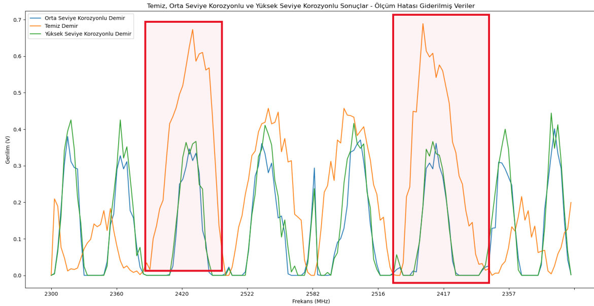
Şekil 4.4: Ölçüm hataları giderilmiş veriler arasında karşılaştırma grafiği
