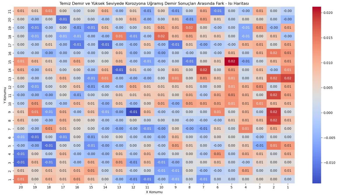
Şekil 4.12. Temiz demir ve yüksek seviyede korozyona uğramış demir sonuçları arasında farkın ısı haritasında gösterilmesi
