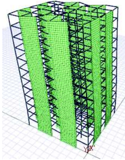
Şekil 4.43. Sistem 2'nin 1. Mod hali.
