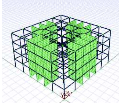
Şekil 4.14. Sistem 3 3B çubuk model.
