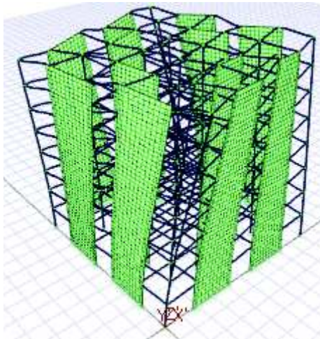
Şekil 4.29. Sistem 2'nin 3. Mod hali.
