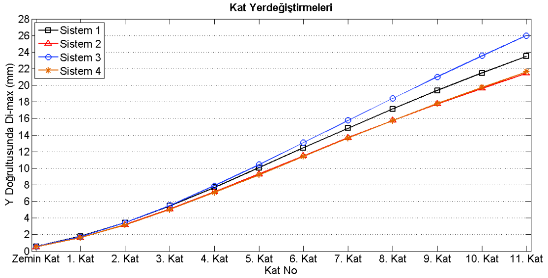
Şekil 5.51. 8 katlı sistemlerin Y doğrultusundaki yer değiştirmeleri
