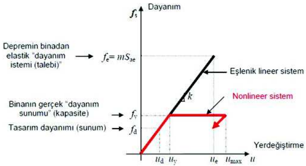
Şekil 2.7. Dayanıma göre tasarımda lineer-nonlinear sistem (Aydınöğlu, 2008).
