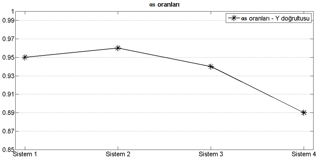
Şekil 5.28. 8 katlı sistemlerin Y yönündeki \alpha_s değerleri
