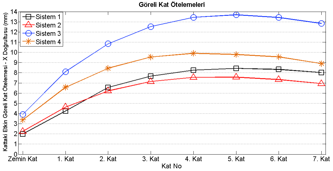
Şekil 5.31. 8 katlı sistemlerin X doğrultusundaki görel kat ötelemeleri
