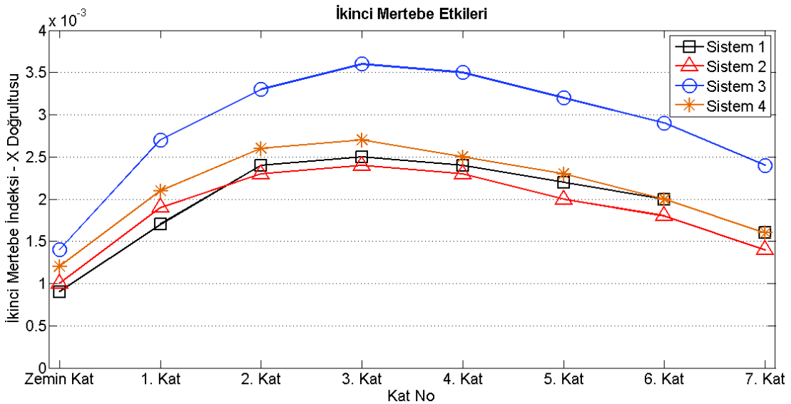
Şekil 5.33. 8 katlı sistemlerin X doğrultusundaki ikinci mertebe etkileri
