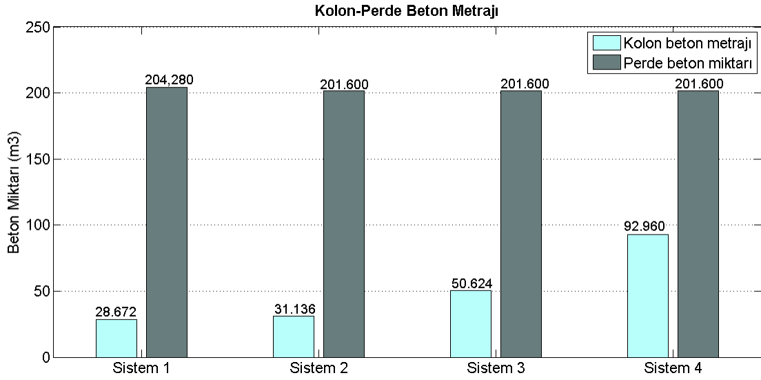
Şekil 5.16. Sistemlerin kolon-pere beton metrajlarının karşılaştırılması
