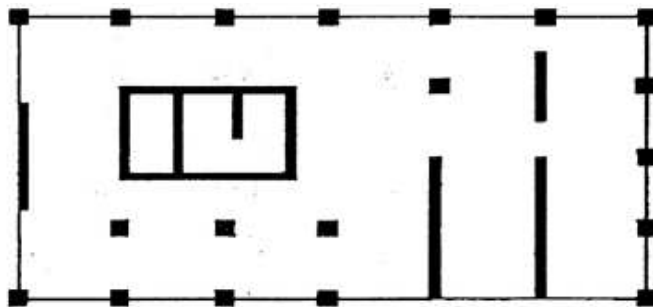
Şekil 2.5. Çekirdek sistem örneği (Özlü, 2015).
