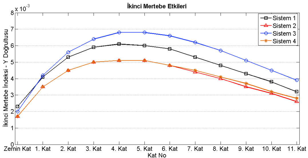
Şekil 5.55. 12 katlı sistemlerin Y doğrultusundaki ikinci mertebe etkileri
