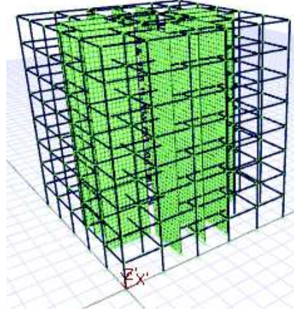
Şekil 4.34. Sistem 4 3B çubuk model.
