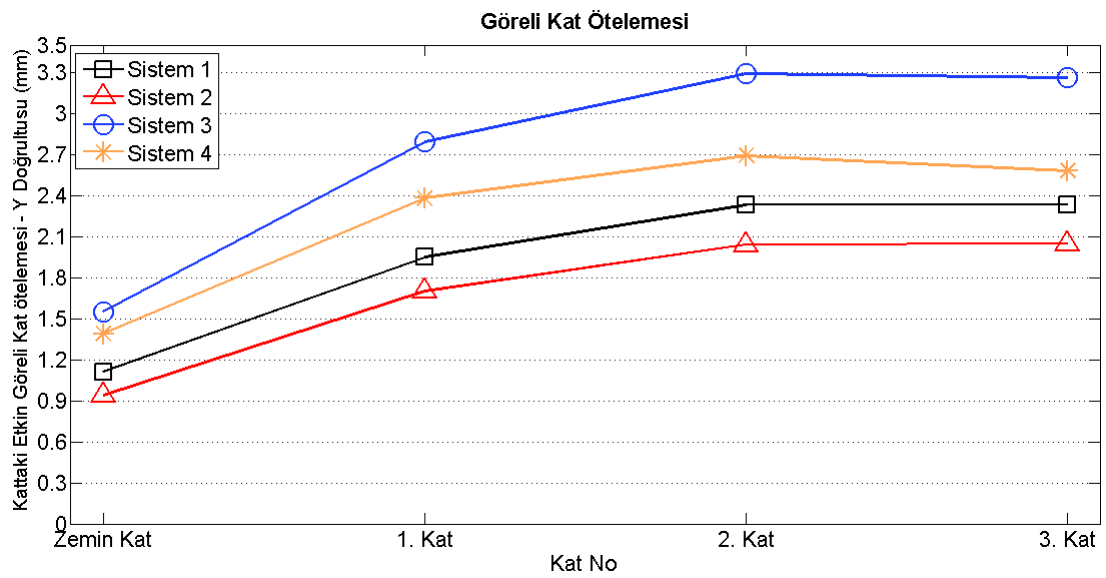
Şekil 5.10. 4 katlı sistemlerin Y doğrultusundaki görel kat ötelemeleri
