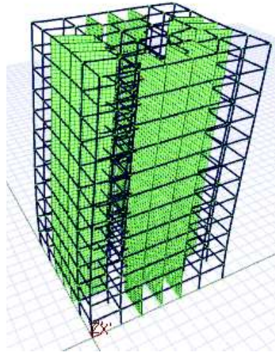
Şekil 4.48. Sistem 3'ün 2. Mod hali.
