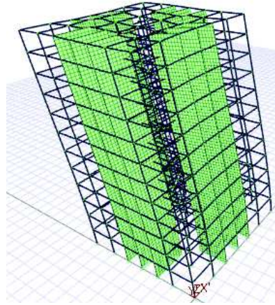
Şekil 4.49. Sistem 3'ün 3. Mod hali.
