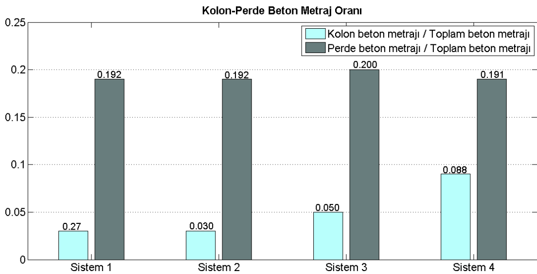
Şekil 5.17. Sistemlerin kolon-pere beton metrajlarının toplam beton metrajına oranlarının karşılaştırılması
