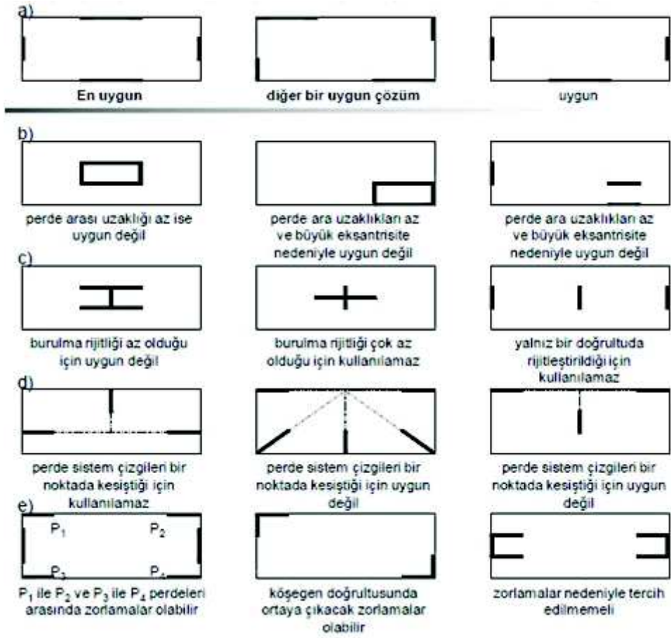
Şekil 2.16. Planda çeşitli perde kullanımı örnekleri (Gülay, 2010).
