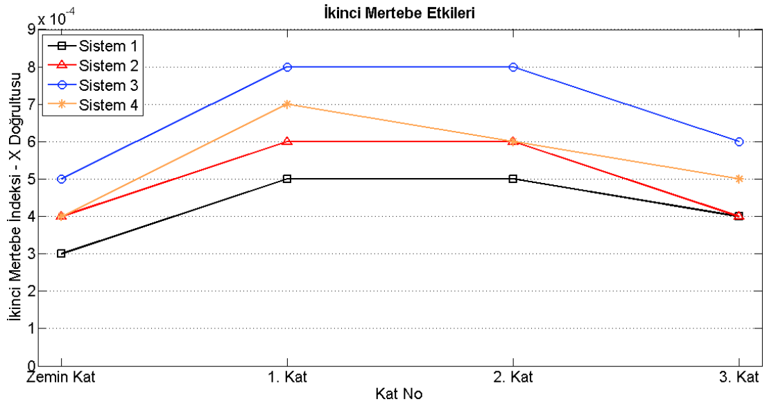
Şekil 5.11. 4 katlı sistemlerin X doğrultusundaki ikinci merteye etkileri
