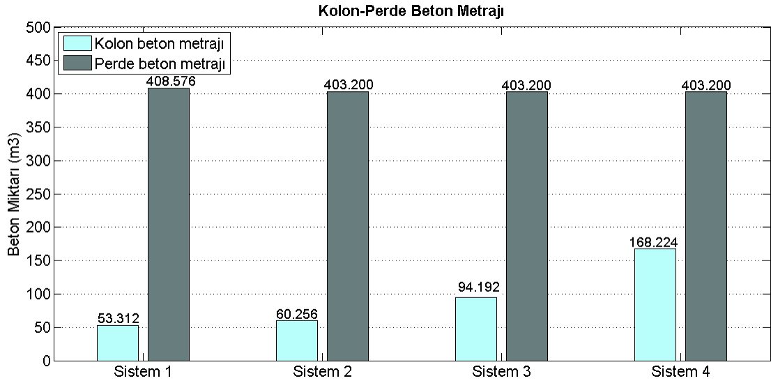
Şekil 5.38. Sistemlerin kolon-pere beton metrajlarının karşılaştırılması
