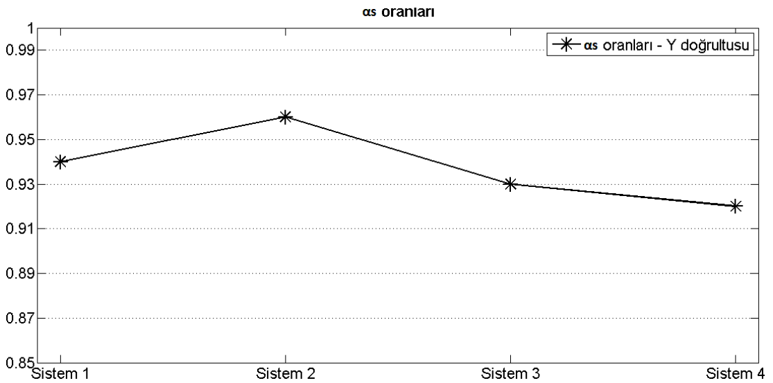
Şekil 5.50. 8 katlı sistemlerin Y yönündeki \alpha_s değerleri
