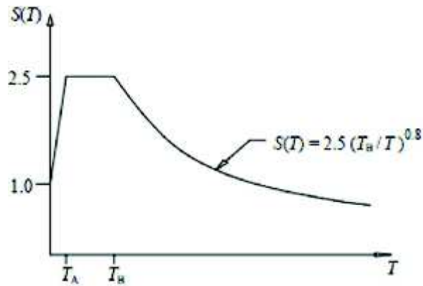
Şekil 3.2. Periyot-Spektrum katsayısı grafiği (Özlü, 2015).
