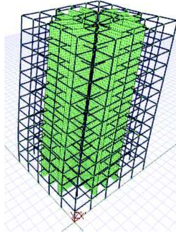
Şekil 4.52. Sistem 4'ün 2. Mod hali.
