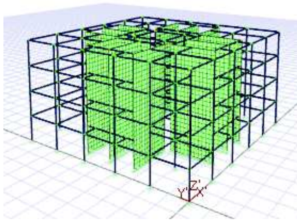
Şekil 4.18. Sistem 4 3B çubuk model.
