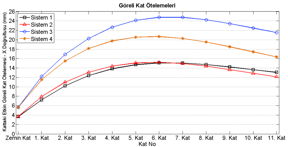
Şekil 5.52. 12 katlı sistemlerin X doğrultusundaki görel kat ötelemeleri
