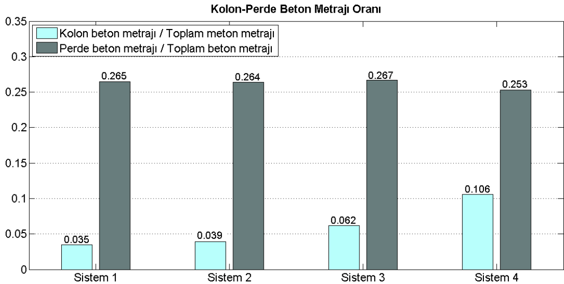
Şekil 5.39. Sistemlerin kolon-pere beton metrajlarının toplam beton metrajına oranlarının karşılaştırılması
