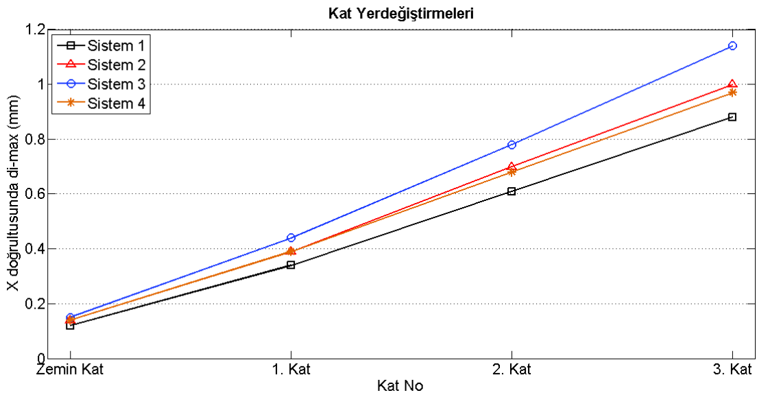
Şekil 5.7. 4 katlı sistemlerin X yönündeki yer değiştirmeleri
