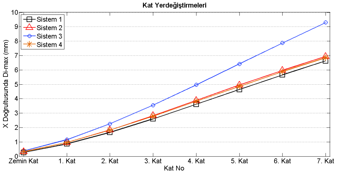
Şekil 5.29. 8 katlı sistemlerin X doğrultusundaki yer değiştirmeleri
