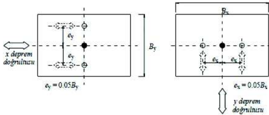
Şekil 3.1. Kütte merkezinin yeri ve kaydırılmış kütte merkezinin konumları (Özlü,2015).
