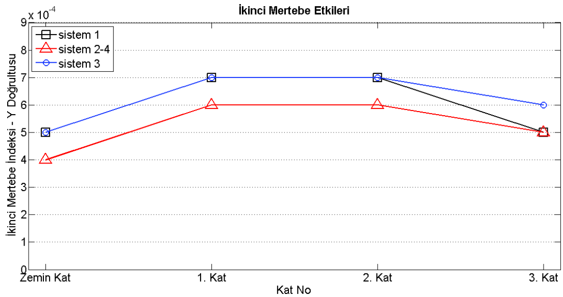
Şekil 5.12. 4 katlı sistemlerin Y doğrultusundaki ikinci merteye etkileri
