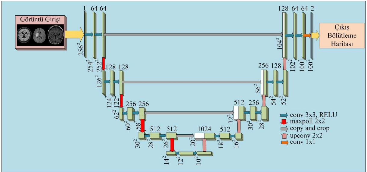
Şekil 4.10. U-Net mimarisi
