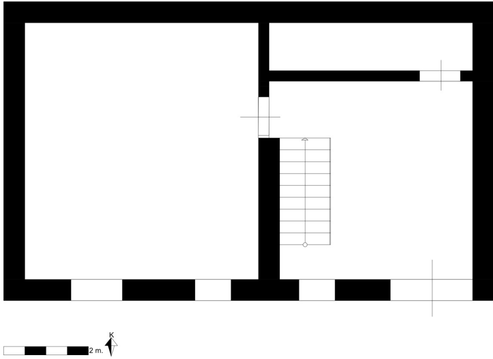
Çizim 2.18. İmamların Odası Alt Kat Planı
