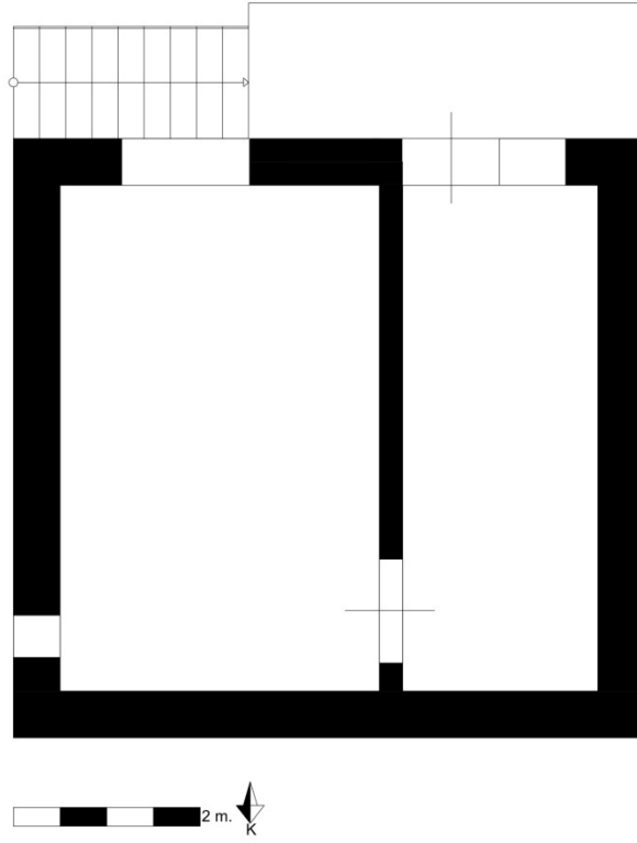
Çizim 2.26. Issıları / Hatıpların Odası Üst Kat Planı
