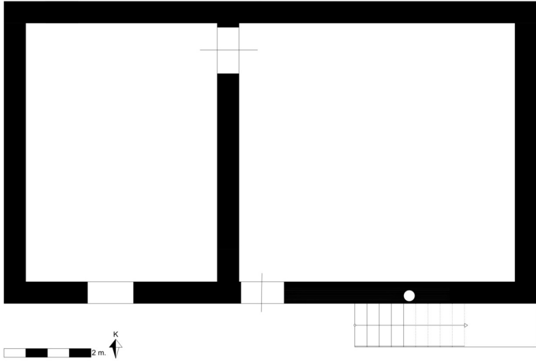
Çizim 2.6. Kayışoğlu Odası Alt Kat Planı
