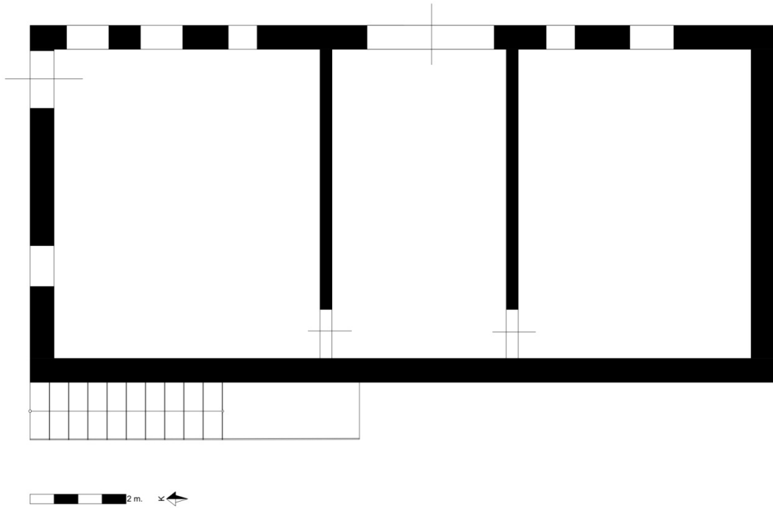
Çizim 2.16. Gökçimen Meydan Konağı / Odası Alt Kat Planı
