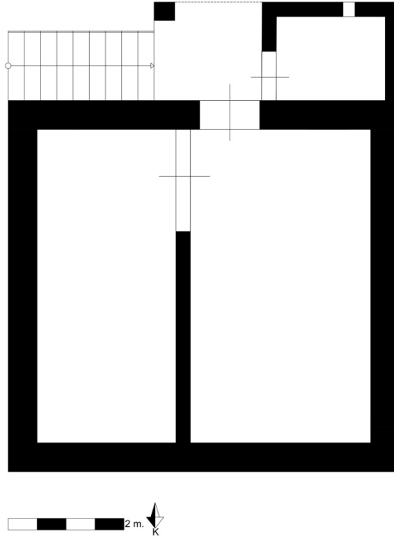
Çizim 2.27. Issıların / Hatıpların Odası Alt Kat Planı
