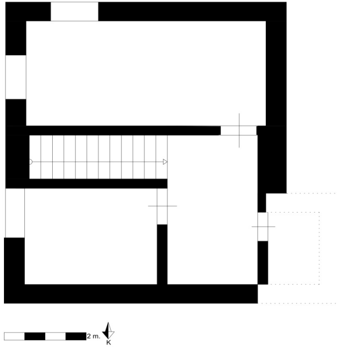
Çizim 2.37. Ömer Çavuş Odası Üst Kat Planı
