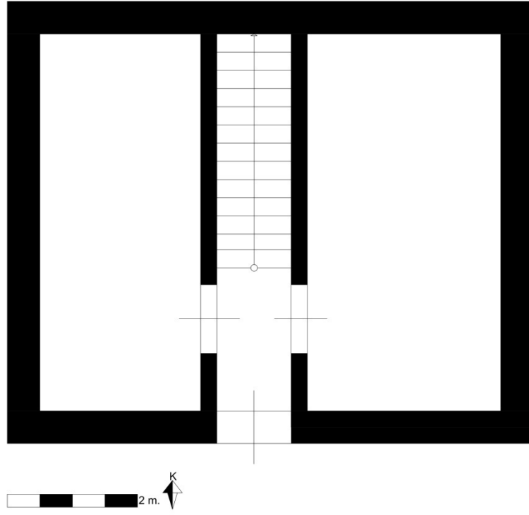
Çizim 2.38. Karaböcüler Odası Alt Kat Planı
