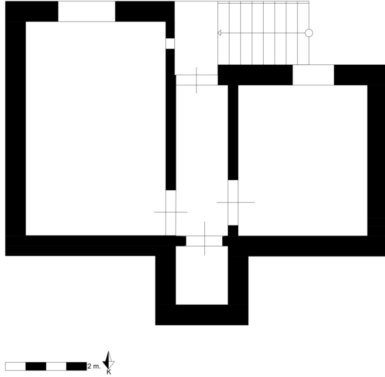
Çizim 2.35. Kel İbrahim Odası Kat Planı
