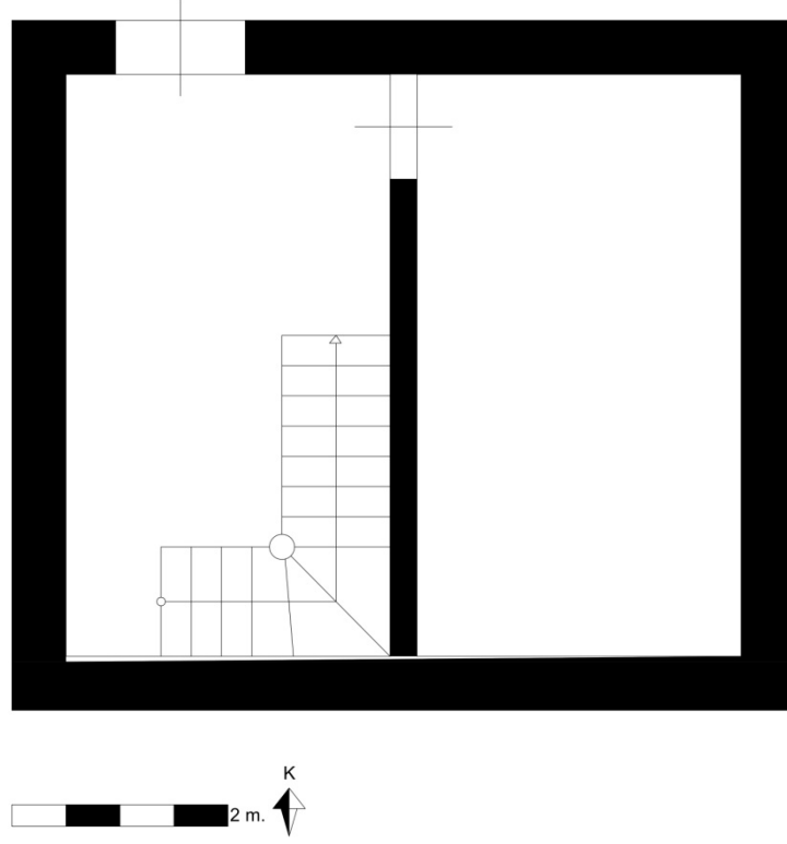
Çizim 2.30. Karaböceklerin Odası Alt Kat Planı
