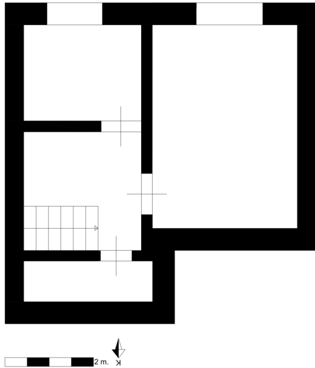
Çizim 2.28. Kavaslari Odası Alt Kat Planı
