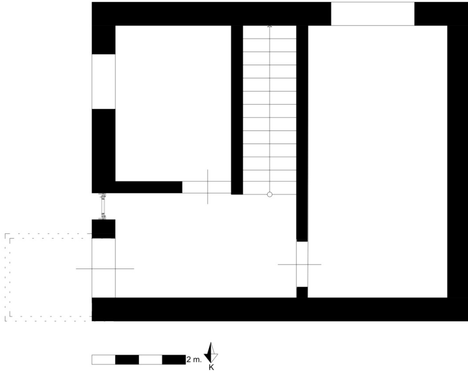
Çizim 2.39. Karaböcüler Odası Üst Kat Planı
