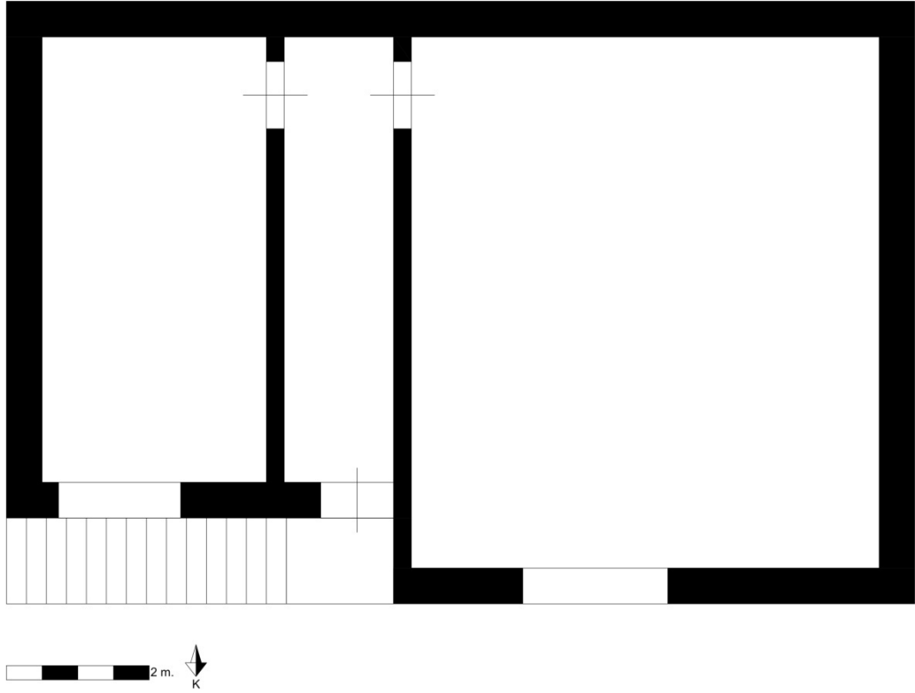
Çizim 2.23. Tellinin Odası Üst Kat Planı
