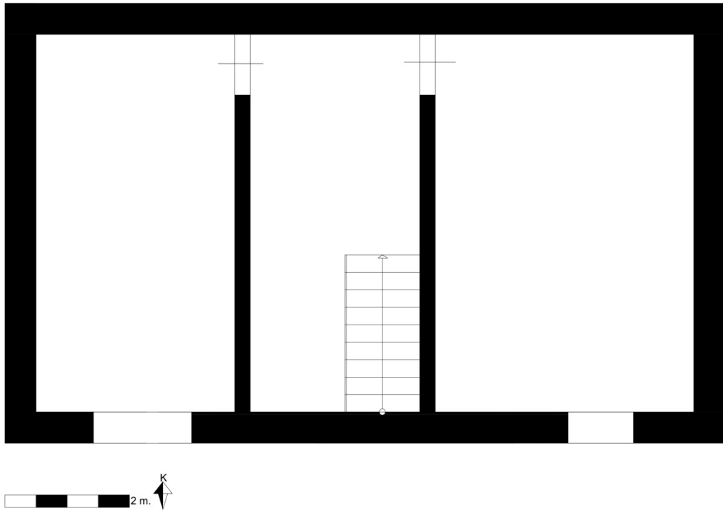
Çizim 2.19. İmamların Odası Üst Kat Planı
