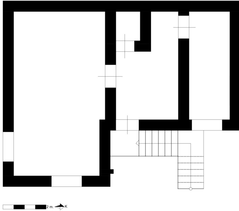
Çizim 2.5. Efendi Odası Üst Kat Planı
