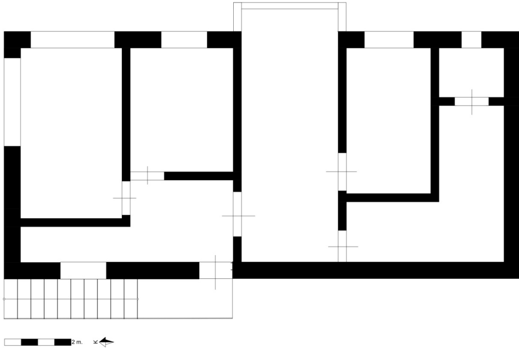
Çizim 2.15. Gökçimen Meydan Konağı / Odası Üst Kat Planı
