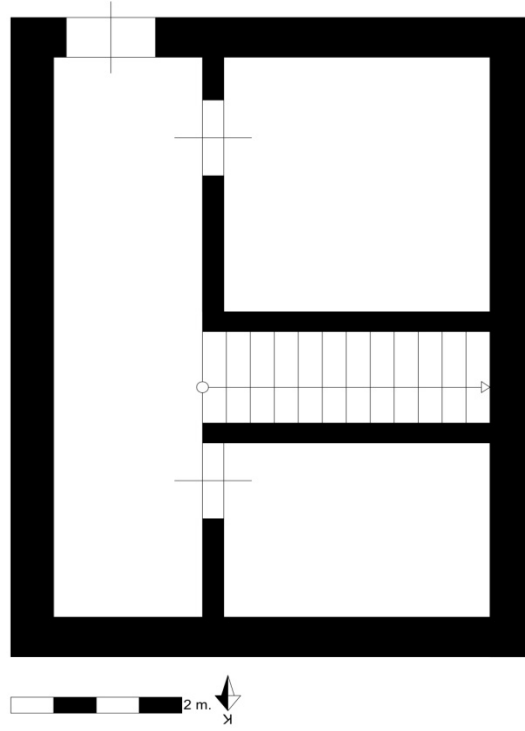
Çizim 2.36. Ömer Çavuş Odası Alt Kat Planı
