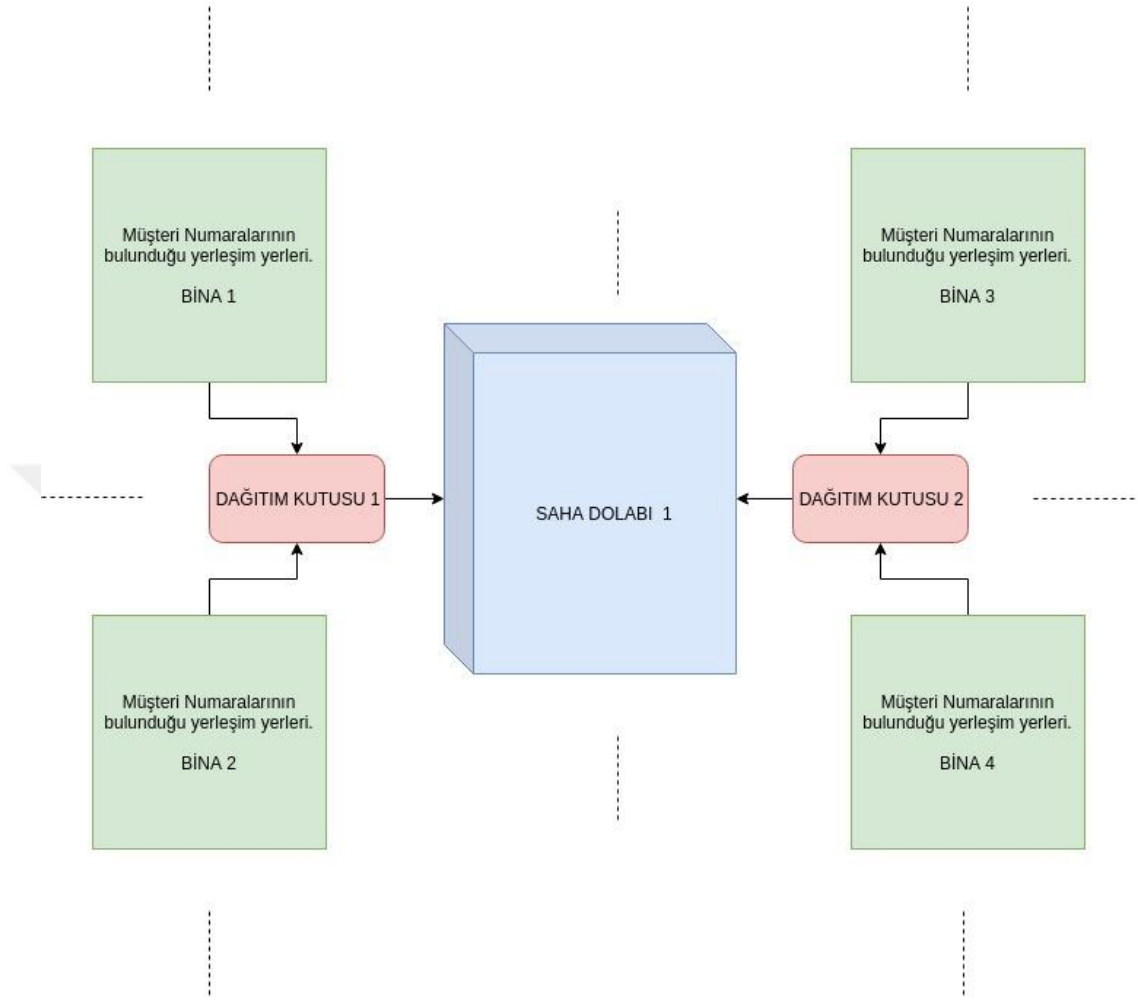
Şekil 3.1. Lokasyon Tipleri
