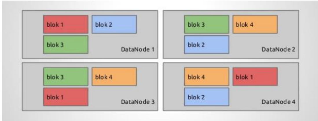
Şekil 2.1. HDFS Blokları
