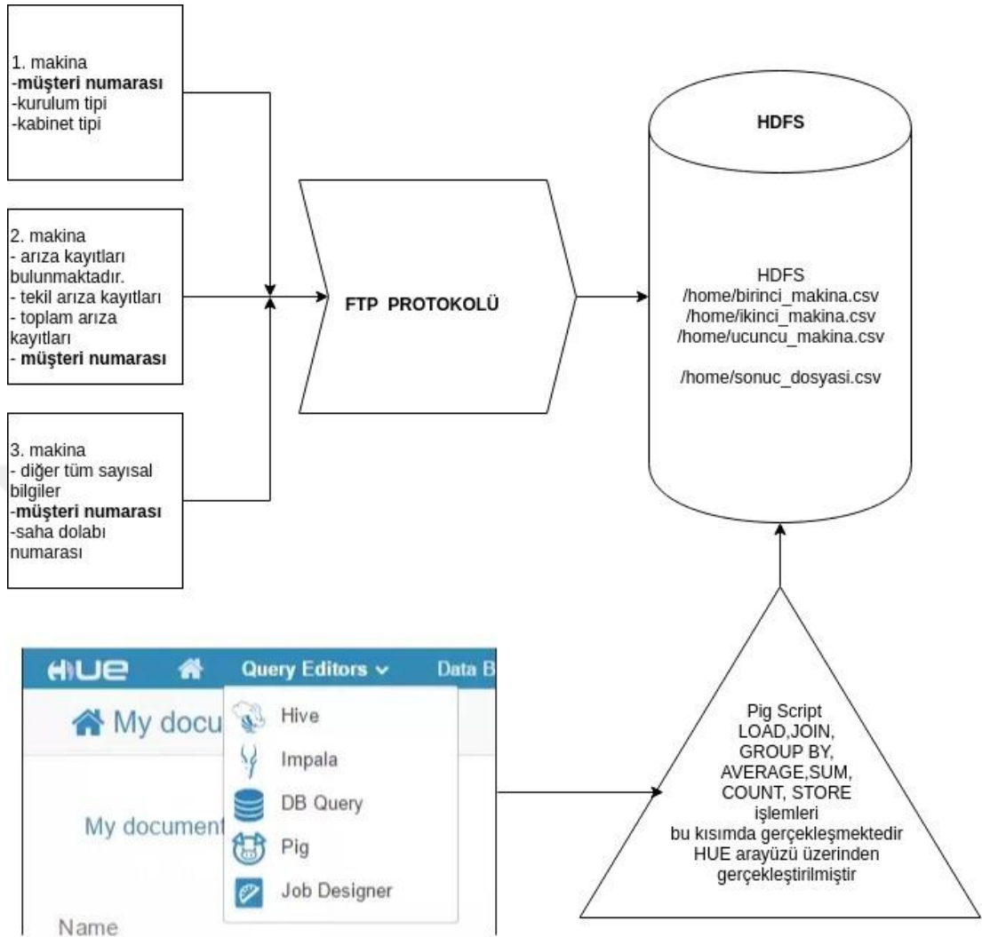
Şekil 3.2. İşlemler Diyagramı
