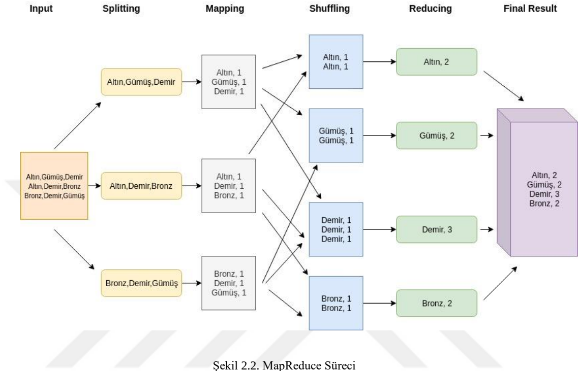
Şekil 2.2. MapReduce Süreci
