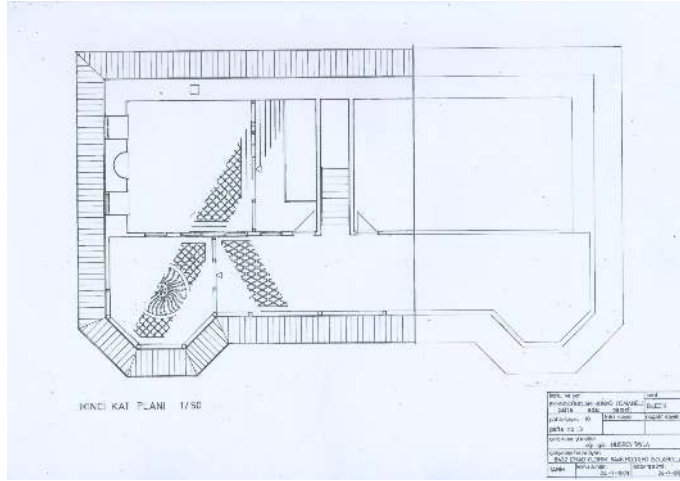
Şekil 5.5 Harem kısmı ikinci kat planı(M.S.Ü. Restorasyon Anabilim Dalı Arşivi).
