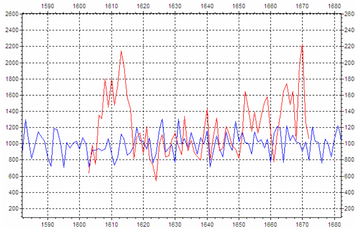
Çizelge 5.1 Osmaneli civarına en yakın karaçam ana kronoloji (Bolu) ve Tokluoğulları Konağından alınan örneğin karşılaştırması. Son yıl 1672; iki grafik arasındaki uyum yüzdesi %66, t=3.63 ve D=57.92 dir. Grafikte, x eksenı yıllar; y eksenı halka indisleridir.
