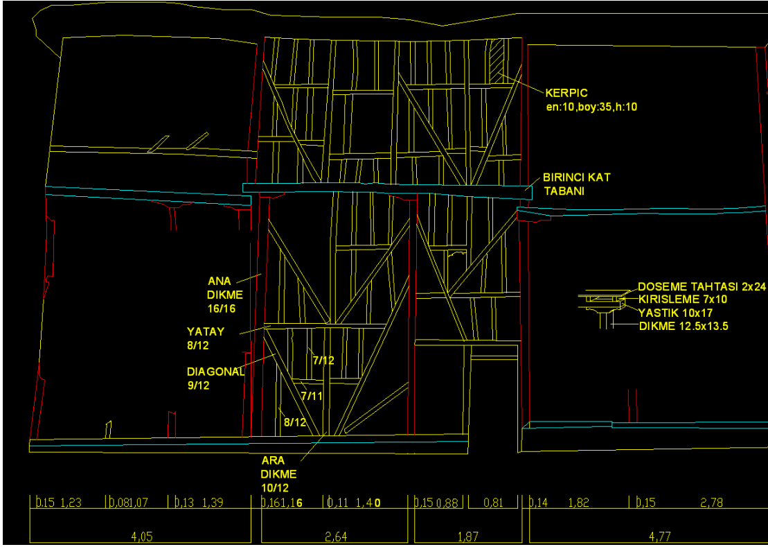
Şekil 4.16 Genel sistem ölçülerinin, arka cephe bölgesinde incelenmesi
