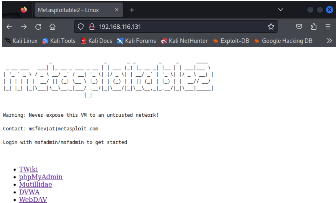
Şekil.10.43.Metasploitable2 Ara Yüzü
