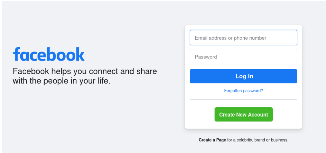
Şekil 10.58.Facebook Giriş Ekranı
