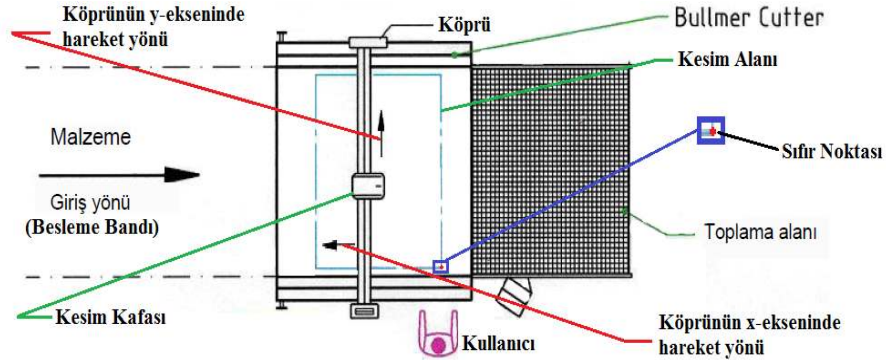
Şekil 3.192 Cutter masası hareket yönleri
