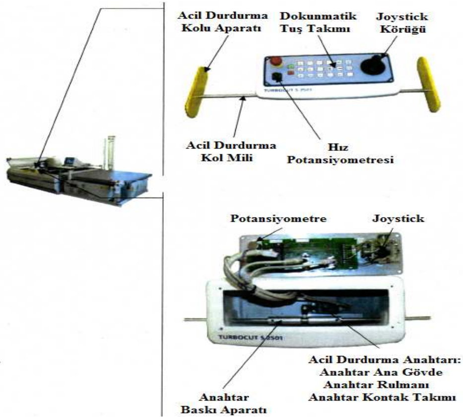
Şekil 3.39 Kontrol panelinin alt bileşenleri (Assyst Bullmer, 2001, düzenleme:M.S.Ç.)
