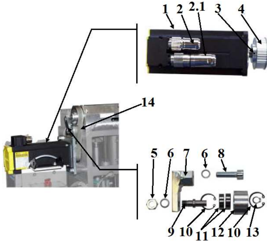
Şekil 3.15 Kayış tahriki – bıçak (önden görünüşte) bileşenleri 1: Servo motor, 2: Servo motor power fişi, 2.1: Servo motor enkoder fişi, 3:Setsukur, 4: Triger dişli, 5: Somun, 6: Rondela, 7: Kafa arka kayış gerdirme aparatı tutucusu, 8: Vida, 9: Arka kayış gerdirme teker mili, 10: Segman, 11: Rondela, 12: Teker, 13: Segman, 14: Triger dişli kayışı (Assyst Bullmer, 2001, düzenleme:M.S.Ç.)
