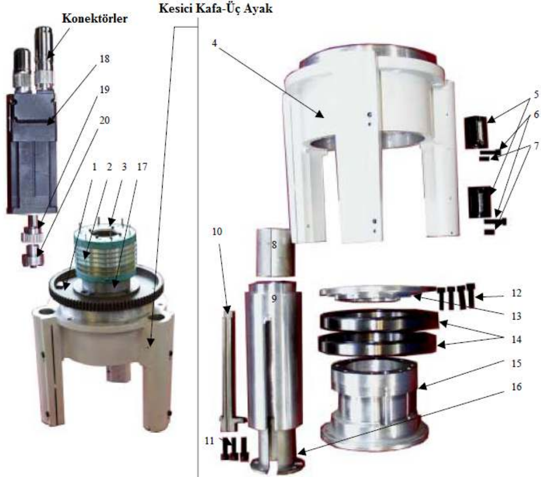
Şekil 3.24 Üç ayak bileşenleri 1: c eksen dişlisi, 2: Akıllı bıçak modülü, 3, 6, 11, 12: Vida, 4: c eksen ana gövdesi, 5: sıralı bilya, 7: Setsukur, 8: Sıralı rulman, 9: Bıçak sürücüsü kılavuz aparatı, 10: Metal kızak, 13: c eksen üst kapak, 14: c eksen üst rulmanı, 15: c eksen rulmanı tutucusu, 16: Bıçak sürücü kılavuz aparatı başlığı, 17: c eksen üst dişlisi, 18: c eksen motoru, 19: c eksen motoru dişlisi, 20: c eksen motoru dişli tutucu segman (Assyst Bullmer, 2001, düzenleme:M.S.Ç.)
