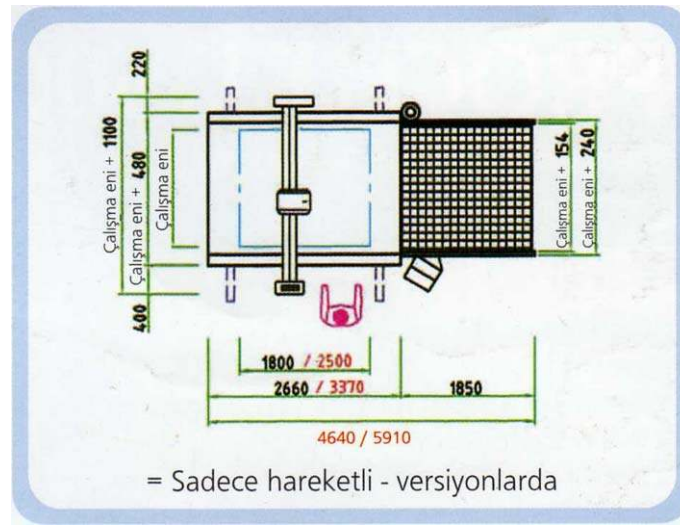
Şekil 2.9 Cutter'ın yerleşim alanı ölçüleri
