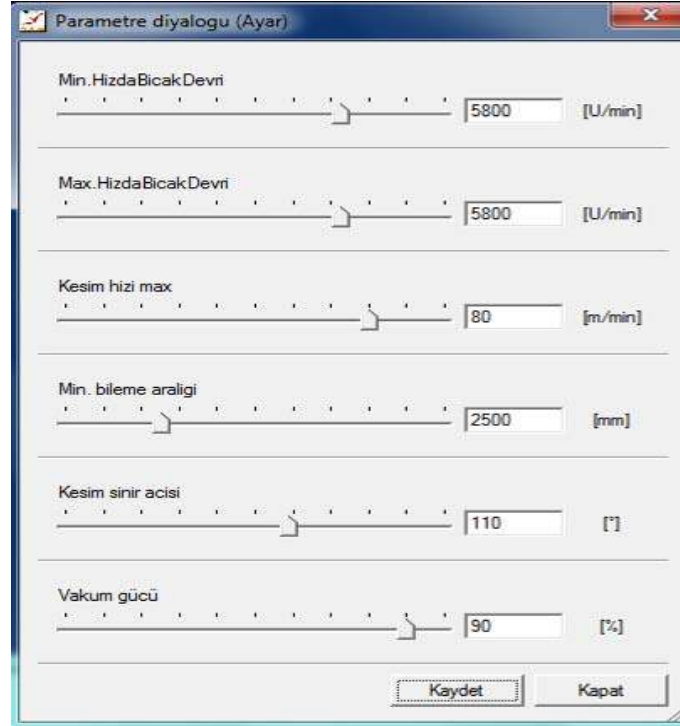
Şekil 3.184 “Parametre diyalogu (Ayar)” penceresi
