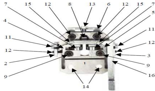
Şekil 3.21 Bıçak kılavuzu bileşenleri 1:Alt bıçak kılavuz aparatı, 2: Sol alt rulman tutucu, 3: Sağ alt rulman tutucu, 4: Sol üst rulman tutucu, 5: Sağ üst rulman tutucu, 6: Sırt rulman tutucu, 7: Bıçak yan rulmanı ile setsukur, 8: Bıçak arka rulmanı ile setsukur, 9, 12, 15: Silindir vida, 10:Setsukur, 11, 13: Altı köşe başlı vida, 14: Vida yatağı, 16: akıllı bıçak hissetme aparatı (Assyst Bullmer, 2001, düzenleme:M.S.Ç.)
