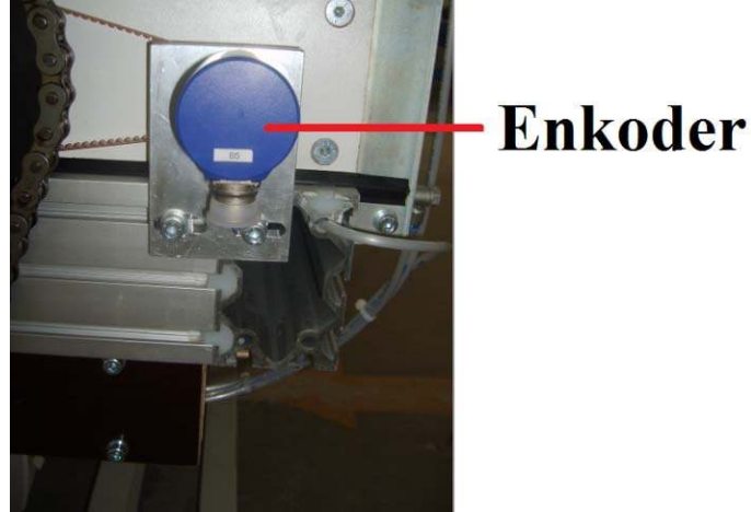
Şekil 3.52 Enkoder (Çekim ve düzenleme: M.S.Ç.)
