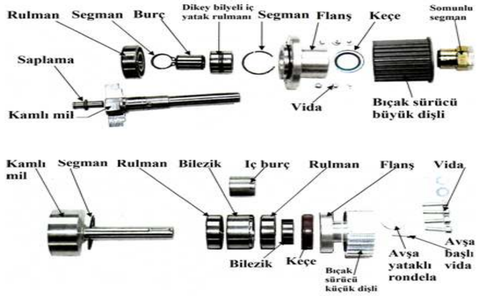
Şekil 3.21 Bıçak tahrik mekanizması kütle balans milleri (Assyst Bullmer, 2001, düzenleme: M.S.Ç.)
