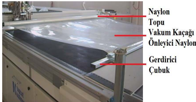
Şekil 3.82 Naylon topu taşıma ve sarma aparatı 2 (Çekim ve düzenleme: M.S.Ç.)
