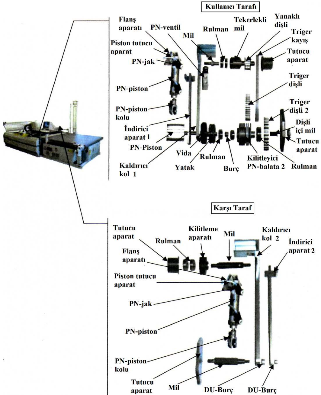
Şekil 3.38 Naylon topu taşıma ve sarma aparatı 2 (Assyst Bullmer, 2001, düzenleme:M.S.Ç.)
