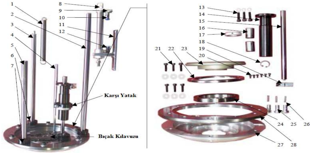
Şekil 3.25 Döner tabla alt aparatı (Çanak) bileşenleri) 1: Yay, 2, 3, 4, 5, 15: Mil, 6: Plastik şok önleyici takoz, 7: Plastik şok önleyici lastik, 8: Piston, 9: PN-jak tansiyonu, 10, 12: PN-jak, 11: Piston tutucu aparat, 13, 20, 21: Vida, 14: c eksenli hareket mili, 16: Sıralı bilya, 17: Bilezik, 18: Segman, 19: Mil sıkıştırma aparatı, 22: c eksenli alt bileziği, 23: c eksenli, 24: c eksenli iç rulmanı, 25: içten geçmeli sıkma vida, 26: Sıkma vida aparatı, 27: çanak ana gövde, 28: çanak ana gövde üst bileziği (Assyst Bullmer, 2001, düzenleme:M.S.Ç.)
