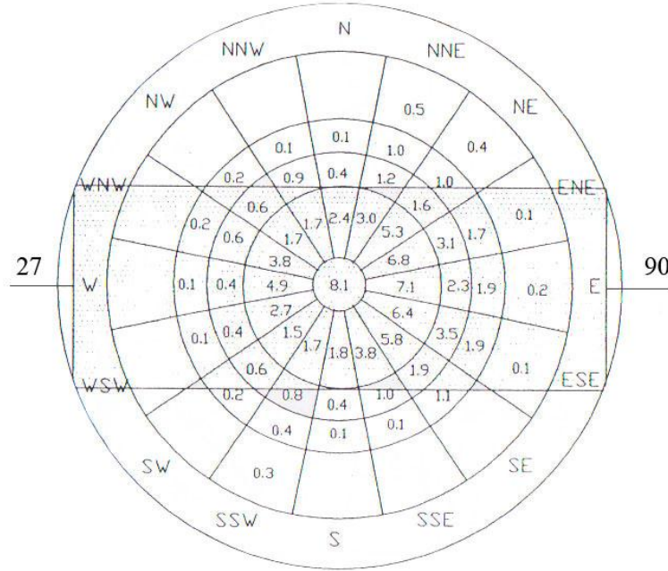
Şekil 3.9. Birinci pist için uygun yönün bulunması [20].
