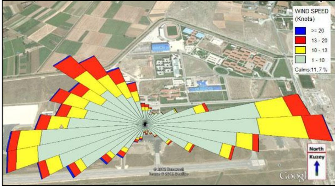
Şekil 5.5. WRPLOT View 7.0 programı yardımıyla rüzgâr verilerinin incelenmesi.
