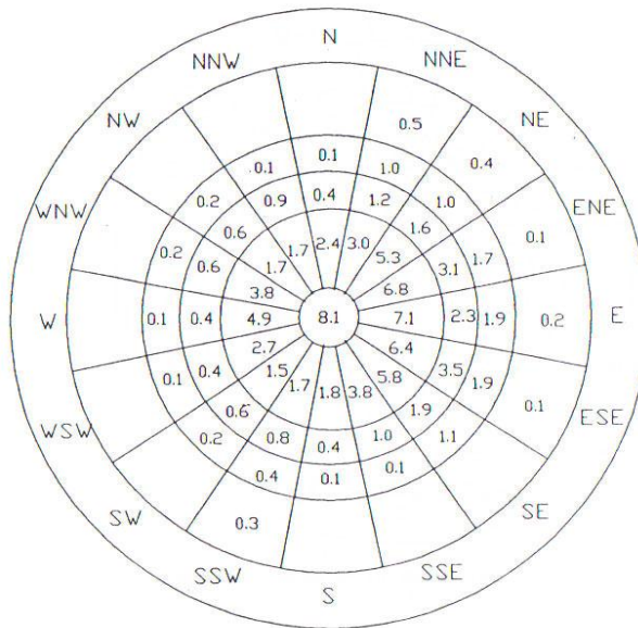
Şekil 3.8. Örnek uygulamaya ait rüzgârgülü [20].
