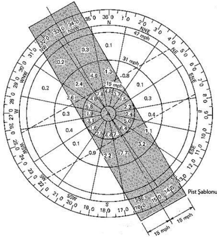
Şekil 3.6. İkinci ve birinci piste ait şablon yerleşimleri [24].
