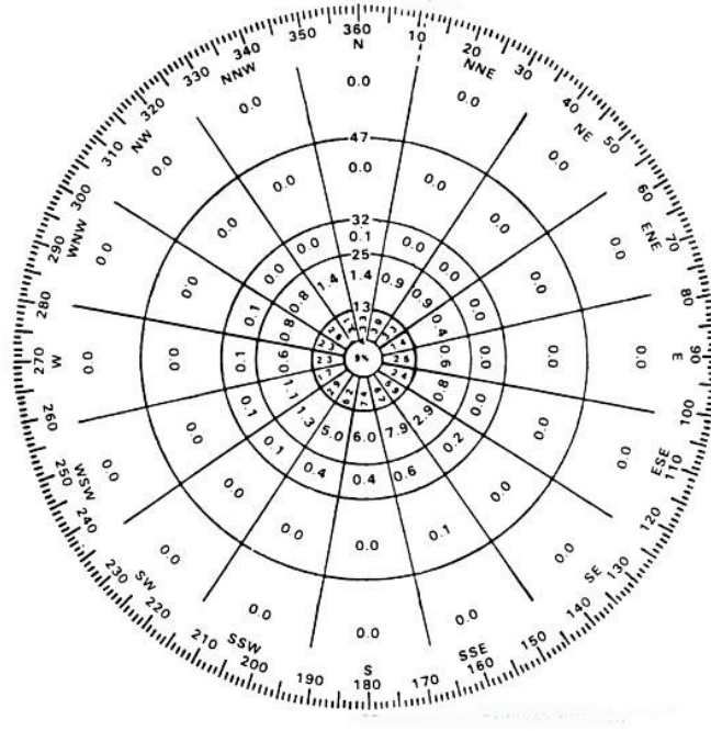
Şekil 3.3. Rüzgârgülü grafiğinin veri işlenmiş hali [22].
