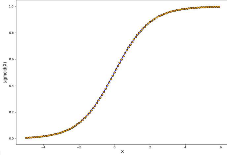
Şekil 3.8. Lojistik Regresyon [65].
