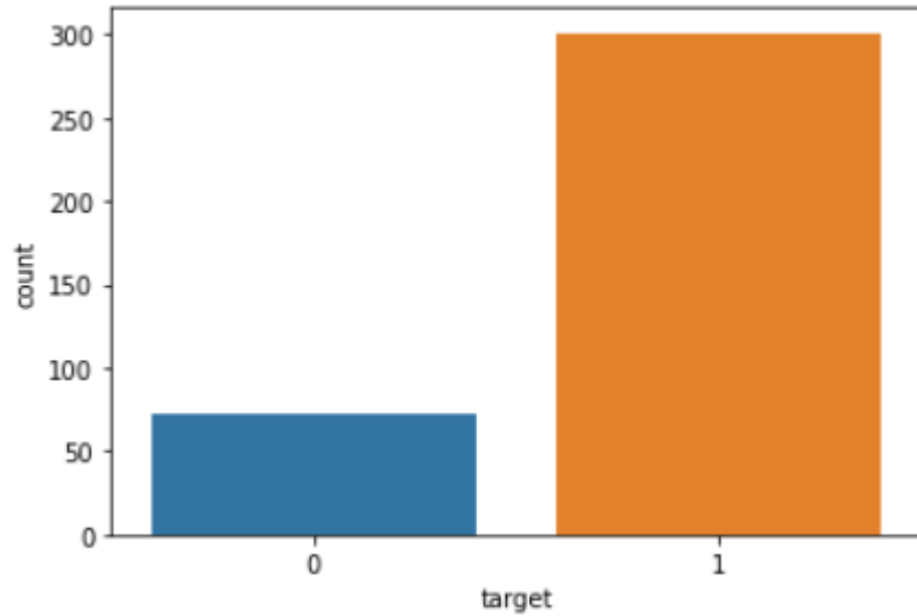
Şekil 4.3. Kategoriler.
