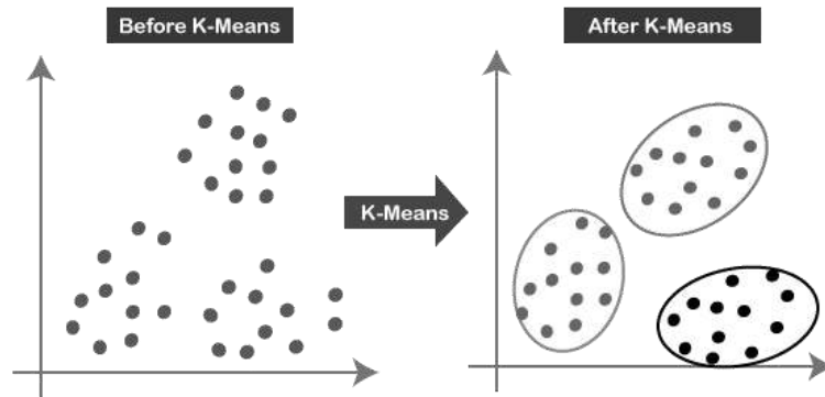
Şekil 3.6. K-Ortalamlar Algoritması [61].
