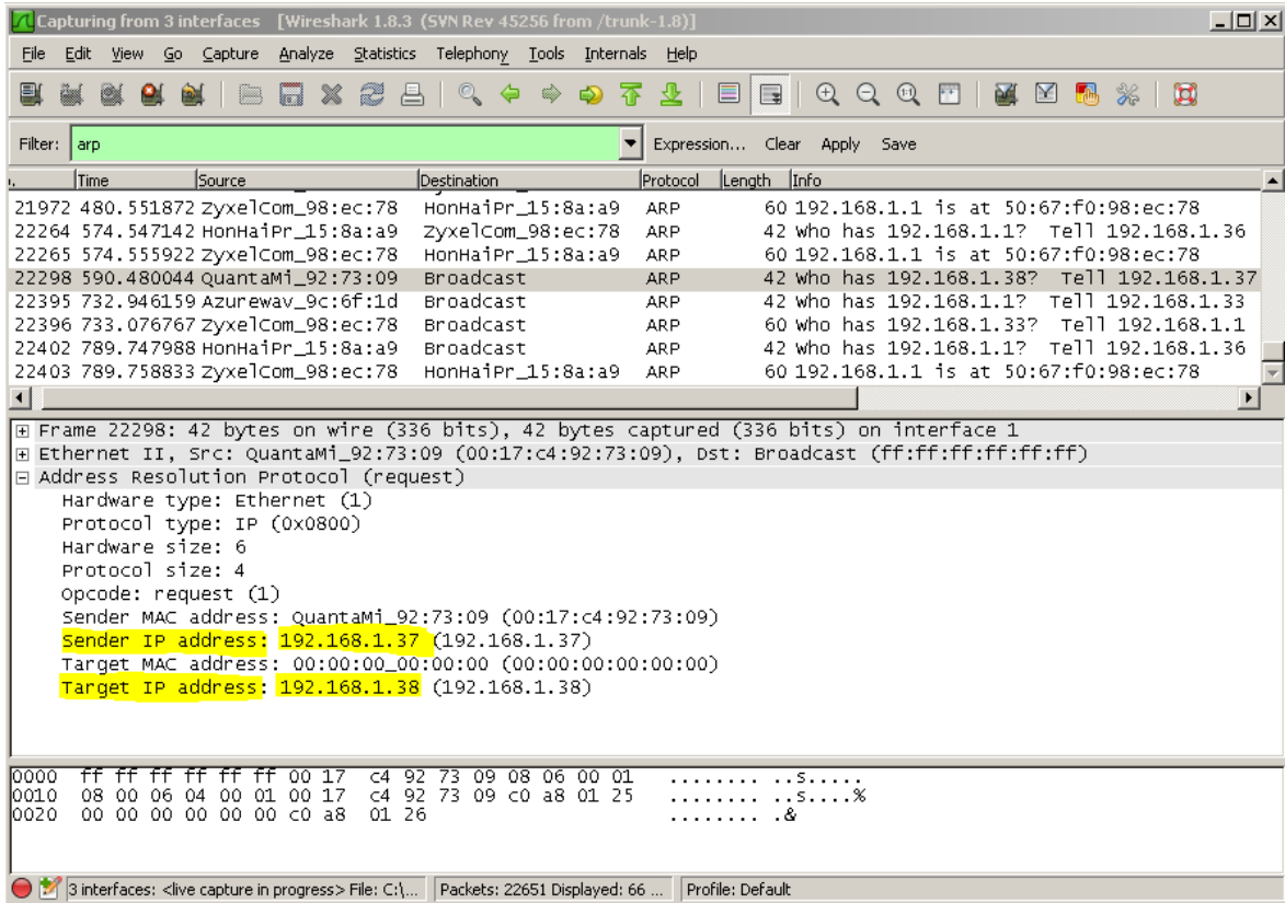
Şekil 25. Wireshark ile saldırıyanın IP adresinin tespit edilmesi
