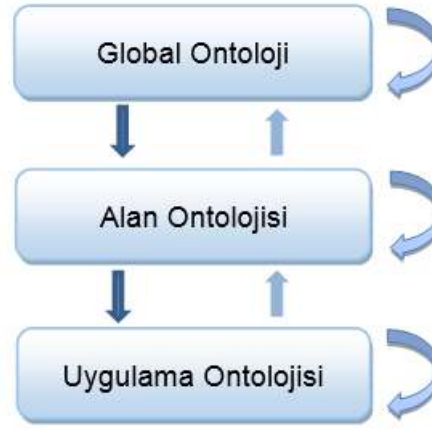
Şekil 4.1 Ontoloji Türleri
