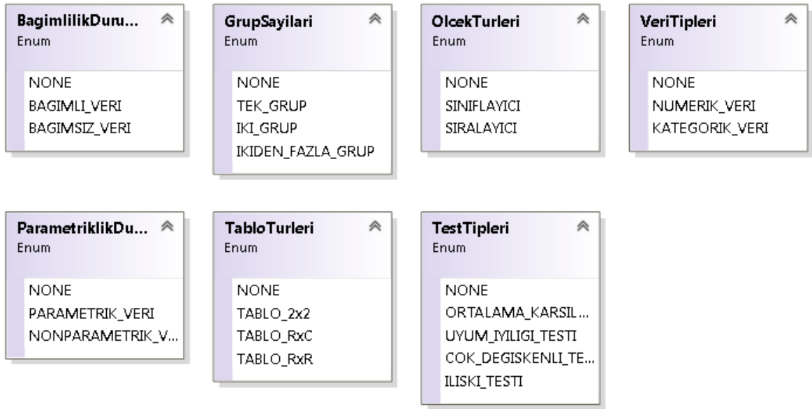
Şekil 5.11 Özellikler Listesi
