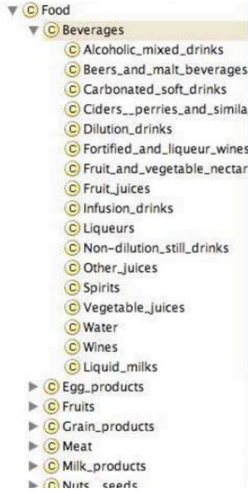
Şekil 4.16 Yemek Ontolojisi
