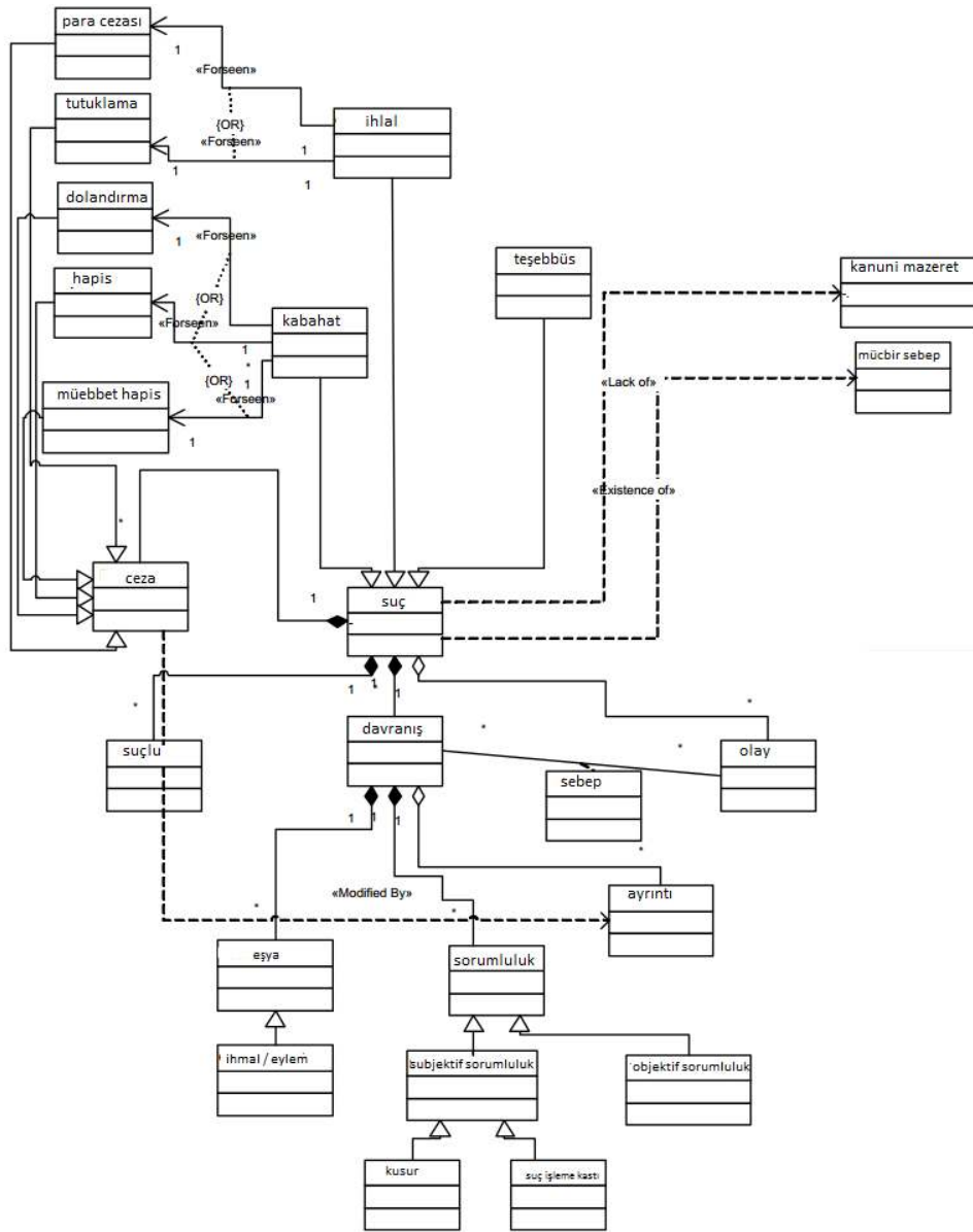
Şekil 4.15 Suç Ontolojisi
