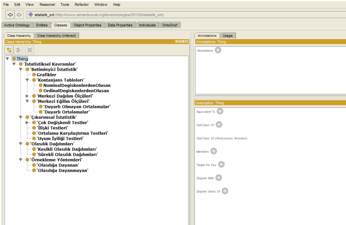
Şekil 5.2 Oluşturulan Sınıflar
