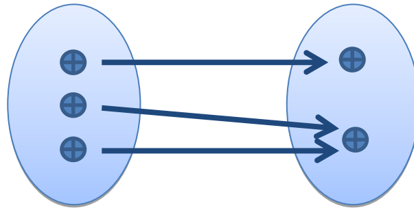
Şekil 4.5 Fonksiyonel Özellik
