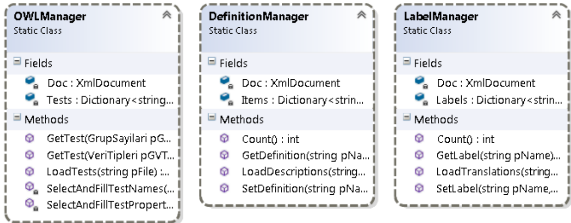
Şekil 5.12 Yönetici Sınıflar
