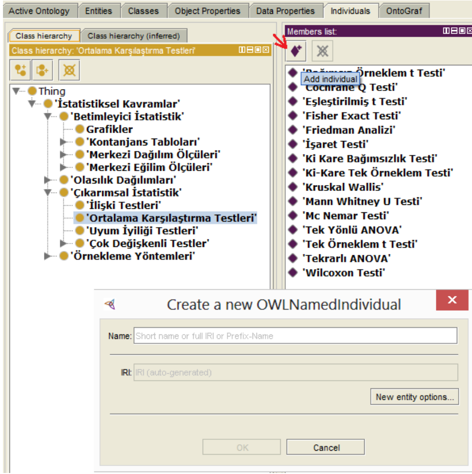
Şekil 5.22 Birey Ekleme
