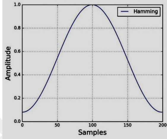
Şekil 2. 9. Hamming Penceresi
