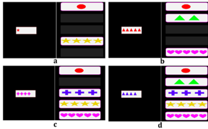
Şekil 2. 4. WKET uygulaması
