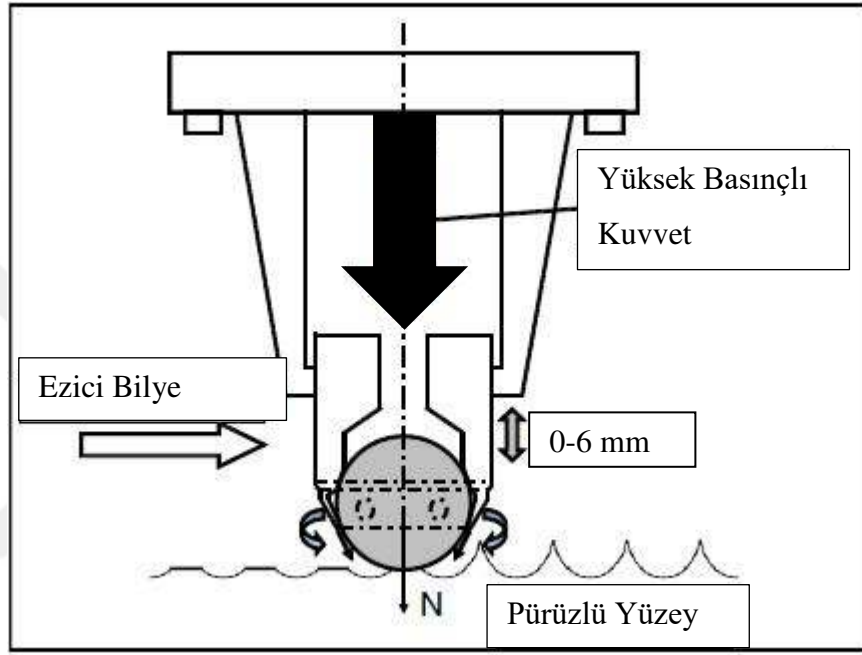
Şekil 4.3 Bilyeli haddelenme işleminde takım ve numunenin hareket şekli [7].
