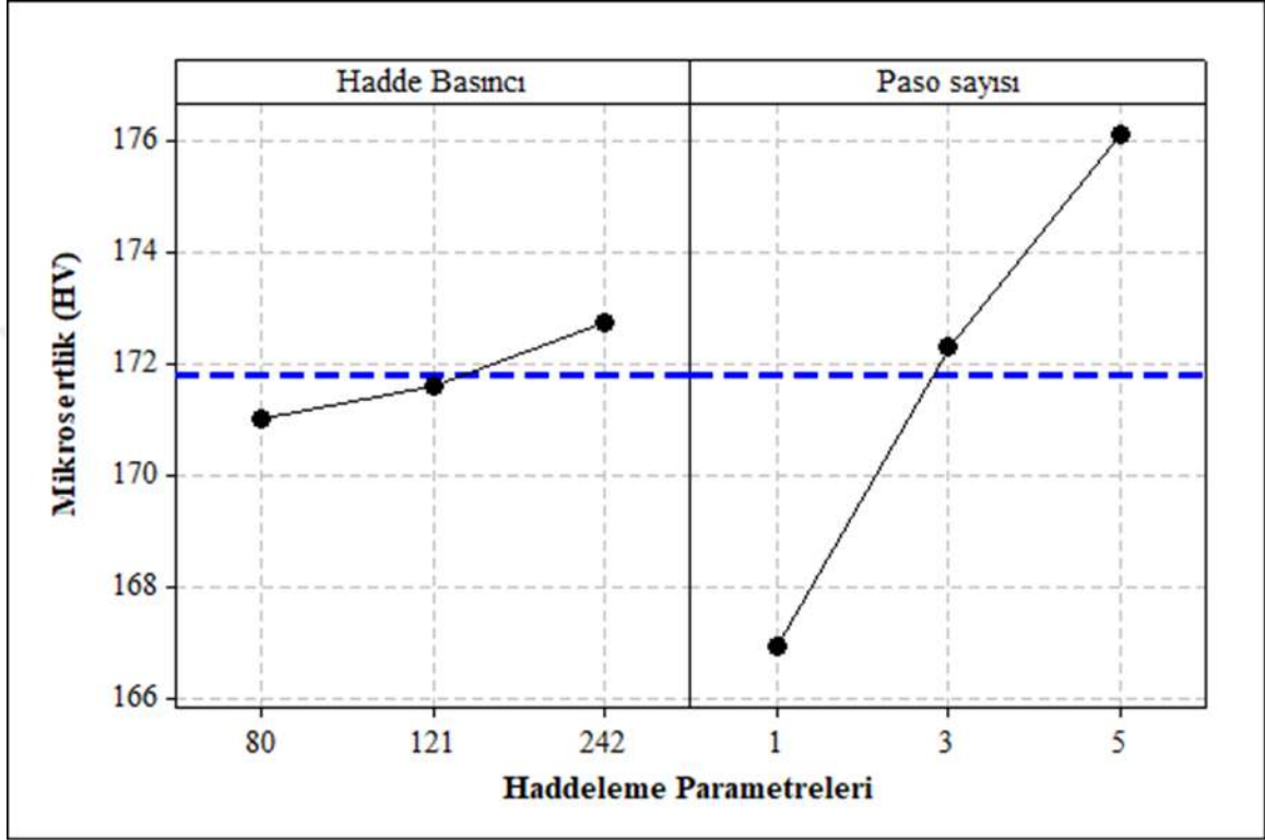
Şekil 6.2 Haddeme parametrelerinin yüzey sertliği üzerindeki etkileri
