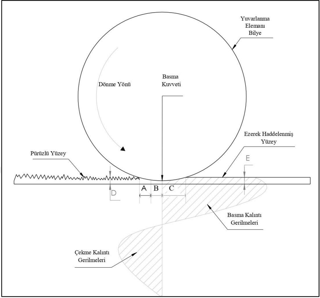
Şekil 4.6 Bilyeli haddelerme işlemi ve malzemede meydana gelen deformasyon [61].
