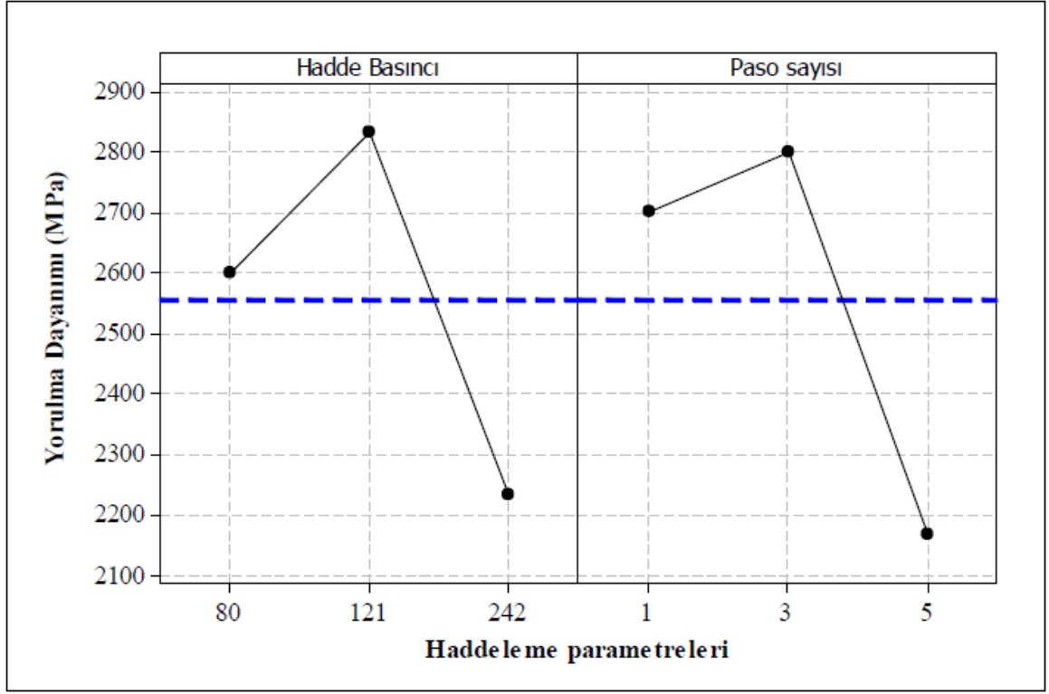
Şekil 6.8 Haddeleme parametrelerinin yorulma ömrü üzerindeki etkileri (Maksimum gerilme)
