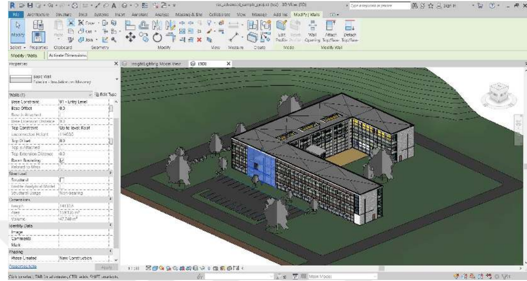
Şekil 3.3. Autodesk Revit 2019 platformunda dış duvar bileşenine ait gösterim
