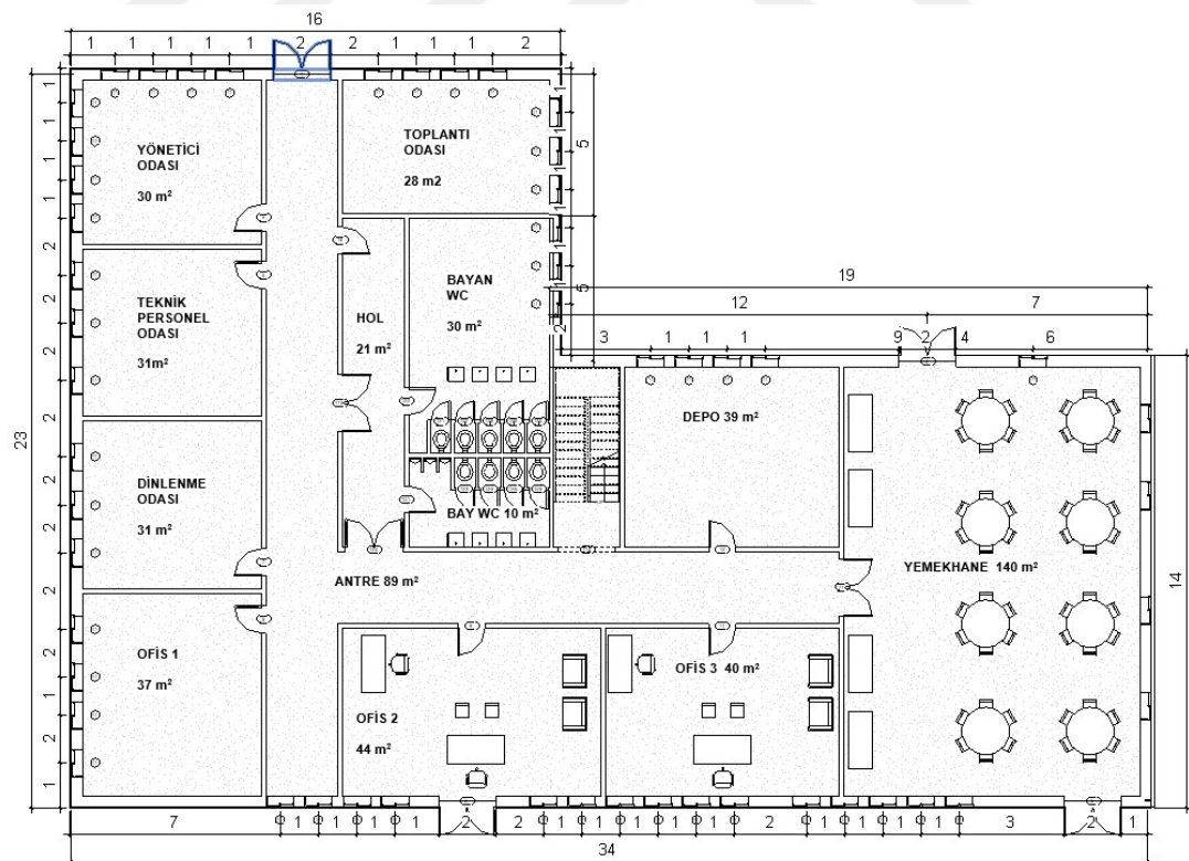
Şekil 4.6. 1.Kat planı
