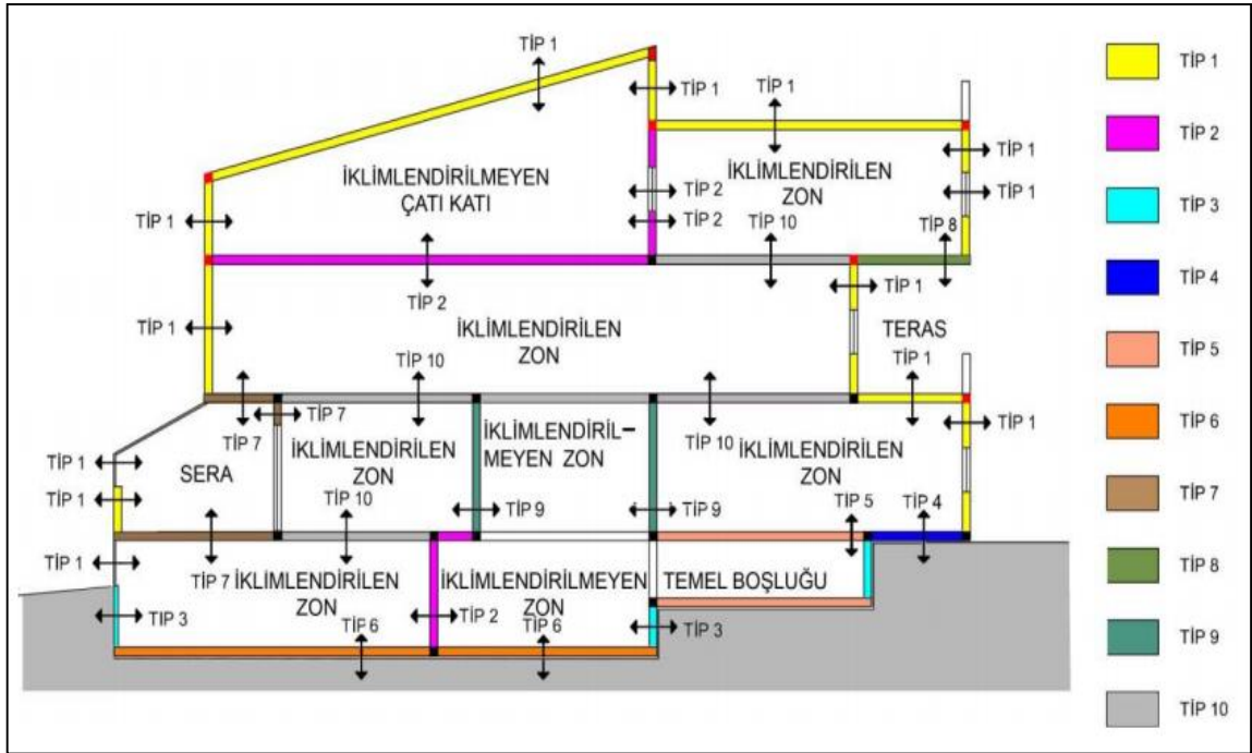
Şekil 25. Isı geçiş hesapları için ısı şartları farklı zonları ayıran yapı bileşenleri
