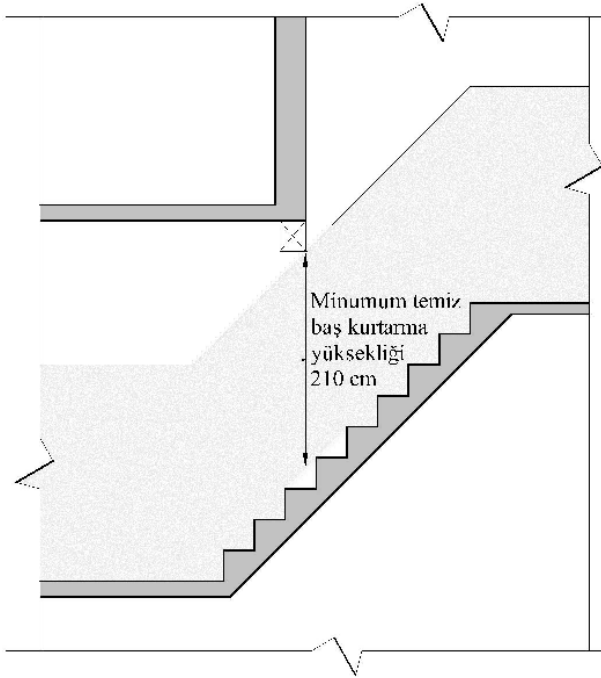
Şekil 5.7. Merdiven yüksekliği [80]
