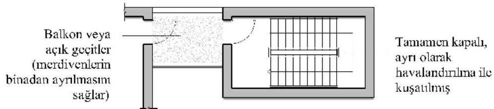
Şekil 5.19. Binadan ayrılmış kaçış merdiveni [15]
