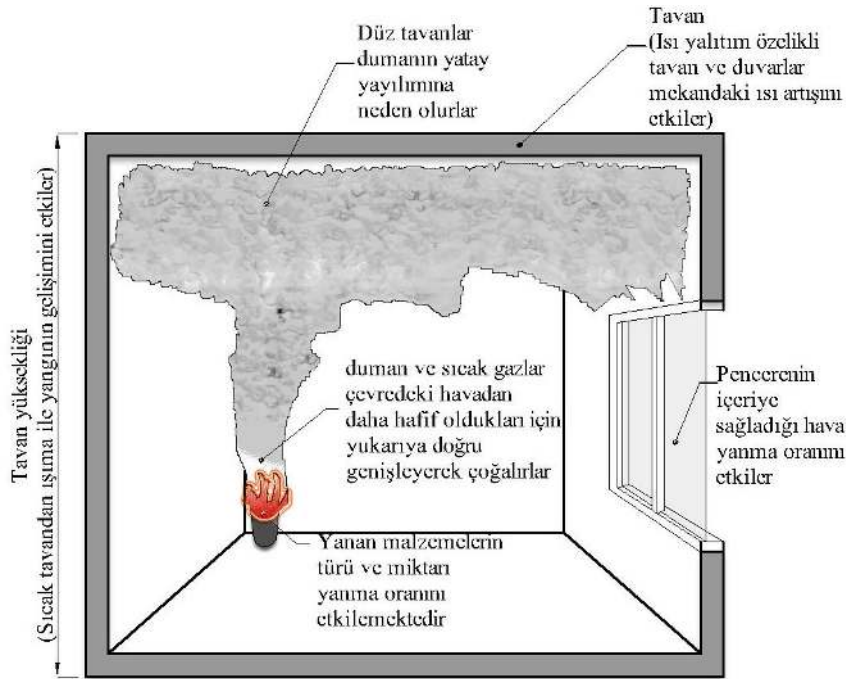
Şekil 2.4. Sınırlı alanlarda yanma davranışı [15]
