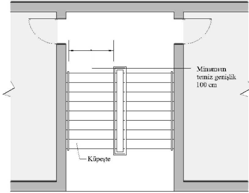
Şekil 5.6. Merdiven genişliği [80]
