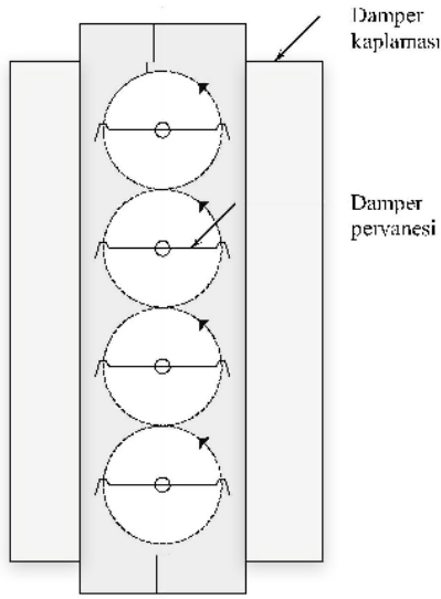
Şekil 4.16. Çok sayıda pervane ile düzenlenmiş yangın ve duman damperi (pervanelerin açık olduğu durum) [65]
