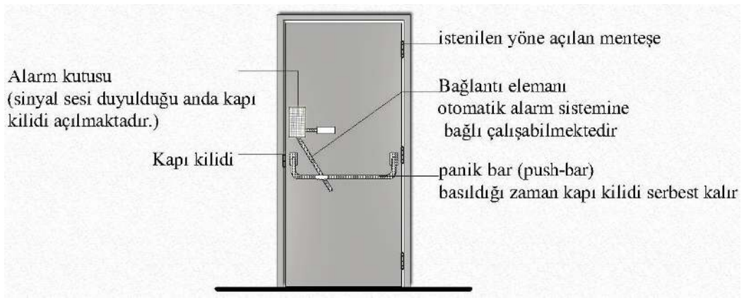
Şekil 5.22. Çıkış kapısı [15]
