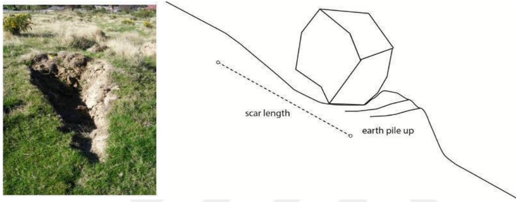
Şekil 3.3. Yumuşak Toprakta Kaya Darbe İzi
