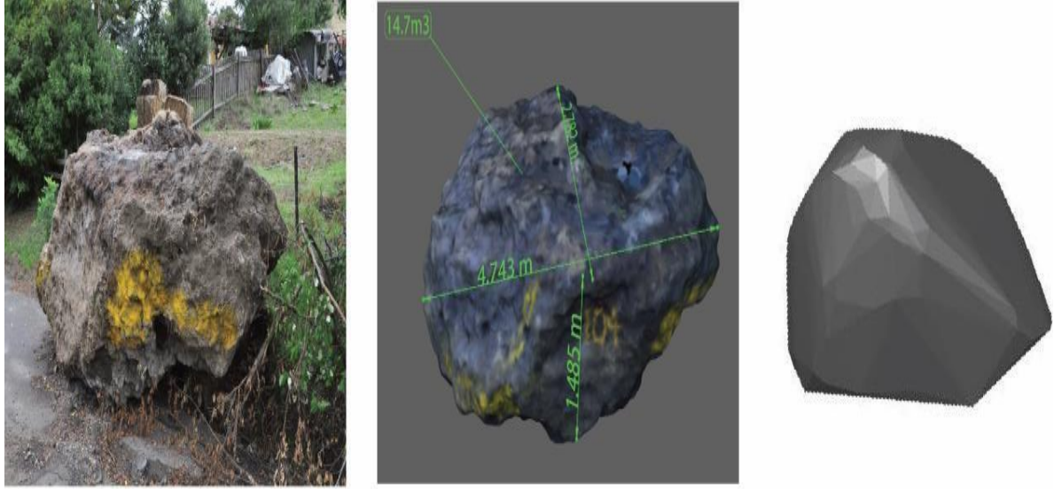
Şekil 3.1. Gerçek Kayaların Lazer Taramaları
