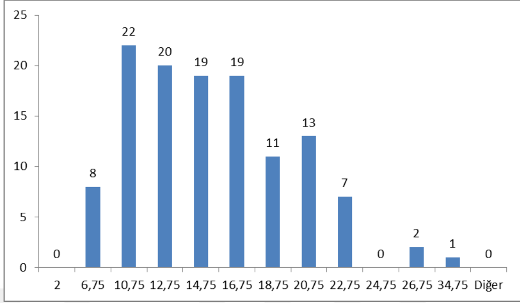
Şekil 4.19. Çinko oranı bakımında popülasyonların frekans dağılımları (mg/kg)
