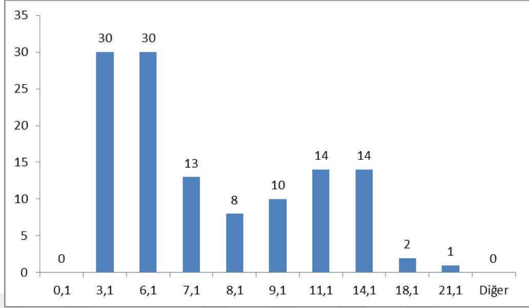
Şekil 4.13. Bakır oranı bakımında popülasyonların frekans dağılımları (mg/kg)
