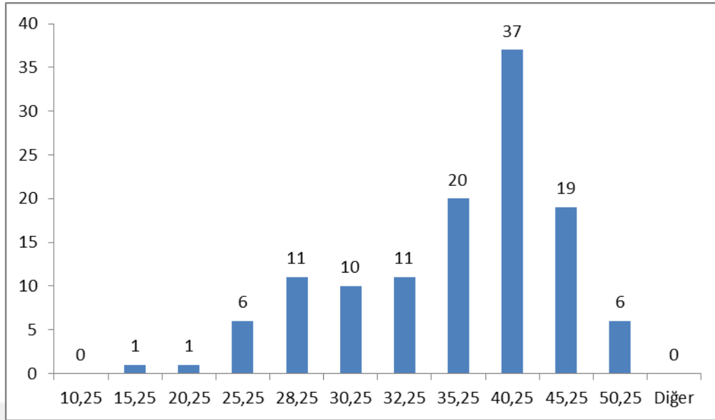
Şekil 4.15. Mangane oranı bakımında popülasyonların frekans dağılımları (mg/kg)
