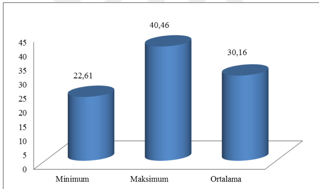
Şekil 4.2. Bin tane ağırlıkları bakımından popülasyona ait ortalama, maksimum ve minimum değerlerin histogramı (g)
