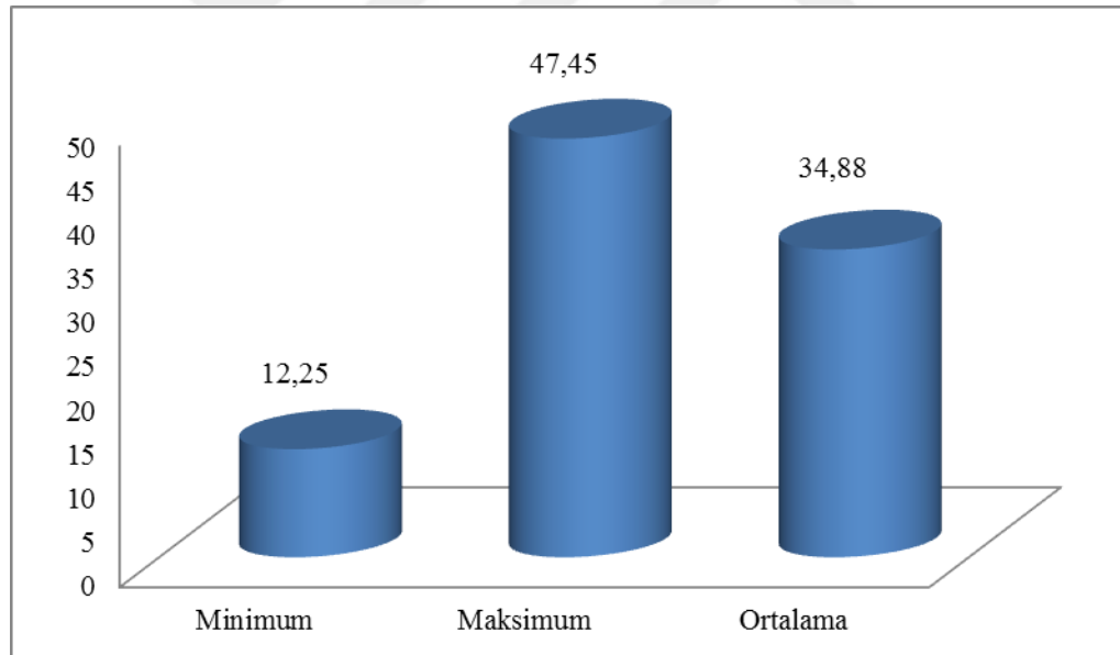
Şekil 4.16. Mangane oranı bakımından popülasyona ait ortalama, maksimum ve minimum değerlerin histogramı (mg/kg)
