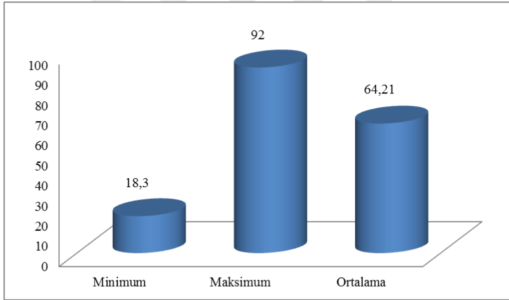
Şekil 4.4. Hektolitre ağırlıkları bakımından popülasyona ait ortalama, maksimum ve minimum değerlerin histogramı (kg/hl)
