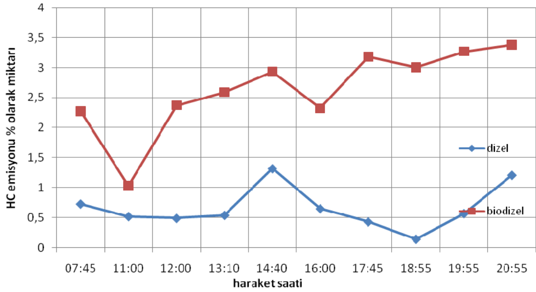
Şekil 4.49. Sabit hız için % olarak HC emisyonu miktarı Üçşhitler-Eminönü
