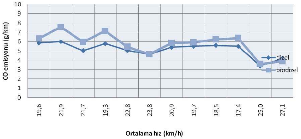
Şekil 4.15. Ortalama hıza göre CO emisyonu (g/km) Eminönü-Üçşehitler
