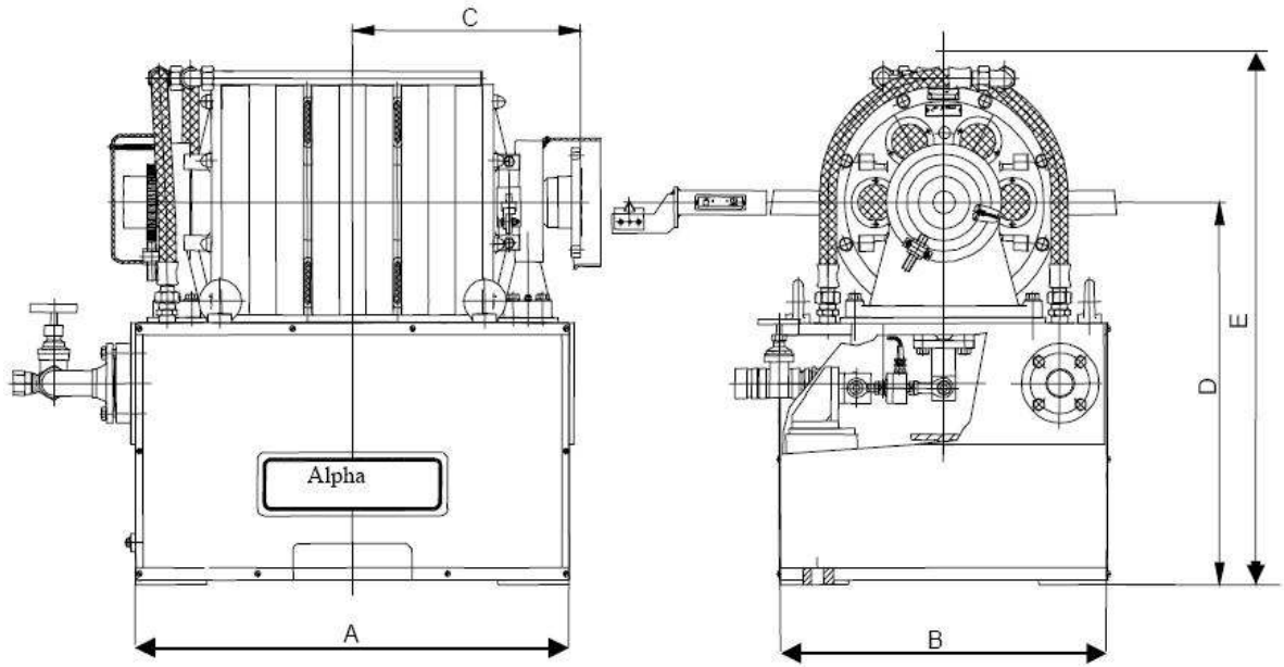
Şekil 2.3. Test dinamometresi
