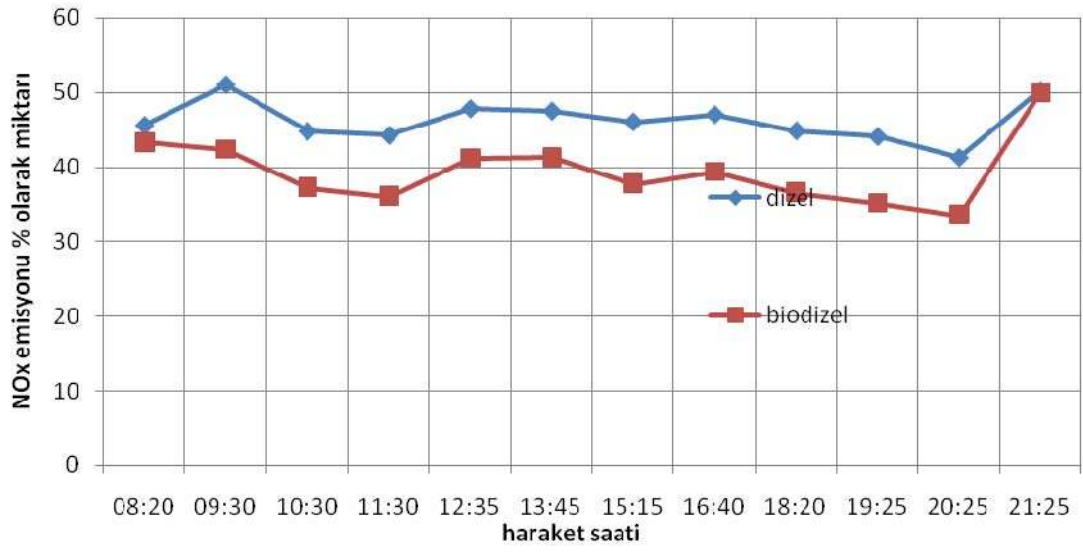
Şekil 4.42. Hızlanma için % olarak NO x emisyonu miktarı Eminönü-Üçşhitler
