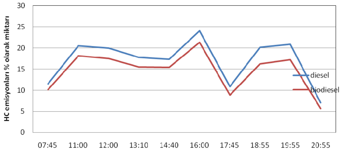
Şekil 4.47. Durma anları için % olarak HC emisyonu miktarı Üçşehitler-Eminönü
