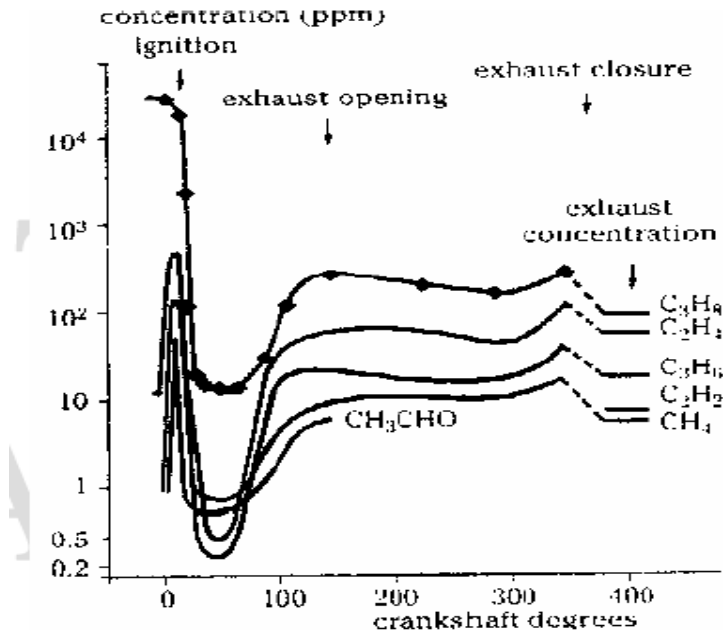
Şekil 1.9. Çevrim esnasında değişik yanmamış hidrokarbonların konsantrasyonu.
