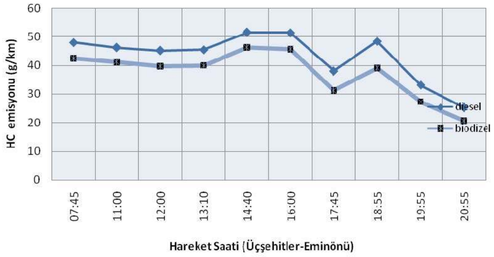
Şekil 4.46. Hareket saatine göre HC emisyonları (kg/km) Üçşehitler-Eminönü
