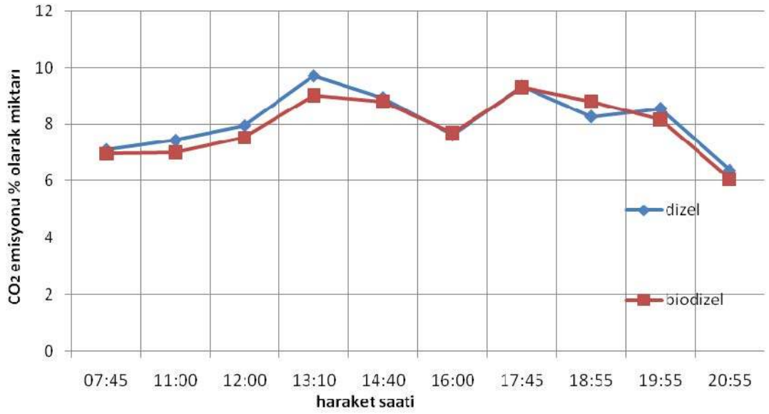
Şekil 4.25. Sabit hız için % olarak CO 2 emisyonu miktarı Üçşehitler-Eminönü
