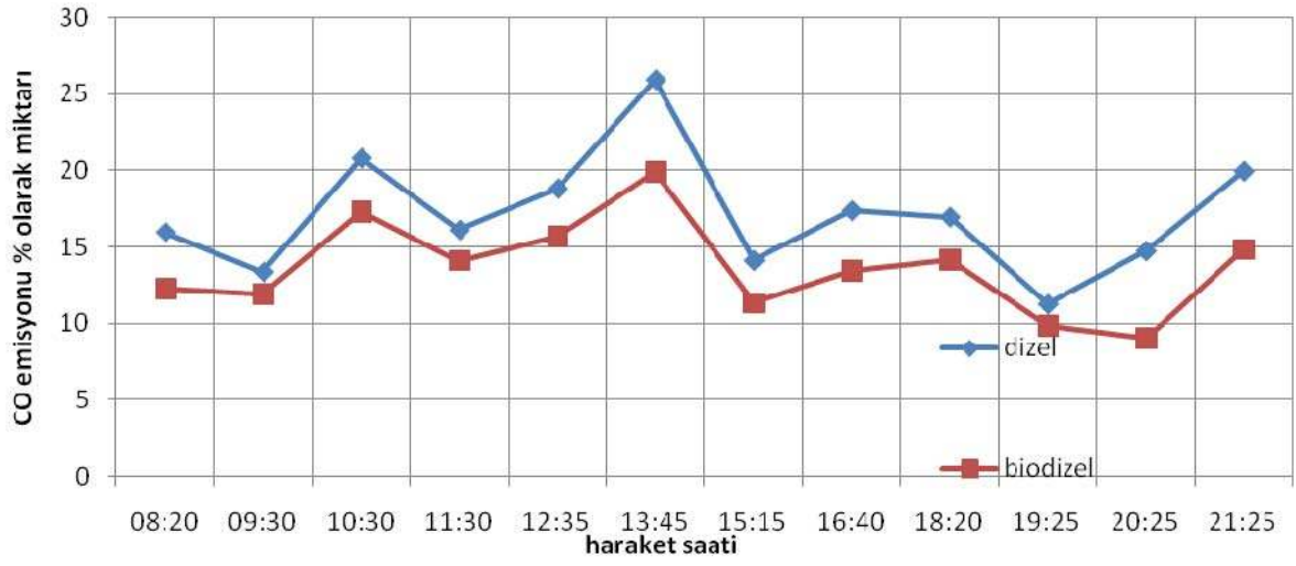
Şekil 4.20. Yavaşlama için % olarak CO emisyonu miktarı Eminönü-Üçşehitler
