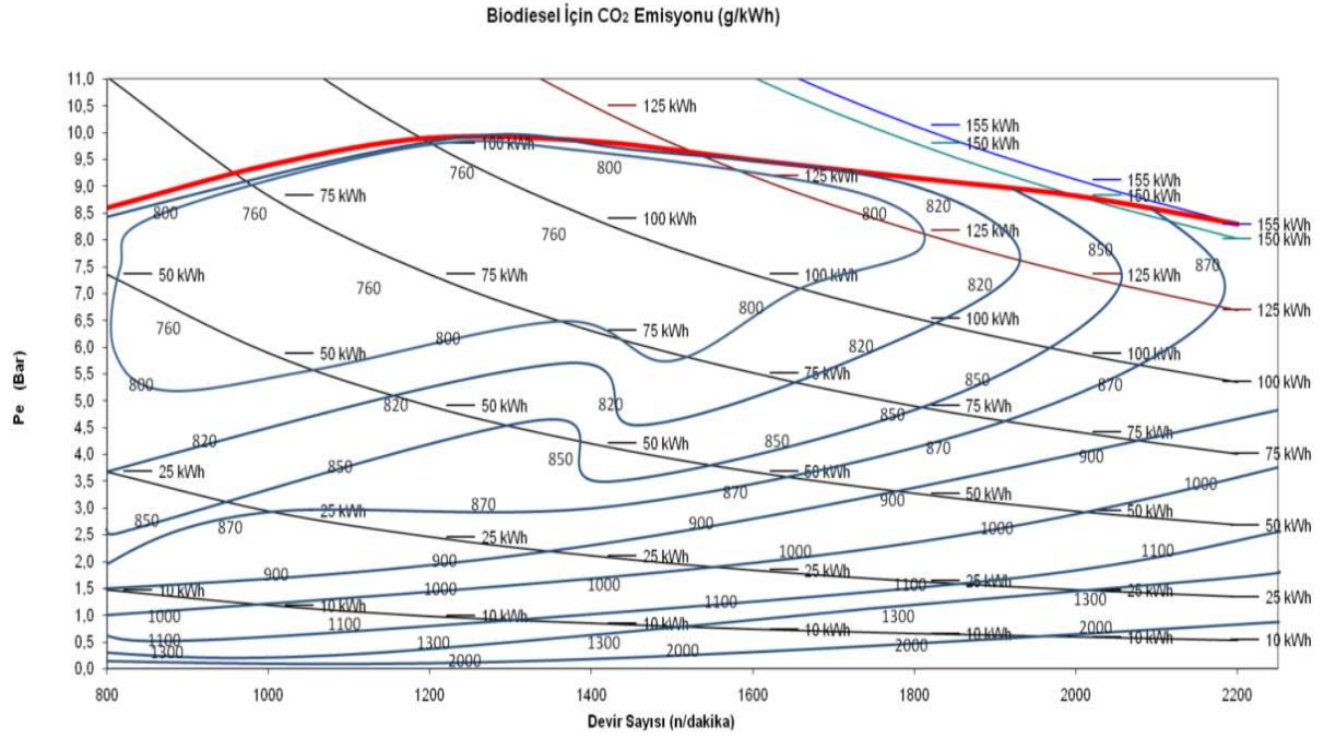
Şekil 4.4. Biodiesel yakıt için CO 2 emisyonu miktarı (g/kWh)
