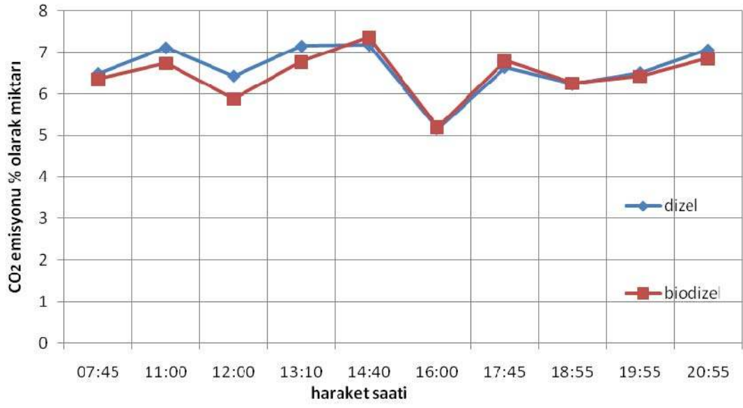
Şekil 4.26. Yavaşlama için % olarak CO 2 emisyonu miktarı Üçşhitler-Eminönü
