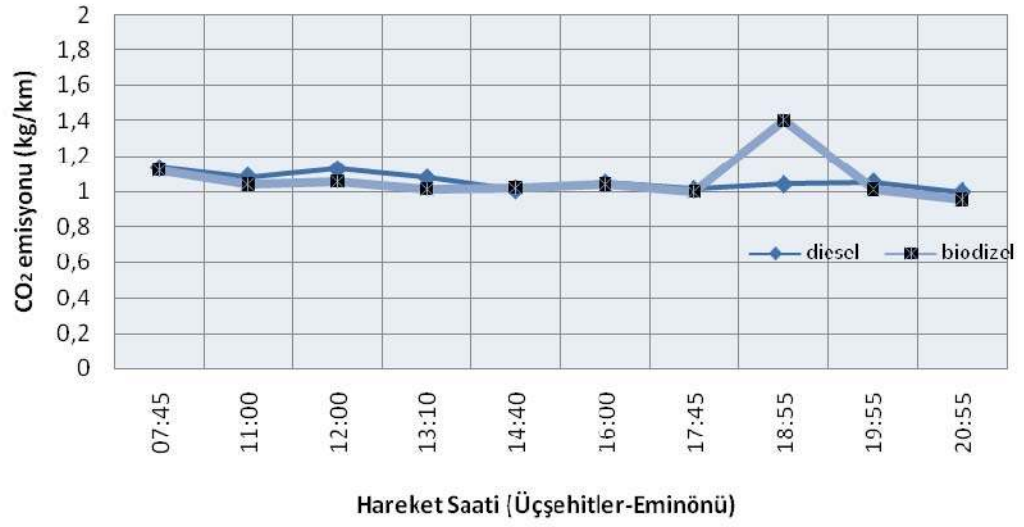
Şekil 4.22. Hareket saatine göre CO 2 emisyonları (kg/km) Üçşehitler-Eminönü
