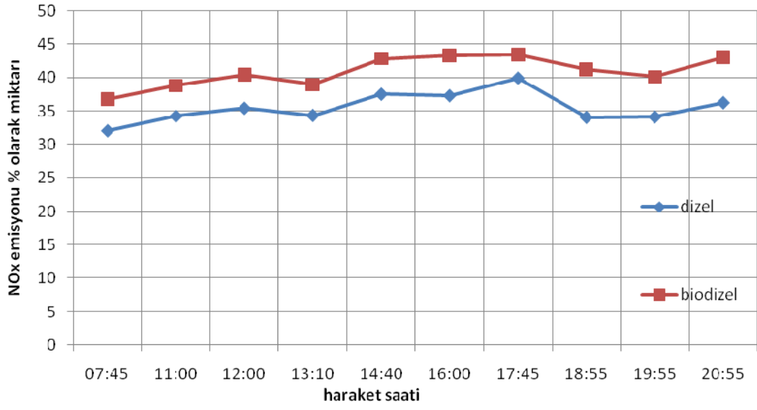
Şekil 4.38. Yavaşlama için % olarak NO x emisyonu miktarı Üçşehitler-Eminönü
