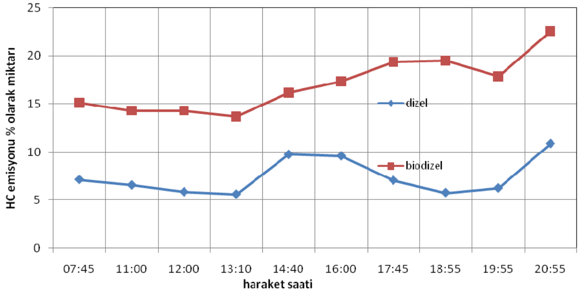
Şekil 4.48. Hızlanma için % olarak HC emisyonu miktarı Üçşhitler-Eminönü
