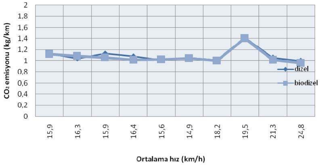
Şekil 4.21. Ortalama hıza göre CO 2 emisyonu (kg/km) Üçşehitler-Eminönü
