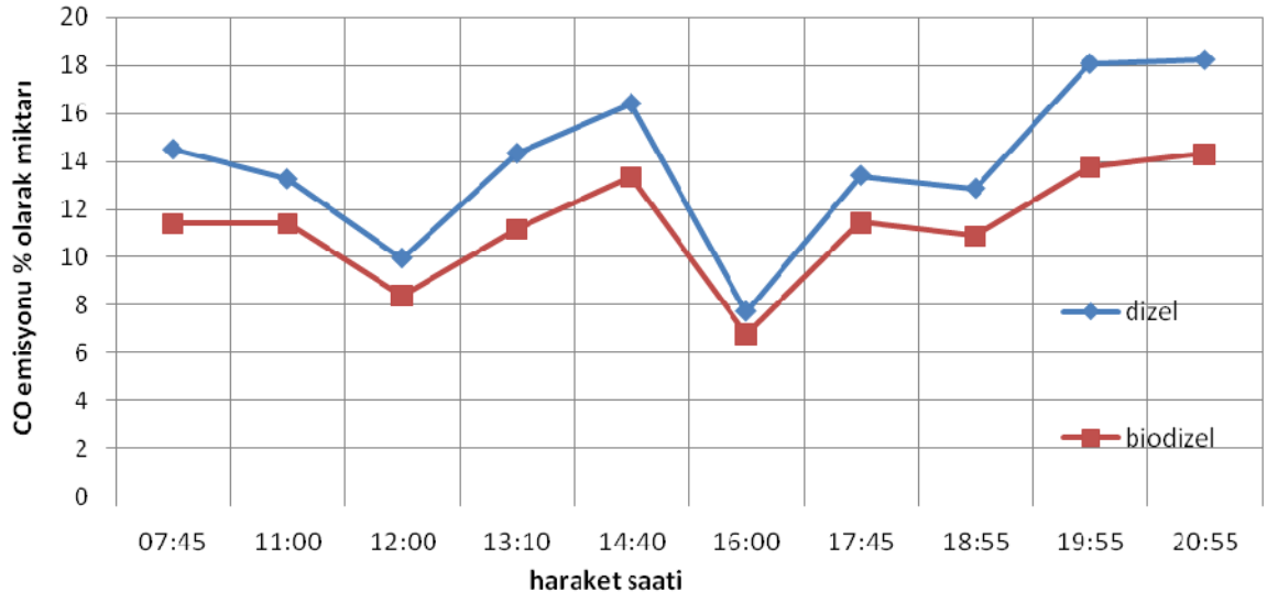
Şekil 4.14. Yavaşlama için % olarak CO emisyonu miktarı Üçşehitler-Eminönü
