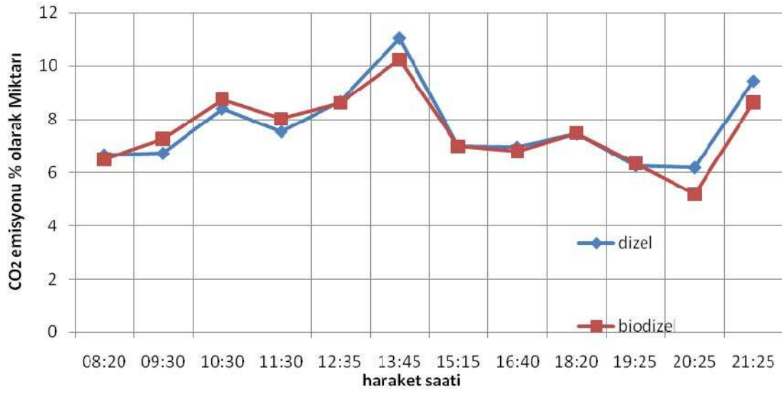
Şekil 4.32. Yavaşlama için % olarak CO 2 emisyonu miktarı Eminönü-Üçşehitler
