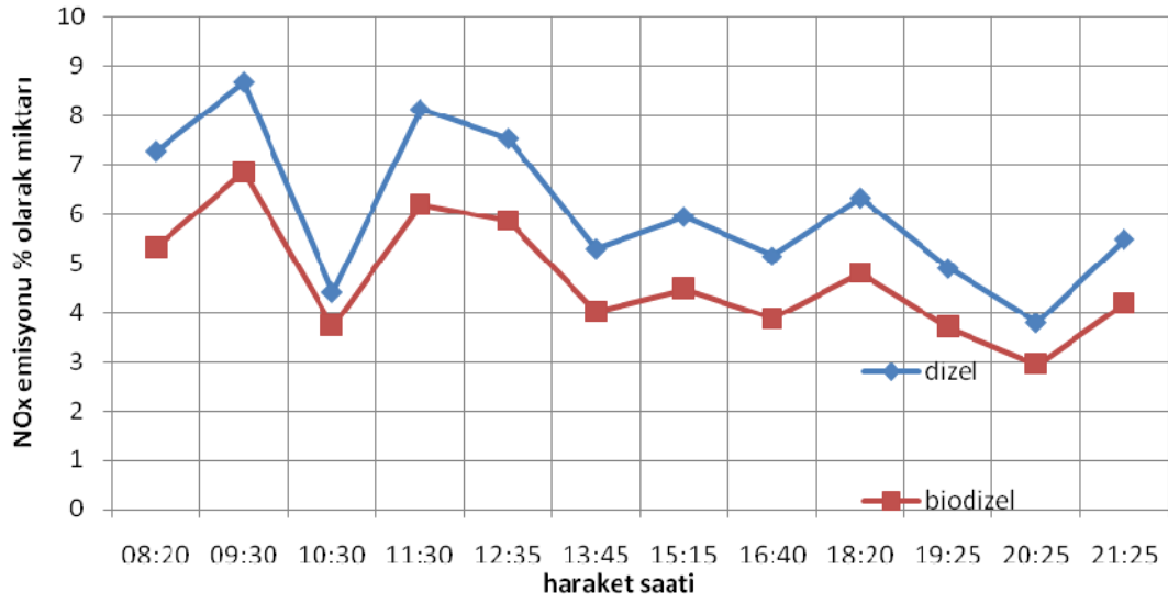
Şekil 4.43. Sabit hız için % olarak NO x emisyonu miktarı Eminönü-Üçşhitler
