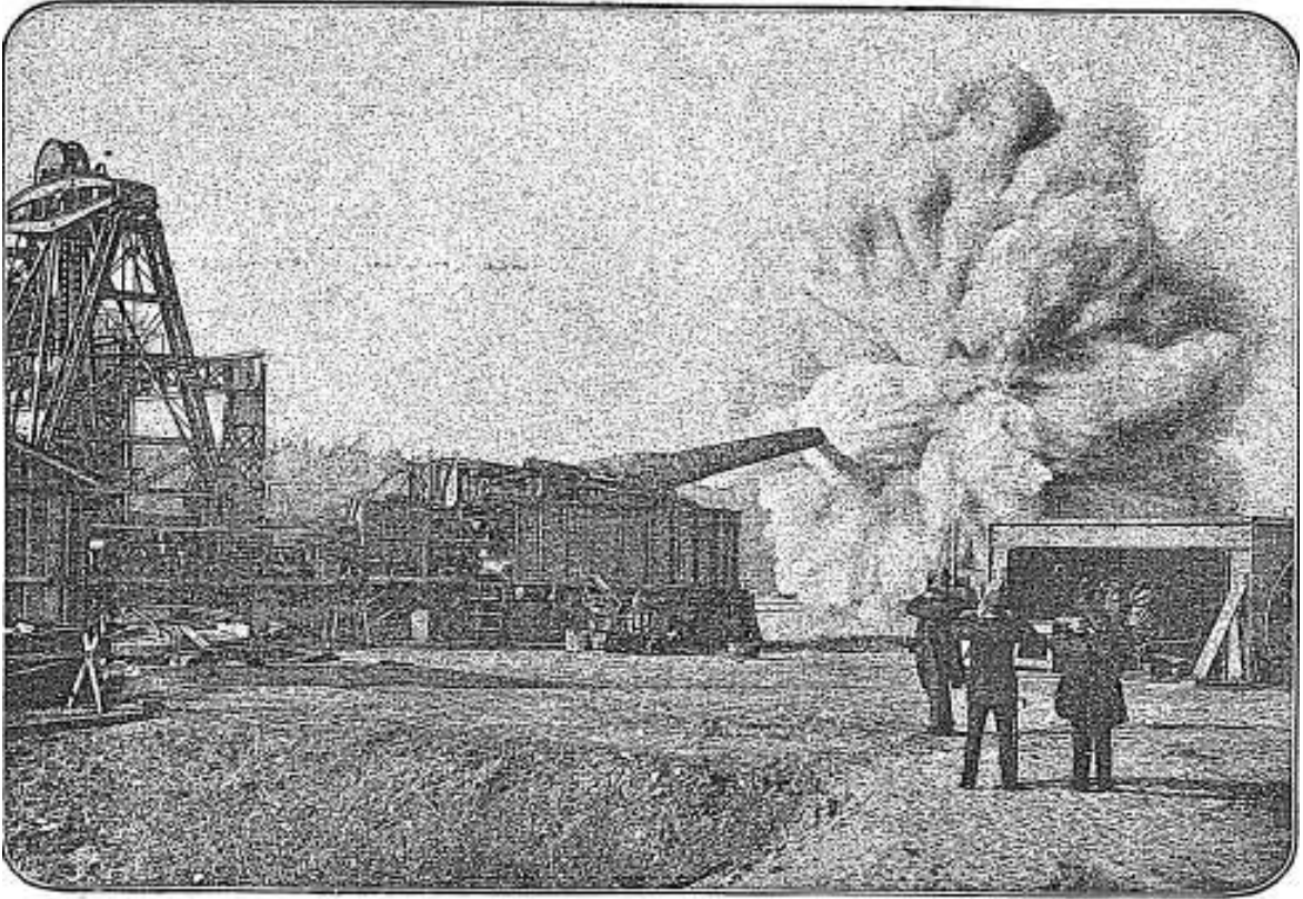
Kruppun 30 buçuk sântimetre katrında idrolik ya'ni tazyik-i bi'lmâ' usulüyle idâre olunur sevâhil ve sefâi'n topu
