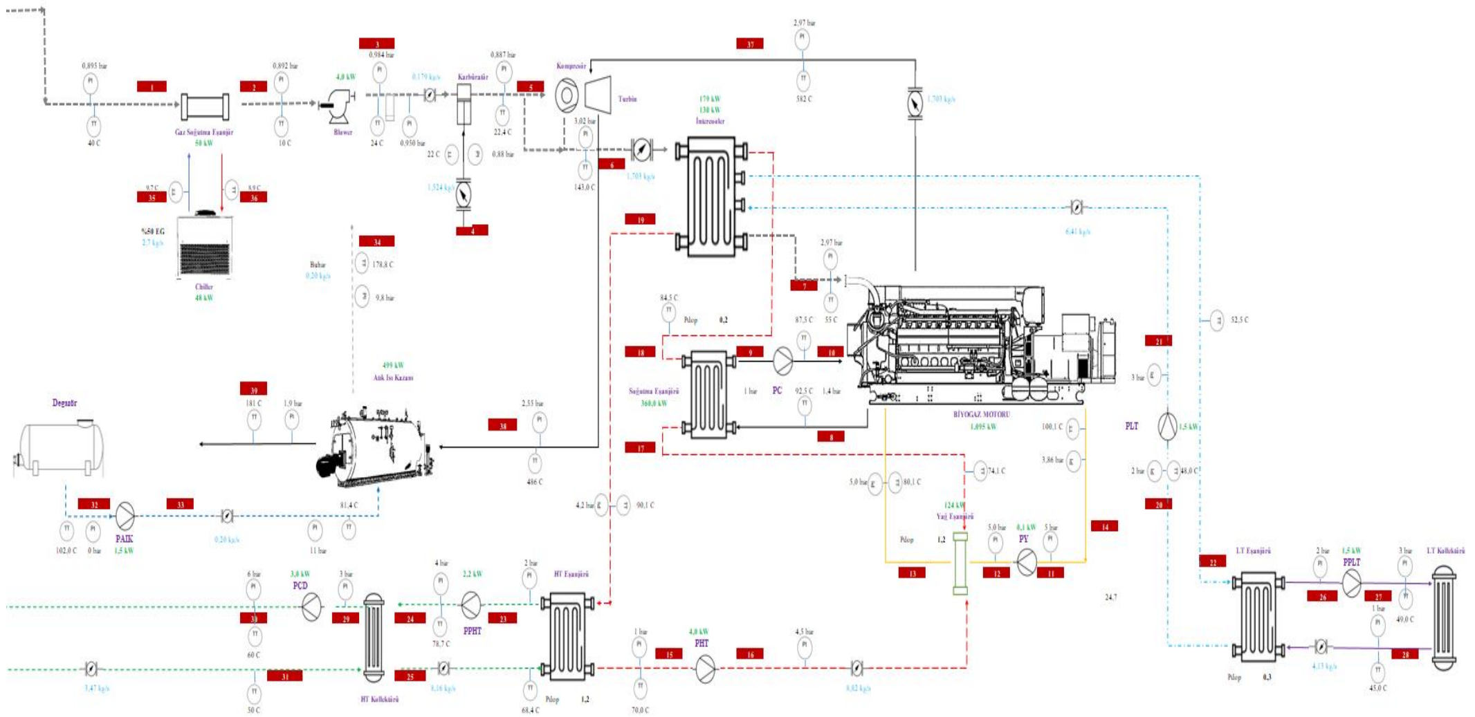
Şekil 6.39. Kojenerasyon sistemi
