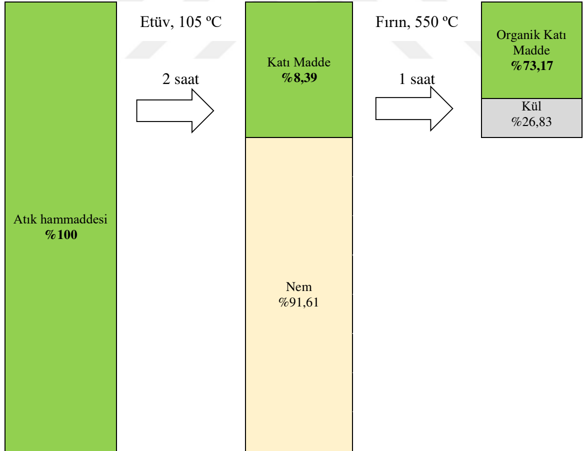
Şekil 6.24. Atık hammadde kütle dengeliği
