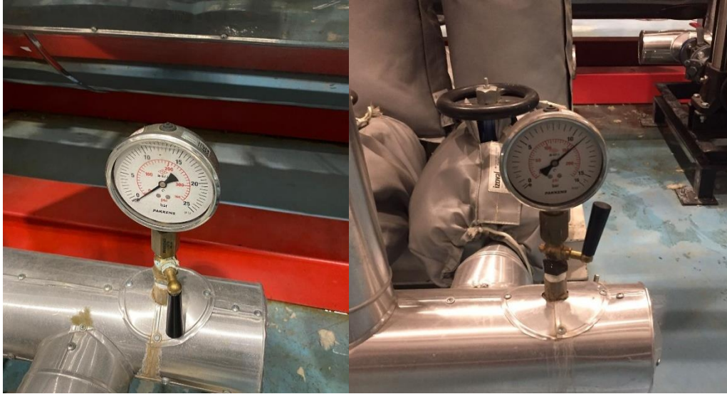
Şekil 6.76. Atık ısı kazanı besli suyu pompa öncesi ve sonrası basınçlar
