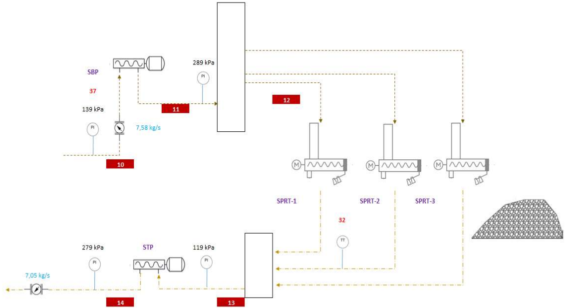
Şekil 6.36. Susuzlaştırma Sistemi
