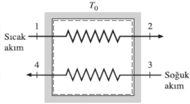
Şekil 6.56. Isı değiştirici akış şeması
