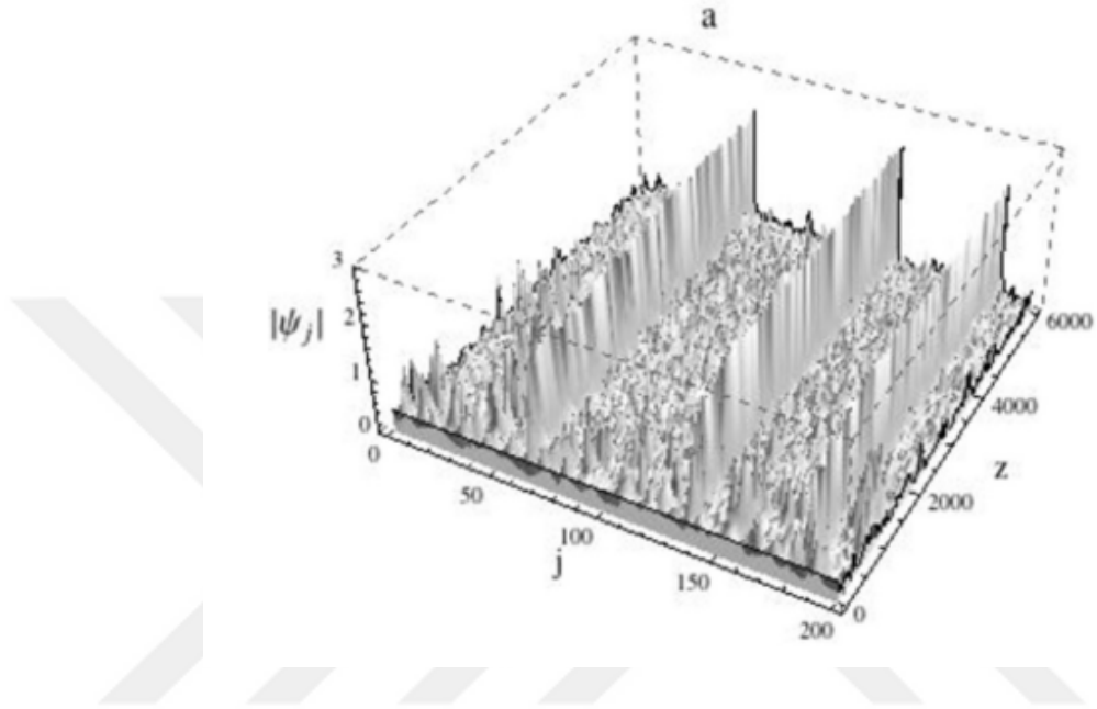
Şekil 4.12: \varepsilon_2=10^{-2} , g=-1 , N=200 ve A=0.4 için \psi_j(z=0)=A alınması durumunda uzun süreli rogue dalgası
