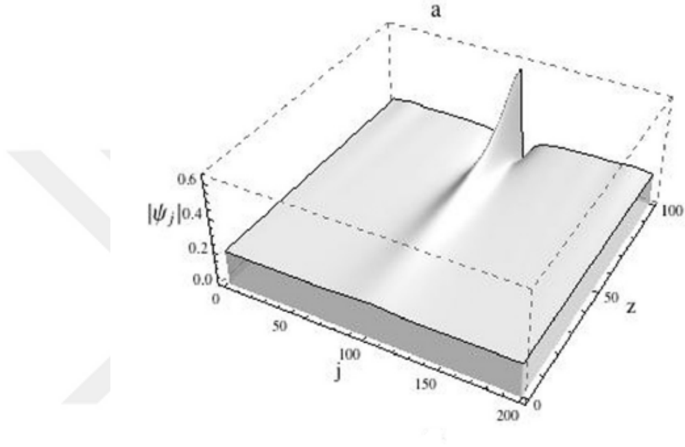
Şekil 4.6: Herhangi bir düzensizliğin olmadığı durumda N=200 , L=100 , g=-1 ve A=0.2 değerleri için alan genliğinin mutlak değeri
