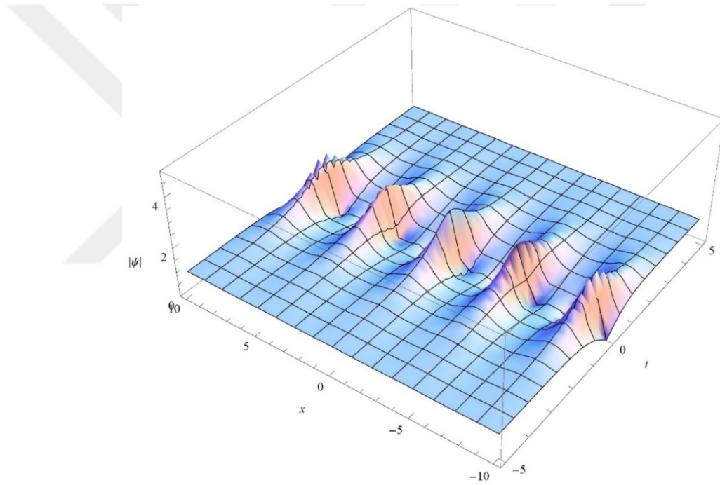
Şekil 3.7: Akhmediev Breather çözümünde a=0.25 değeri için dalga fonksiyonunun mutlak değerinin konum-zaman grafiği
