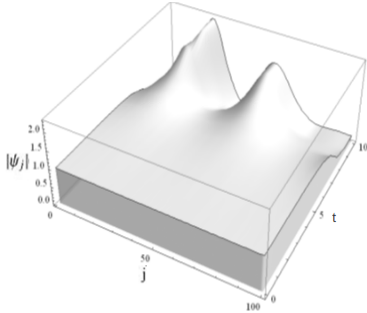
Şekil: 4.2: N=100 , A=1 ve L=100 değerleri için dalga fonksiyonu genliğinin mutlak değerinin konum-zaman grafiğı
