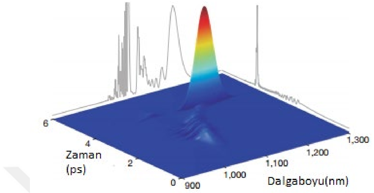
Şekil 2.8: Optikte rogue dalgalarının zaman-dalga boyu ilişkisi(Solli et al., 2007)
