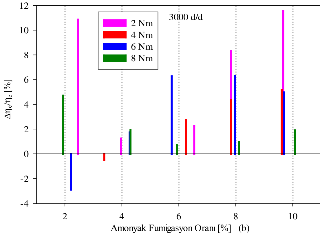
Şekil 31. 3000 d/d'da; (a) Etkif verimin AF oranlarına göre değışimleri, (b) Etkif verim değışiminin AF oranlarına göre değışimleri
