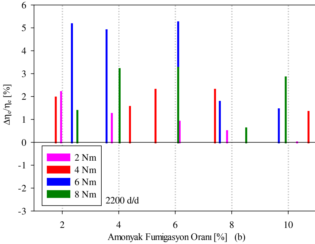
Şekil 25. 2200 d/d'da; (a) Etkatif verimin AF oranlarına göre değişimleri, (b) Etkatif verim değişiminin AF oranlarına göre değişimleri
