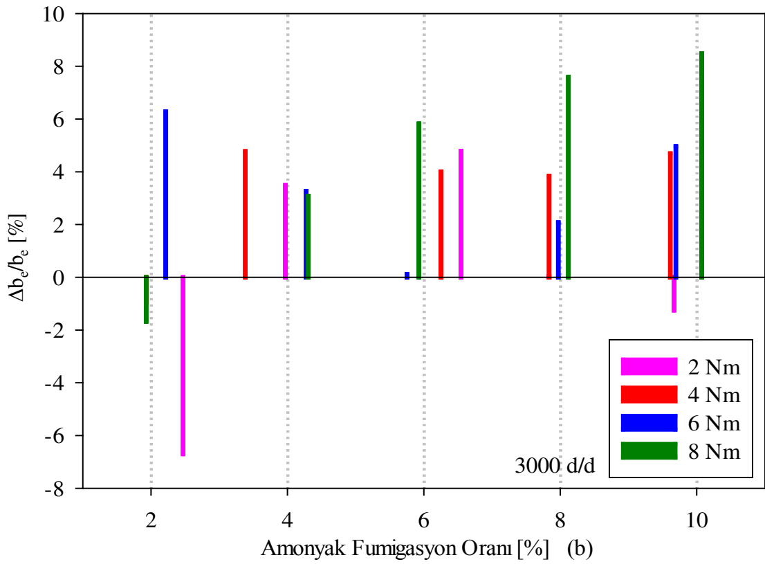
Şekil 30. 3000 d/d'da; (a) ÖYT'nin AF oranlarına göre değişimleri, (b) ÖYT değişiminin AF oranlarına göre değişimleri
