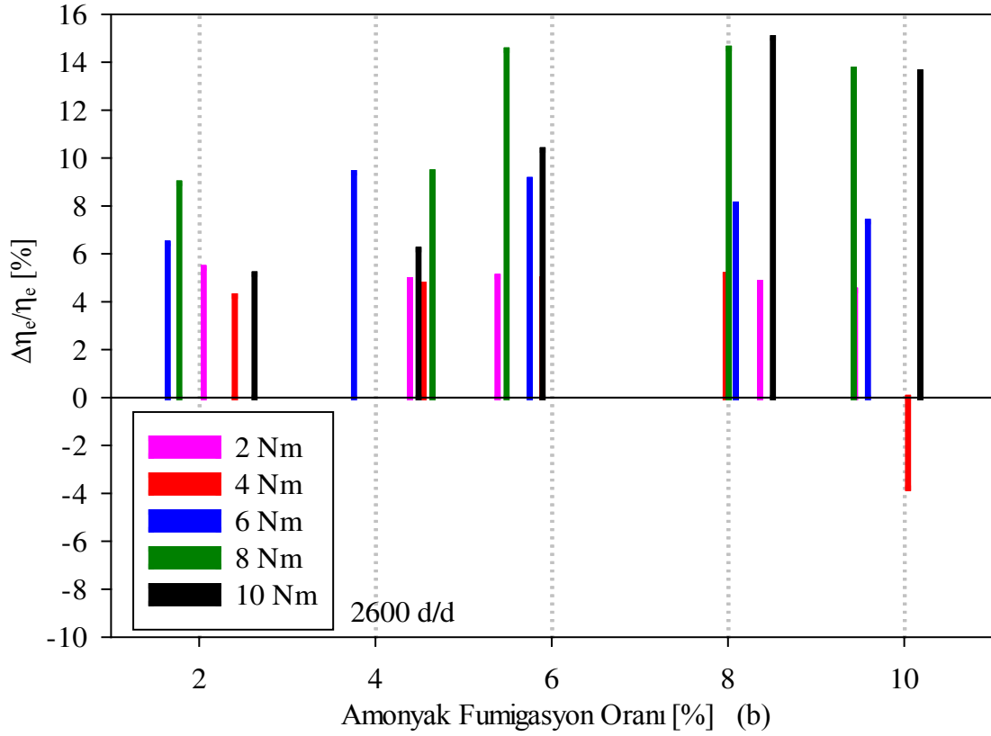
Şekil 28. 2600 d/d'da; (a) Efektif verimin AF oranlarına göre değişimleri, (b) Efektif verim değişiminin AF oranlarına göre değişimleri
