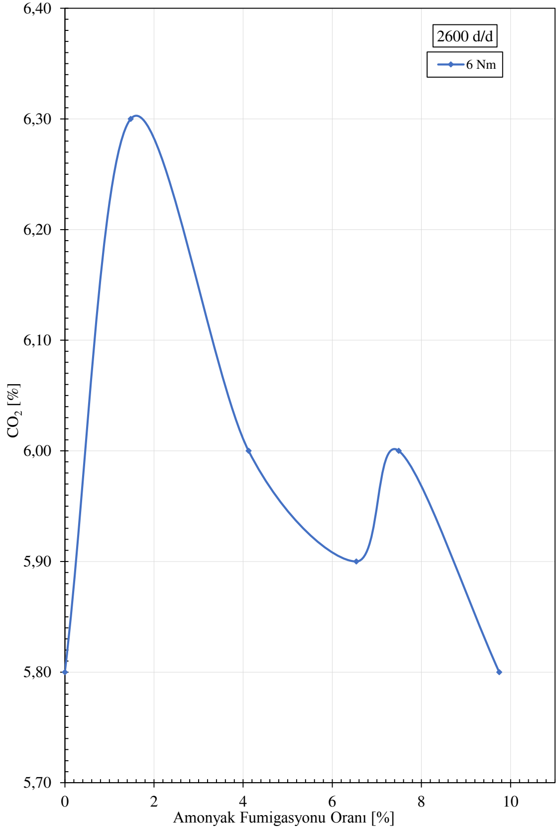
Şekil 43. 2600 d/d'da 6 Nm yük değeri için CO 2 emisyonunun AF oranına göre değişimi
