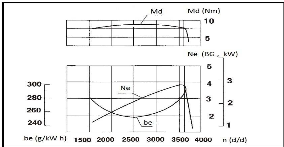
Şekil 4. Deneylerde kullanılan Palmera PA-HP170F dizel motor karakteristikleri
