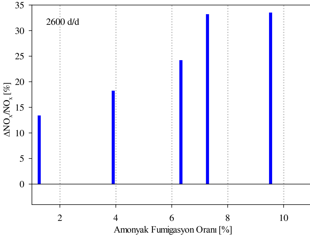
Şekil 48. 2600 d/d’da 6 Nm yük değeri için NO x emisyonu değişim oranının AF oranına göre değişimleri
