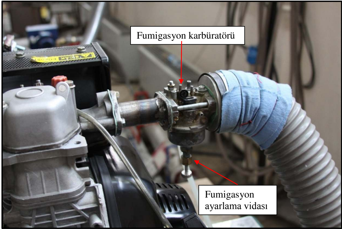
Şekil 5. Deneylerde kullanılan modifiye karbüratör ve motor gövdesine bağlantısı
