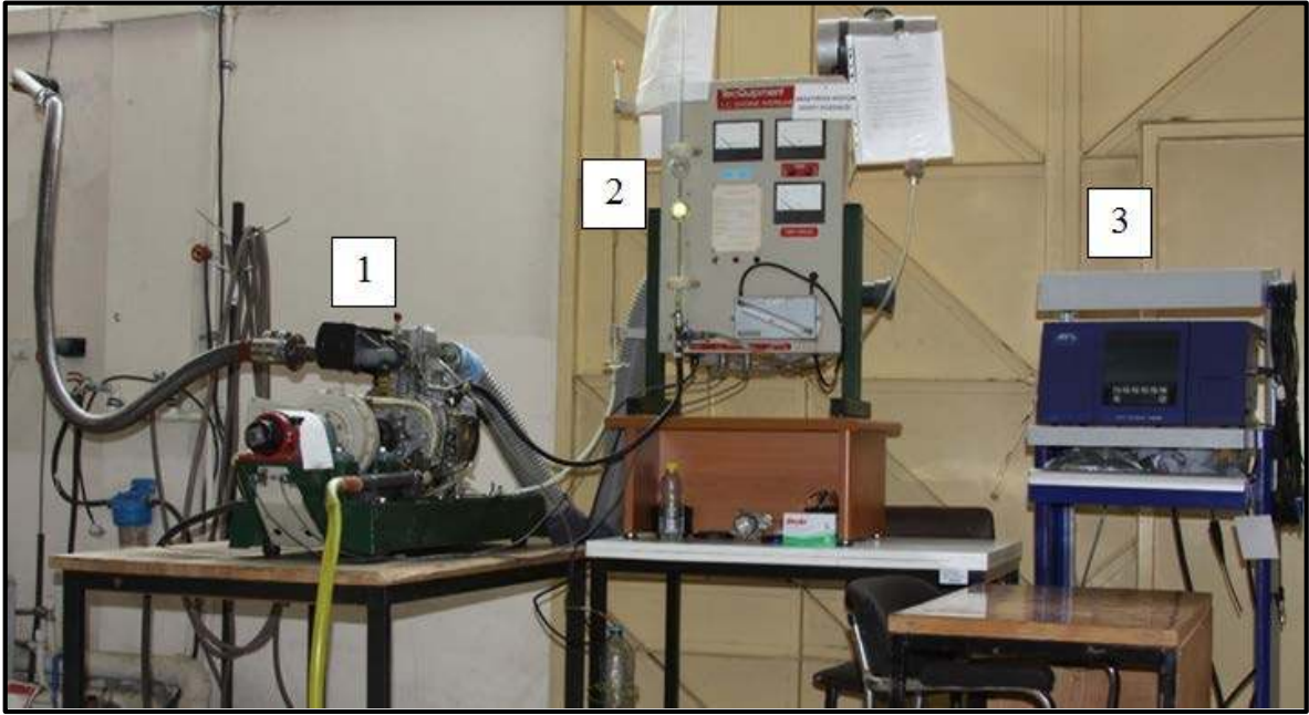
Şekil 1. TD114 küçük araştırma motor deney düzeneđi (1-Araştırma deney motoru, 2-Gösterge panosu, 3-Eksoz gazı analiz cihazı).
