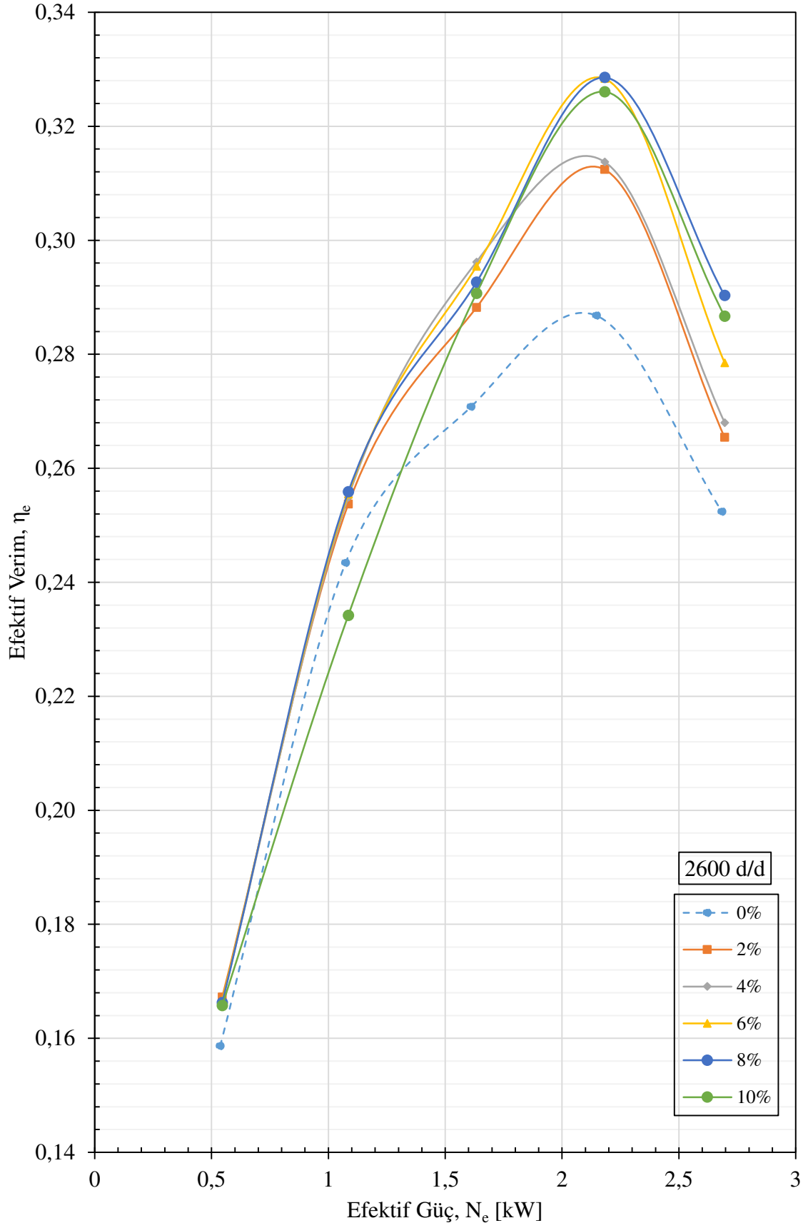
Şekil 19. 2600 d/d'da farklı AF oranları için efektif verimin efektif güçte göre değişimleri
