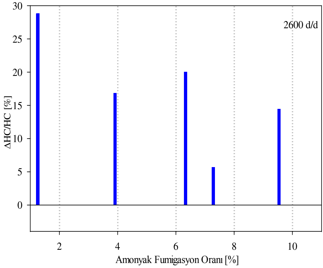
Şekil 46. 2600 d/d'da 6 Nm yük değeri için HC emisyonu değişim oranının AF oranına göre değişimleri
