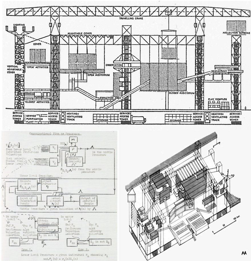
Şekil 3.6: “Programatik ve mekansal yapılanmalar” (Mathews, 2006a).
