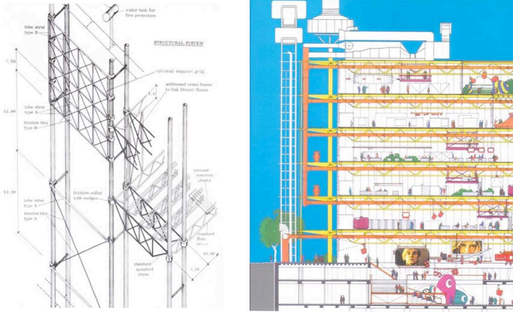
Şekil 4.15: Strüktürel çelik tasarımda “ prefabrikasyon parçalar montajı ”(Branda, 2012).
