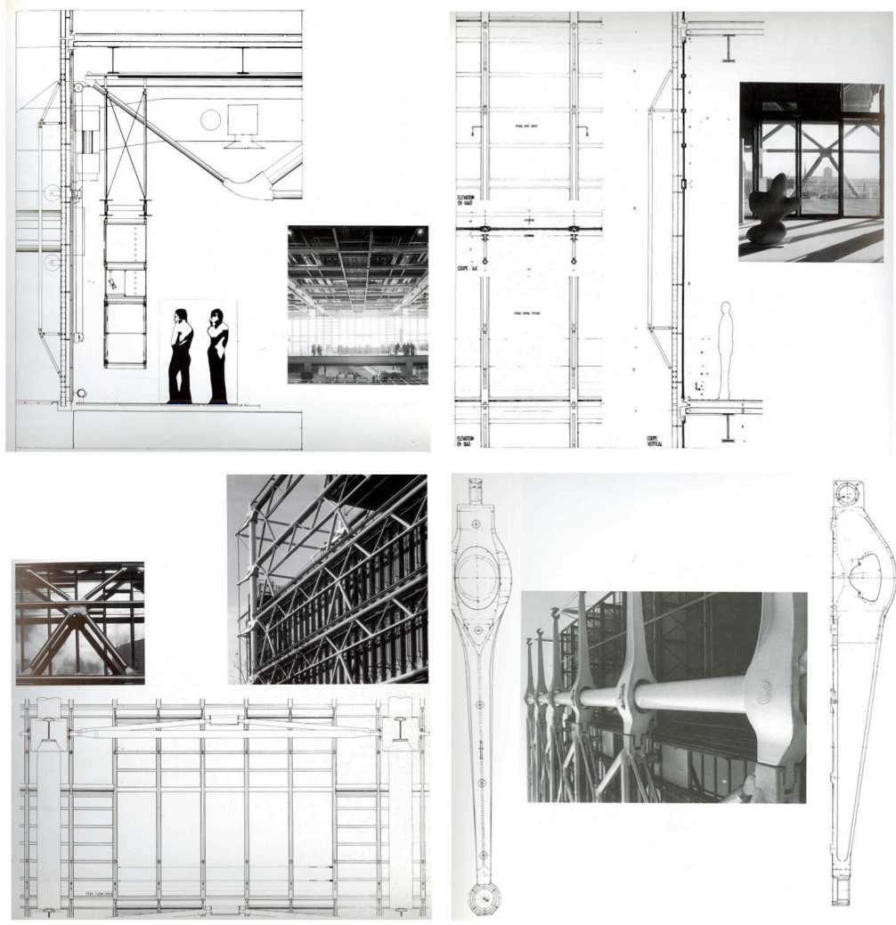
Şekil 4.16: Mekanın “ strüktürel alanı ”na dair çözümler (Burdett, 1996).
