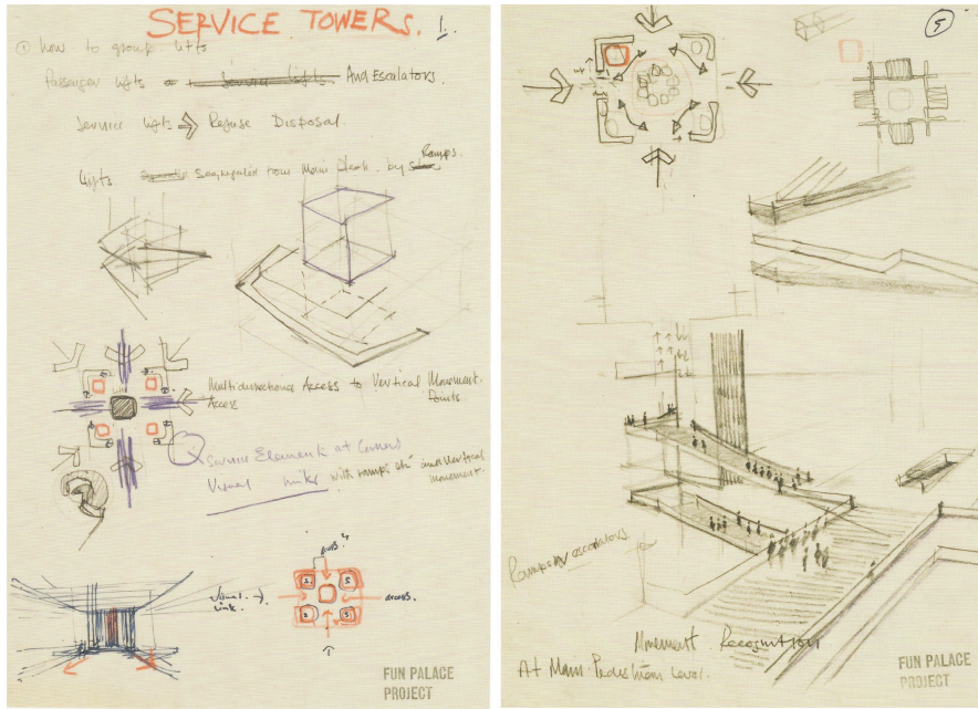
Şekil 3.12: “Servis kulelerinin etrafında olabilecek mekansal kurgular”(Mathews, 2007).
