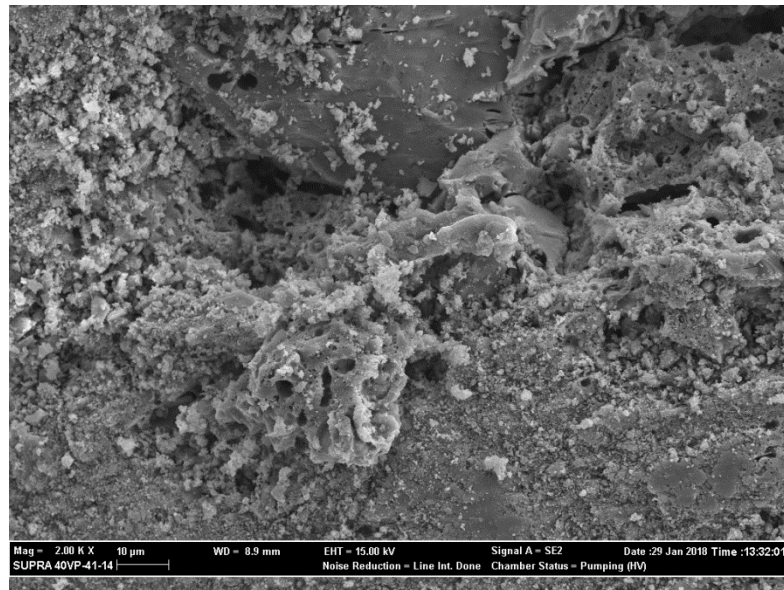
Şekil 4. 113. THY-8 numunesine ait ayrıntılı SEM görüntüsü (10 μm)
