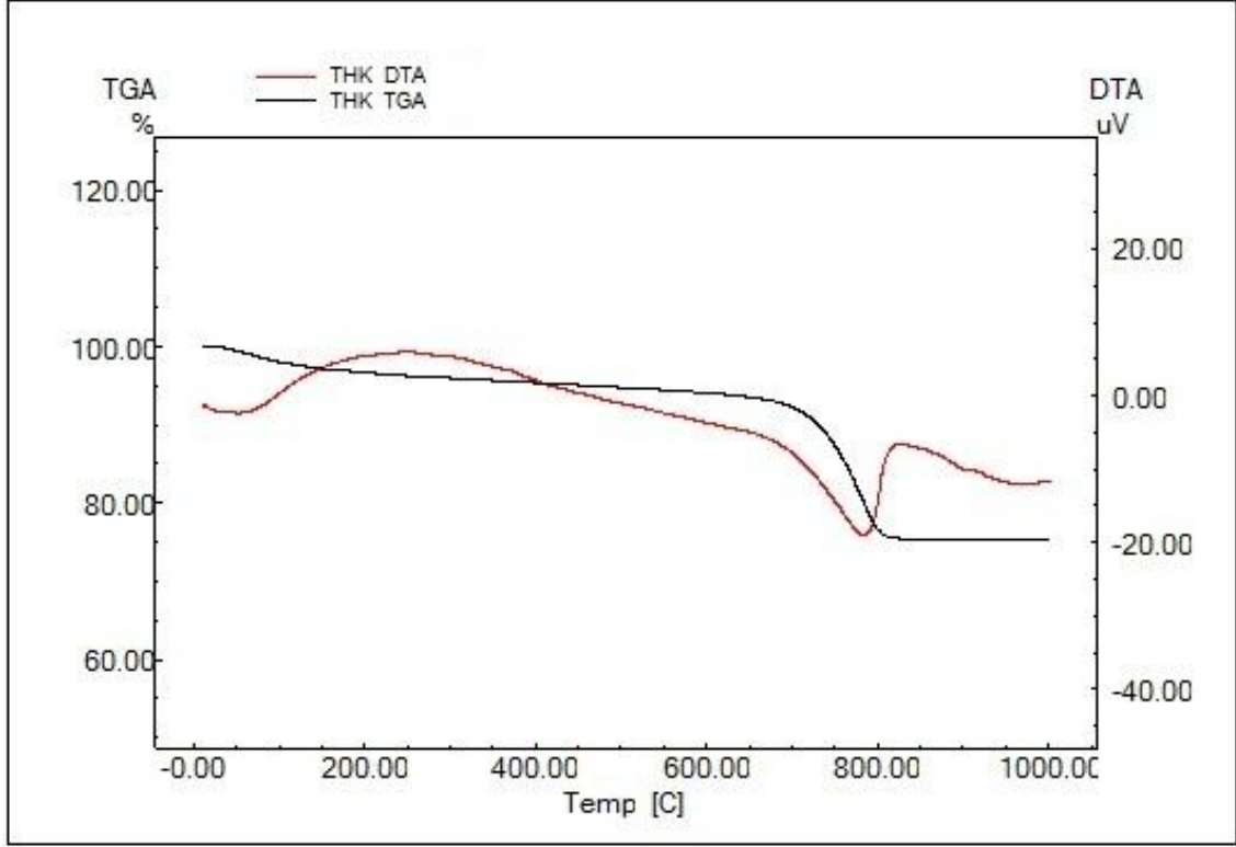
Şekil 4. 56. THK-1 numunesine ait TG-DTA analiz sonucu
