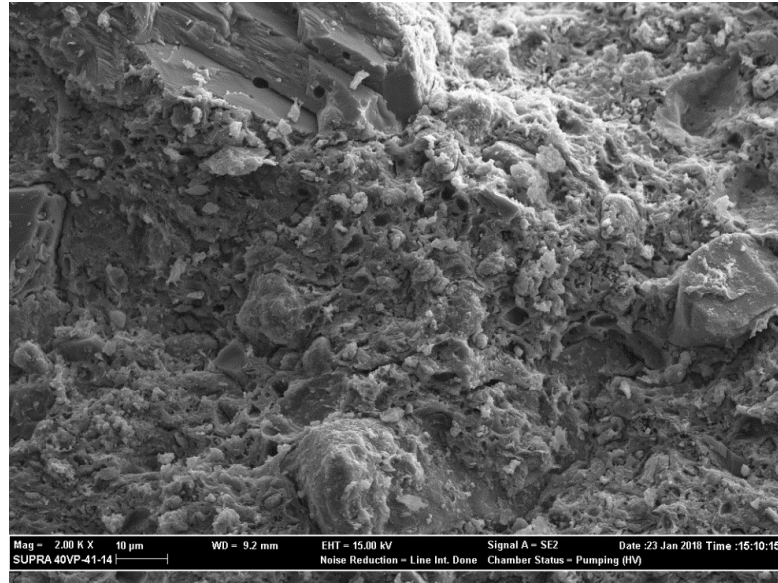
Şekil 4. 83. THK-2 numunesine ait ayrıntılı SEM görüntüsü (10 µm)
