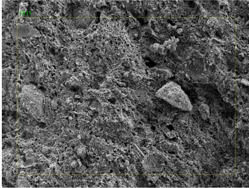
Şekil 4. 124. THY-14 numunesine ait SEM görüntüsü (100 μm)
