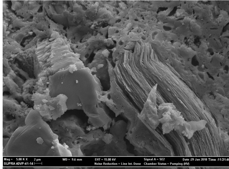
Şekil 4. 109. THY-6 numunesine ait ayrıntılı SEM görüntüsü (10 \mu\text{m} )
