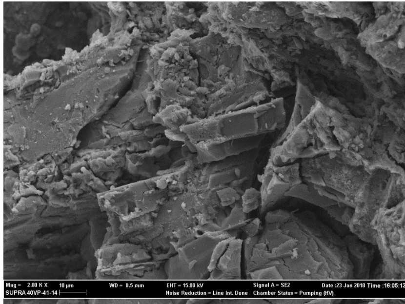
Şekil 4. 89. THK-5 numunesine ait ayrıntılı SEM görüntüsü (10 μm)
