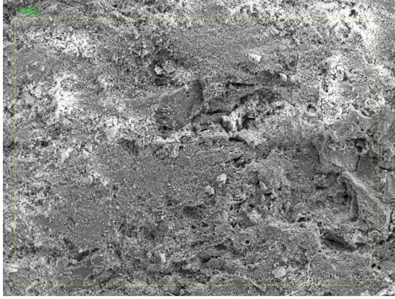
Şekil 4. 112. THY-8 numunesine ait SEM görüntüsü (100 μm)
