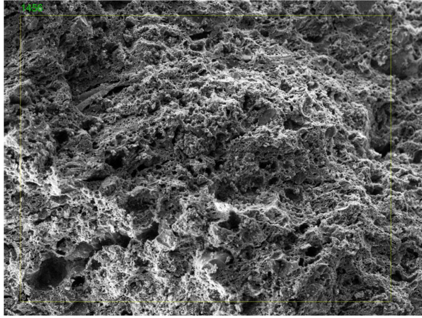
Şekil 4. 120. THY-12 numunesine ait SEM görüntüsü (100 \mu\text{m} )
