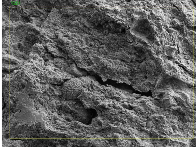
Şekil 4. 84. THK-3 numunesine ait SEM görüntüsü (100 μm)
