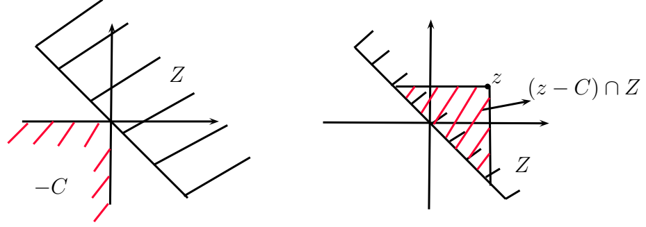
Şekil 3.25. Z = \{(z_1, z_2) : z_1 + z_2 \geq 0\} kümesinin C -kompakt fakat kompakt olmadığıının gösterimi
