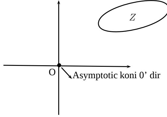
Şekil 2.23. Z kümesinin sınırlı olması durumunda asymptotic koni
