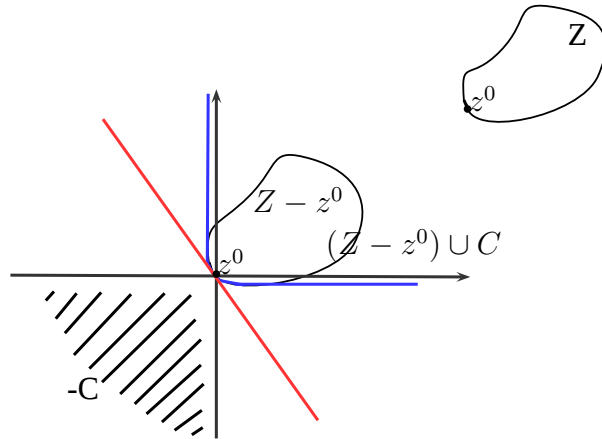
Tanım 2.2.8. z^0 etkin ve cl(conv(cone [(Z - z^0) \cup C])) \cap (-C) = \{0\} oluyorsa, z^0 \in Z değerine Hurwicz has etkin nokta denir. Hurwicz has etkin değerler kümesi z^0 \in PE(Z)_{Hu} şeklinde gösterilir.
