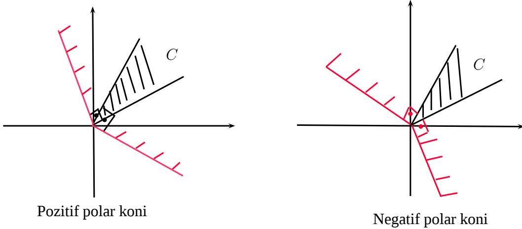
Şekil 1.2. C 'nin pozitif ve negatif polar konileri
