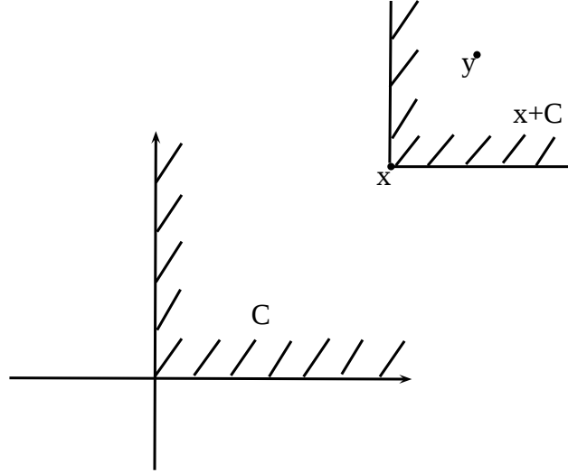
Şekil 1.1. C 'nin pozitif ve negatif polar konileri
