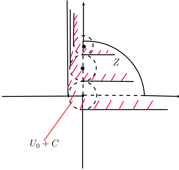
Şekil 3.29. Z = \{(z_1, z_2) : z_1^2 + z_2^2 \leq 1, z_1 > 0, z_2 > 0\} \cup \{(0, 0)\} kümesinin Luc'un tanımına göre C -kompakt oluşunun geometrik ifadesi
