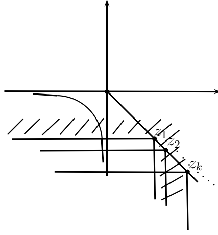
Şekil 3.36. Sonlu örtüye sahip olmayan Z = \{(z_1, z_2) : z_2 < 0, z_1 z_2 = 1\} \cup \{(z_1, z_2) : z_2 \leq 0, z_2 = -z_1\} kümesinin C -yarıkompakt olmadığının geometrik yorumu
