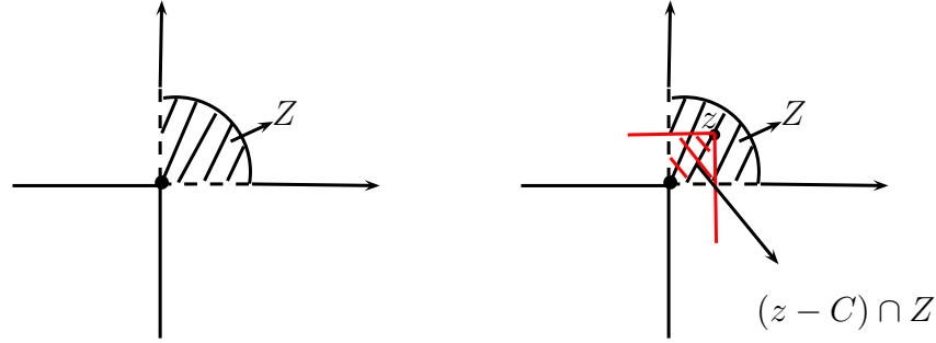
Şekil 3.26. Z = \{(z_1, z_2) : z_1^2 + z_2^2 \leq 1, z_1 > 0, z_2 > 0\} \cup \{(0, 0)\} kümesinin C -kompakt olmadığının gösterimi
