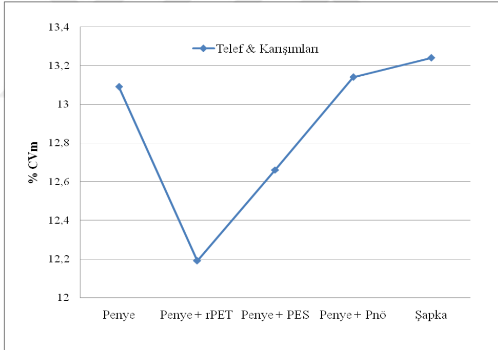
Şekil 4.32 : Ne 16/1 OE-Rotor ipliklere ait düzgünsüzlük sonuçları
