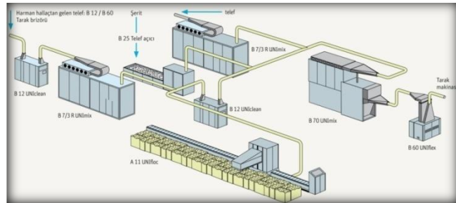
Şekil 2.1 : Telef değerlendirme için örnek bir proses akışı ve geri kazanım tesisi a) örnek bir proses akışı b) geri kazanım tesisi [17]
