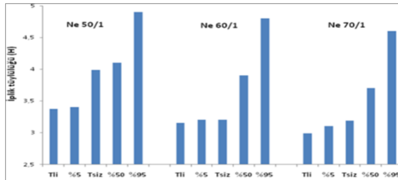
Şekil 4.15 : İplik tüylülüğü
