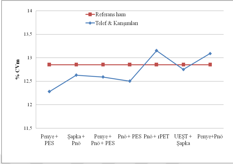
Şekil 4.31 : Ne 20/1 OE-Rotor ipliklere ait düzgünsüzlük sonuçları
