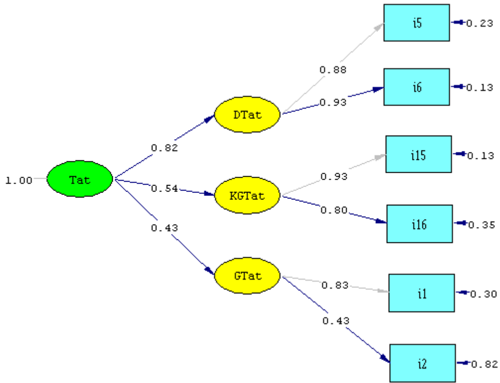
Şekil 8. İş Tatmini İkinci Düzey Doğrulamalı Faktör Analizine İlişkin Path Diyagramı
