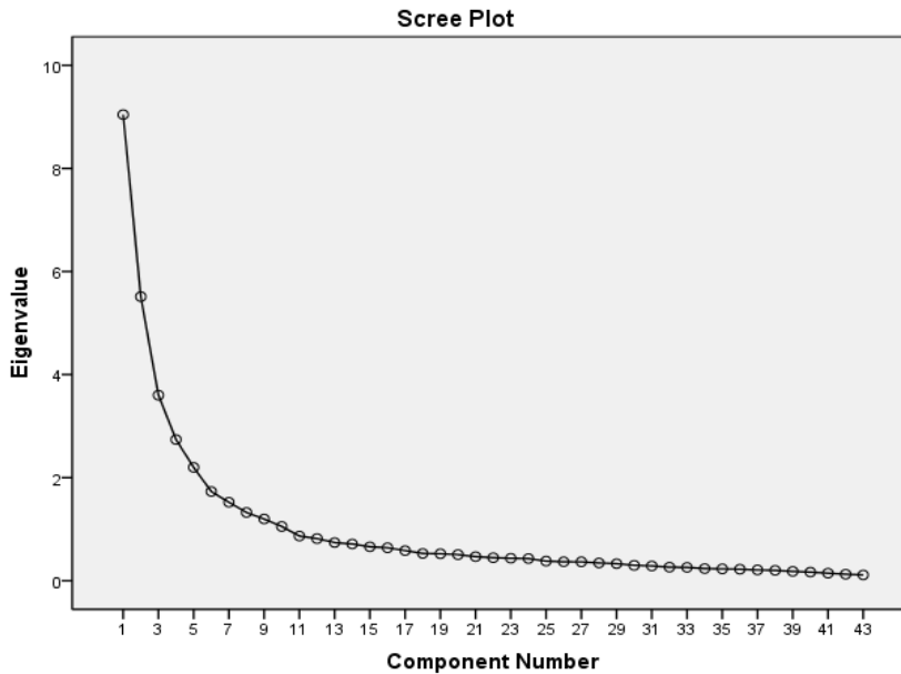
Şekil 3.1 Scree Plot
