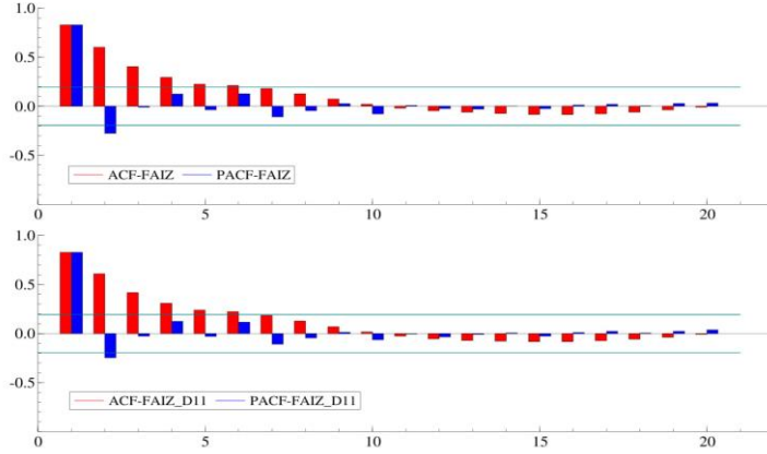
Şekil 4. Mevsimsellikten Arındırılmış ve Arındırılmamış FAIZ Serisinin ACF ve PACF Grafikleri
