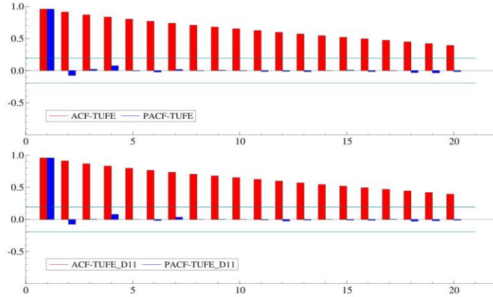
Şekil 7. Mevsimsellikten Arındırılmış ve Arındırılmamış TUF E Serisinin ACF ve PACF Grafikleri
