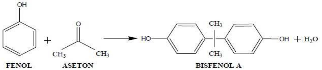
Şekil 3.1. Bisfenol-A'nın fenol ve asetonla kondensasyonu [ 14 ].
