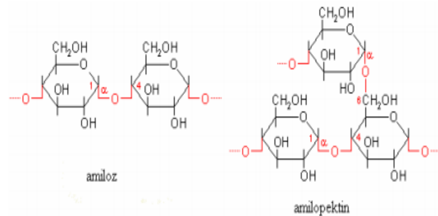
Şekil 2.2. Amilozun yapısı ve Amilopektinin yapısı
