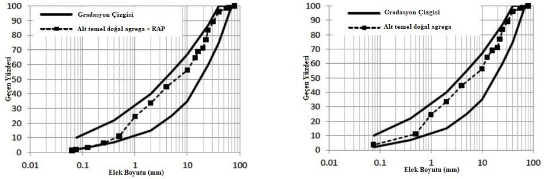
Şekil 2.6. Doğal agrega ve % 50 RAP içeren alt temelin granülometri eğrisi [65].
