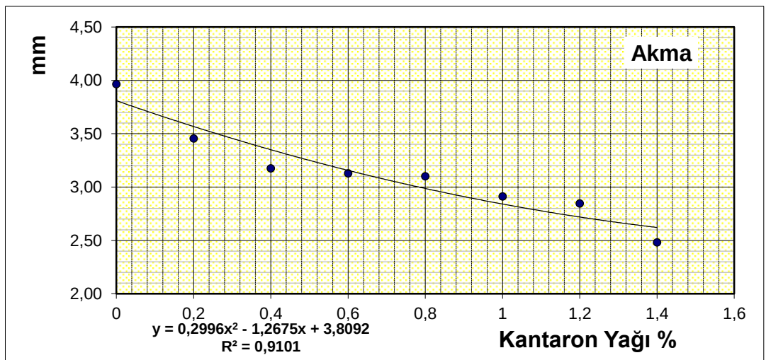
Şekil 4.24. Akmanın bitüm yüzdesi ile değişimi.
