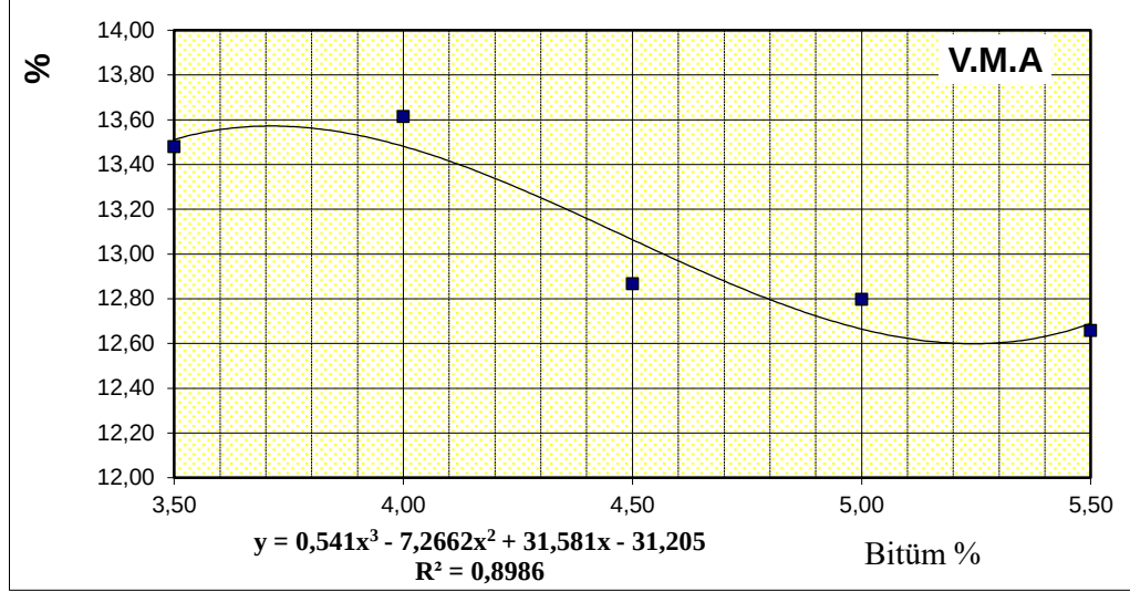
Şekil 4.5. VMA'nın bitüm yüzdesi ile değişimi.
