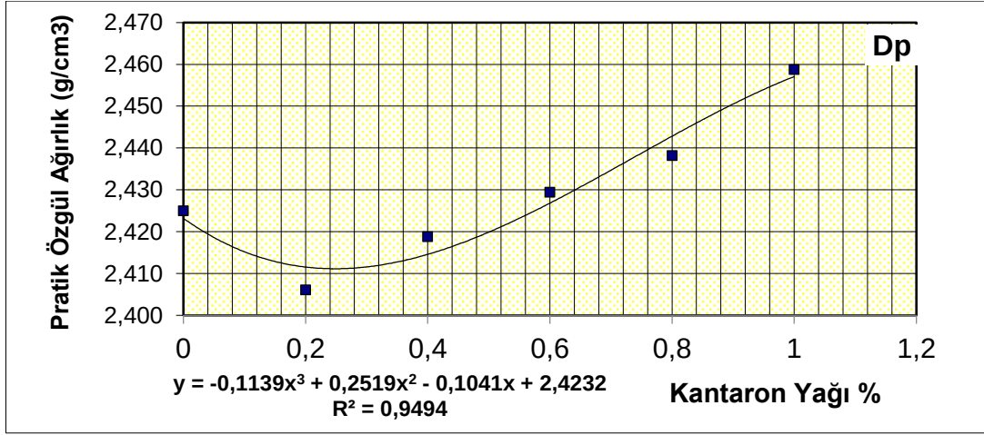
Şekil 4.13. Pratik özgül ağırlığın bitüm yüzdesi ile değişimi.
