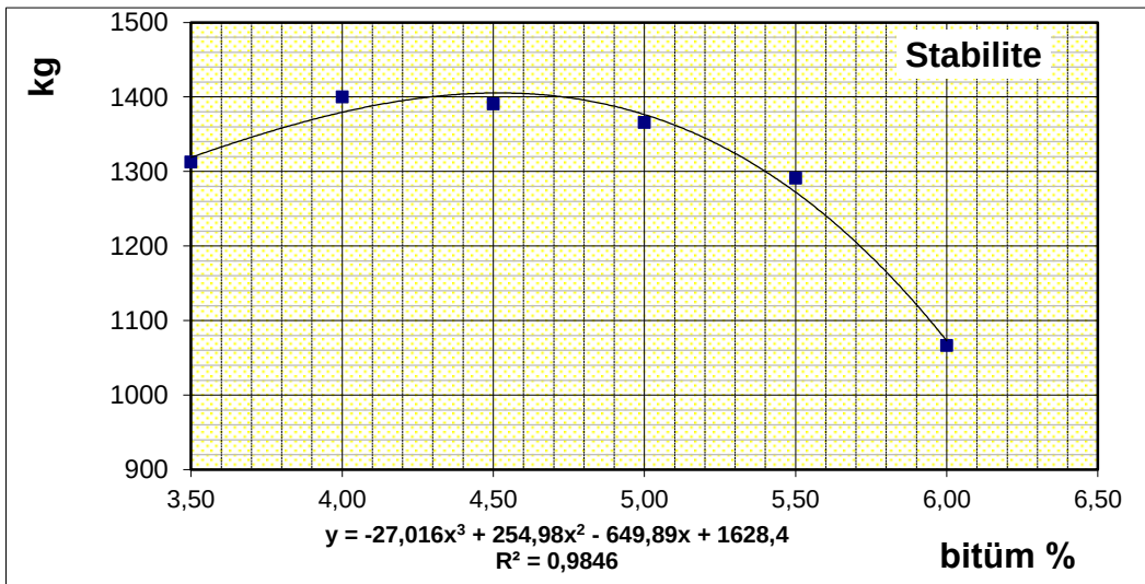
Şekil 4.4. Stabilitenin bitüm yüzdesi ile değişimi.
