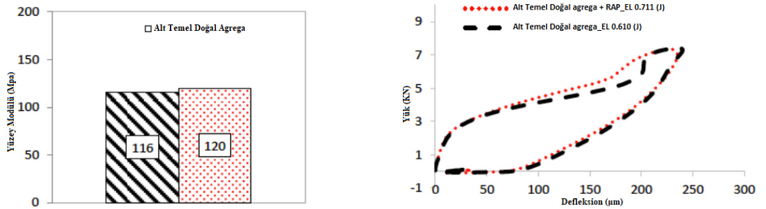
Şekil 2.7. LWD sonuçları [65].
