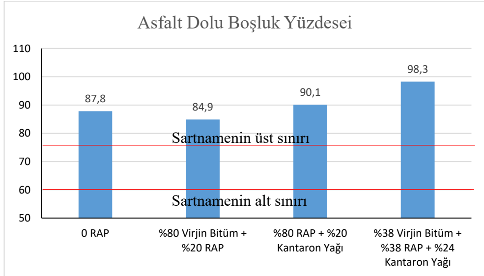
Şekil 4.26. Karşılaştırılmalı asfalt dolu boşluk yüzdesi değerleri.
