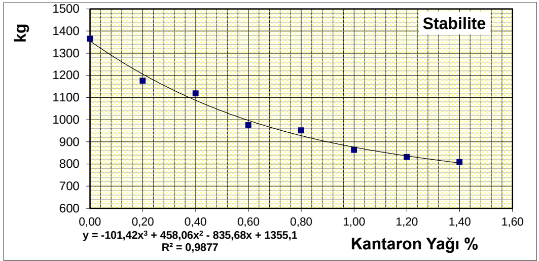
Şekil 4.22. Stabilitenin bitüm yüzdesi ile değişimi.
