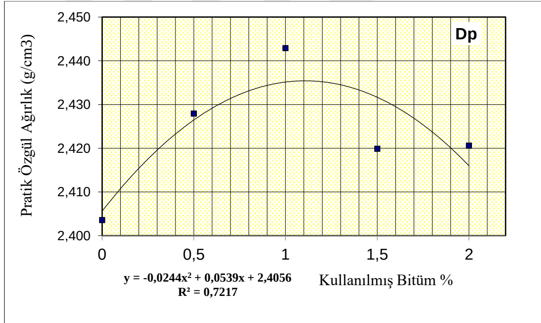
Şekil 4.7. Pratik özgül ağırlığın bitüm yüzdesi ile değişimi.
