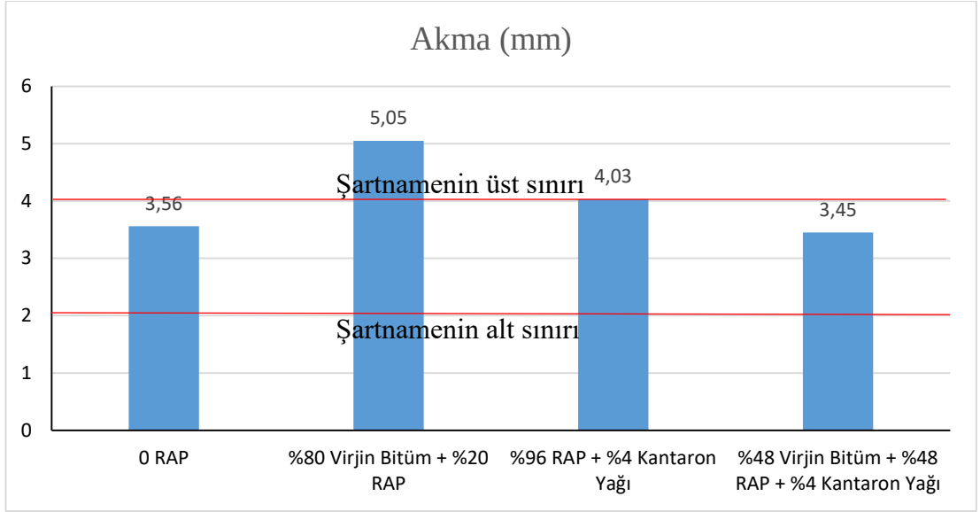
Şekil 4.30. Karşılaştırılmalı akma değerleri.
