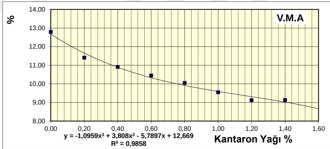
Şekil 4.23. VMA'nın bitüm yüzdesi ile değişimi.
