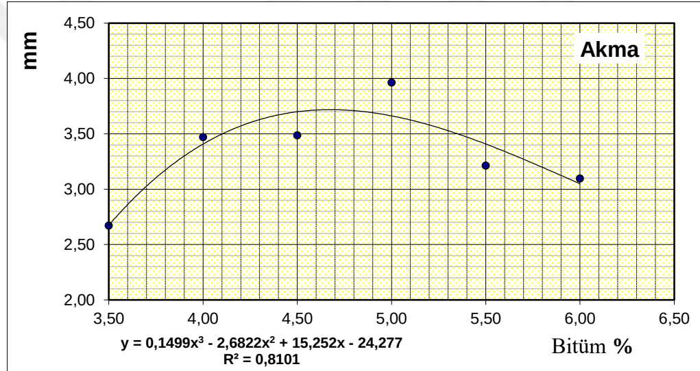
Şekil 4.6. Akmanın bitüm yüzdesi ile değişimi.
