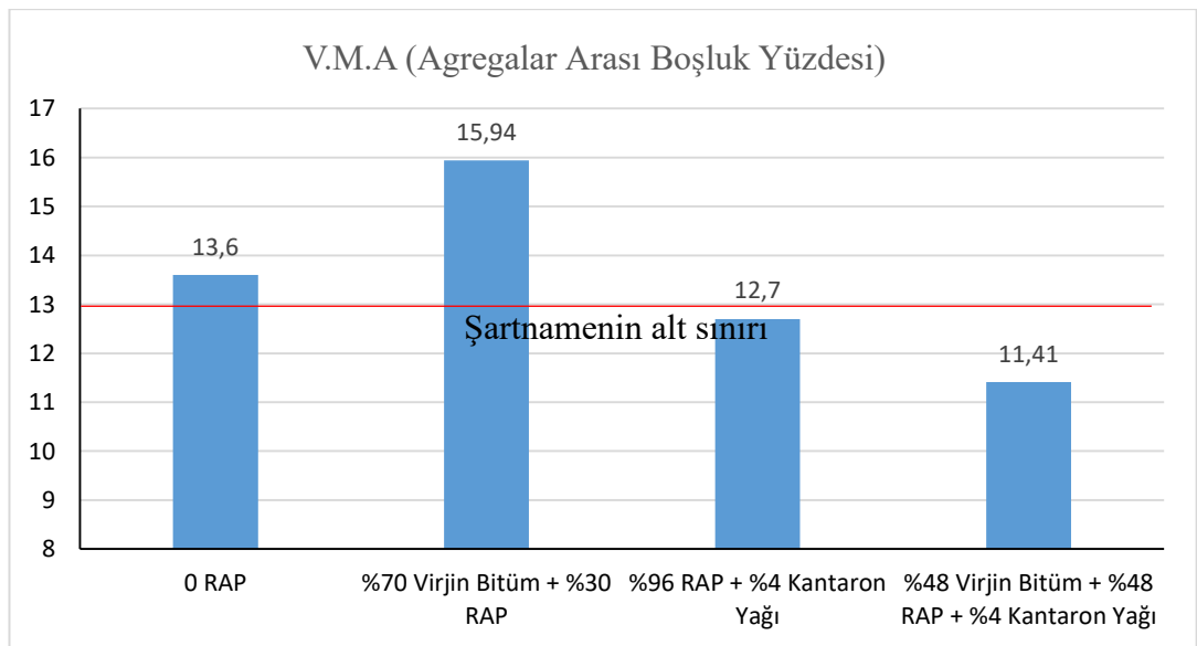
Şekil 4.28. Karşılaştırılmalı V.M.A değerleri
