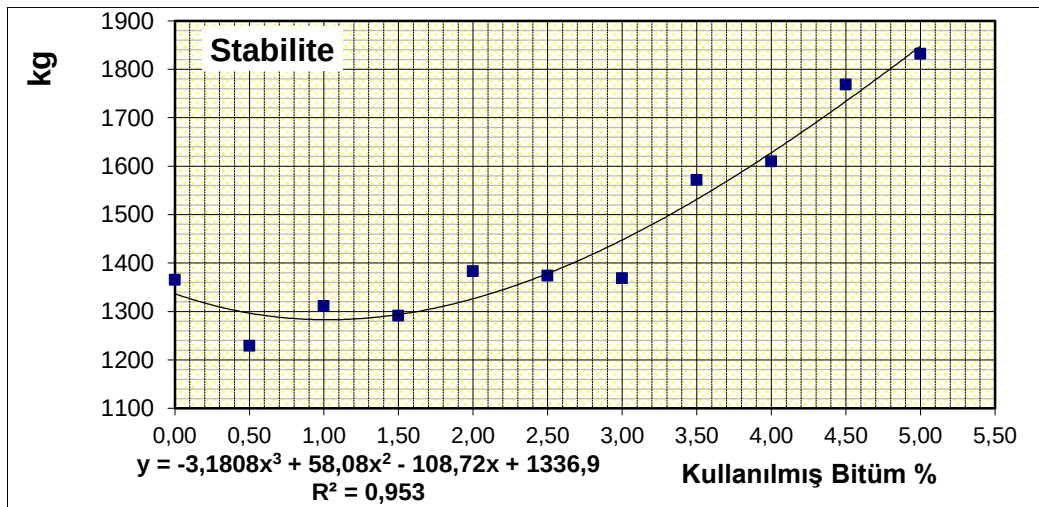
Şekil 4.10. Stabilitenin bitüm yüzdesi ile değişimi.
