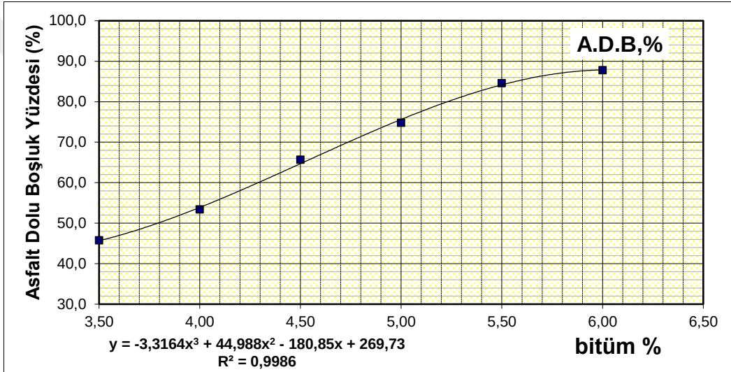
Şekil 4.3. Asfalt dolu boşluk yüzdesinin bitüm yüzdesi ile değişimi.
