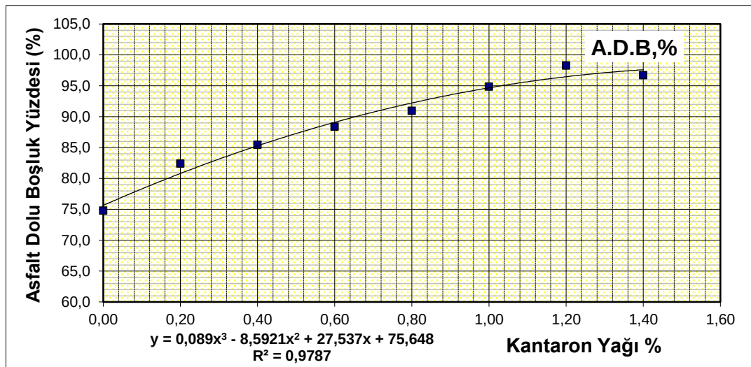
Şekil 4.21. Asfalt dolu boşluk yüzdesinin bitüm yüzdesi ile değişimi.
