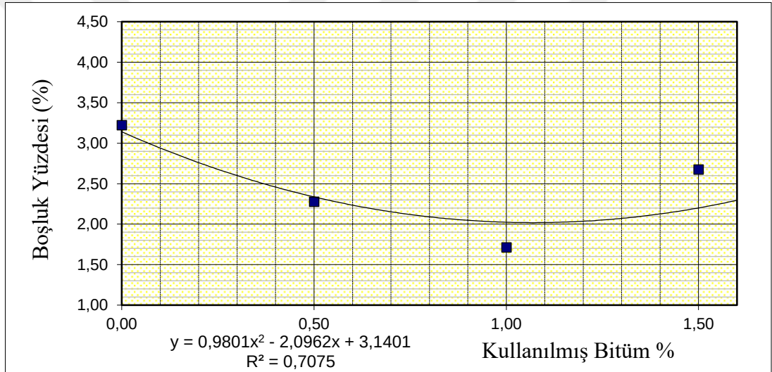
Şekil 4.9. Boşluk yüzdesinin bitüm yüzdesi ile değişimi.
