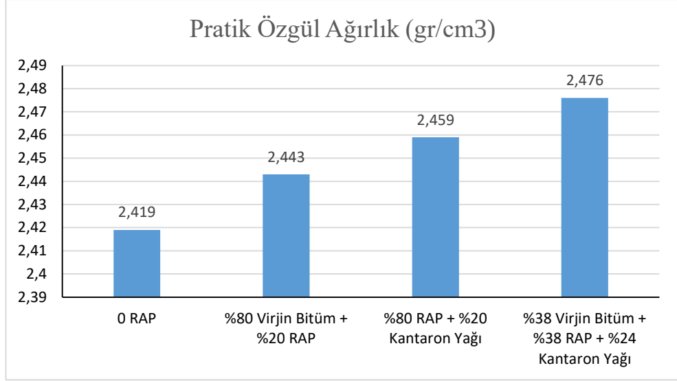
Şekil 4.25. Karşılaştırılmalı pratik özgül ağırlık ( D_p ) değerleri.
