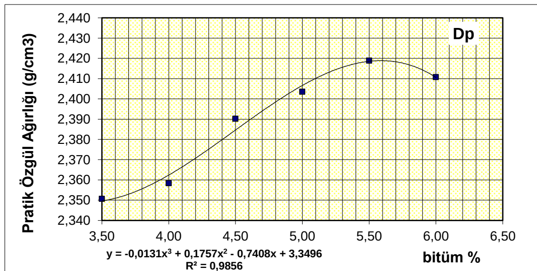
Şekil 4.1. Pratik özgül ağırlığın bitüm yüzdesi ile değişimi.
