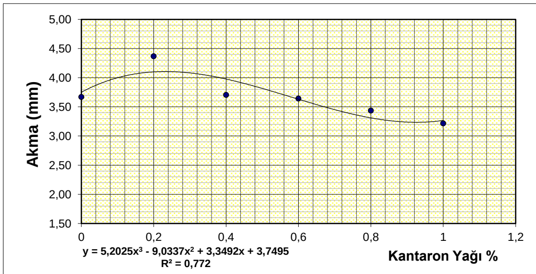
Şekil 4.18. Akmanın bitüm yüzdesi ile değişimi.
