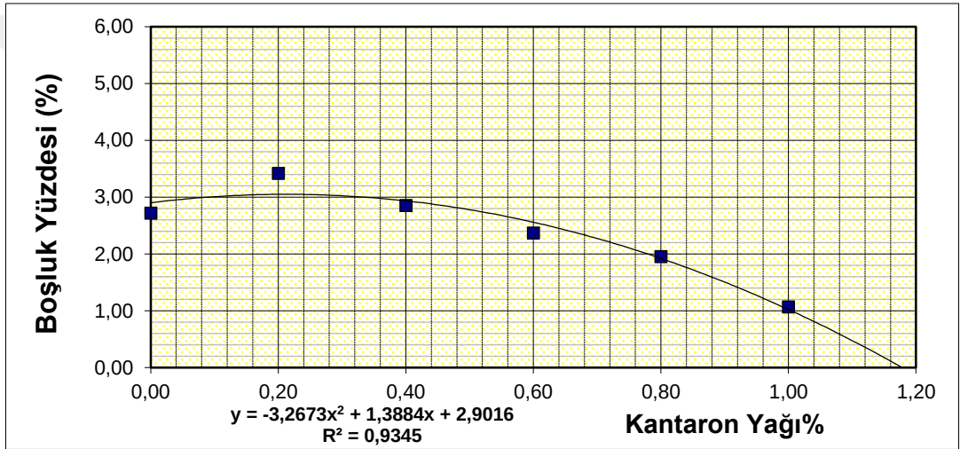
Şekil 4.14. Boşluk yüzdesinin bitüm yüzdesi ile değişimi.
