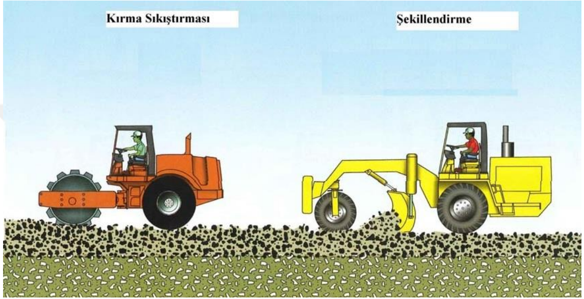
Şekil 1.14. Tam derinlikli geri dönüşümün kırma sıkıştırma ve şekillendirme [42].
