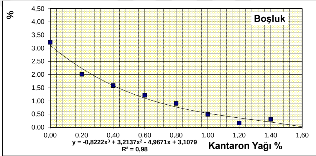
Şekil 4.20. Boşluk yüzdesinin bitüm yüzdesi ile değişimi.
