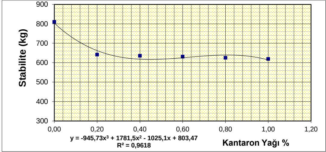
Şekil 4.16. Stabilitenin bitüm yüzdesi ile değişimi.
