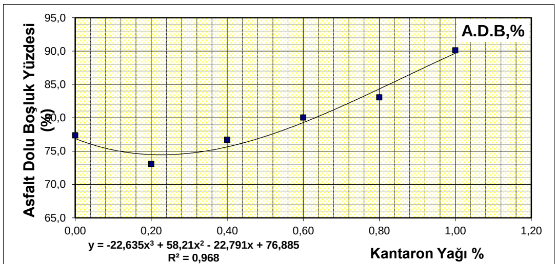
Şekil 4.15. Asfalt dolu boşluk yüzdesinin bitüm yüzdesi ile değişimi.
