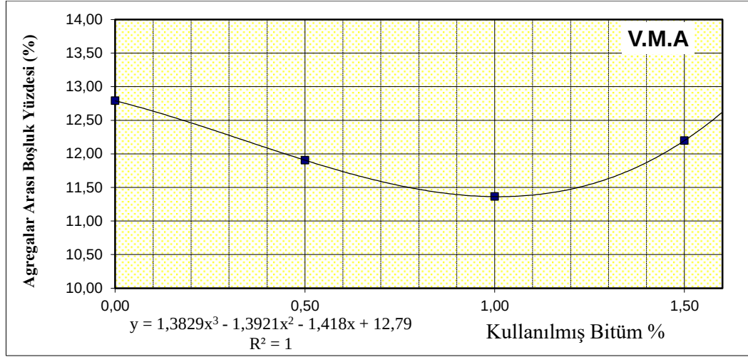
Şekil 4.11. VMA'nın bitüm yüzdesi ile değişimi.
