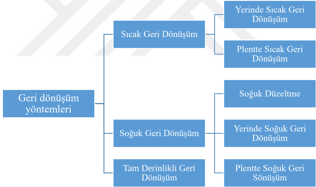
Çizelge 1.1. Geri dönüşüm yöntemleri.
