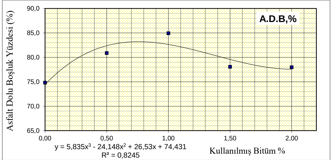
Şekil 4.8. Asfalt dolu boşluk yüzdesinin bitüm yüzdesi ile değişimi.
