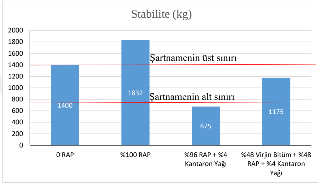
Şekil 4.29. Karşılaştırılmalı stabilite değerleri.
