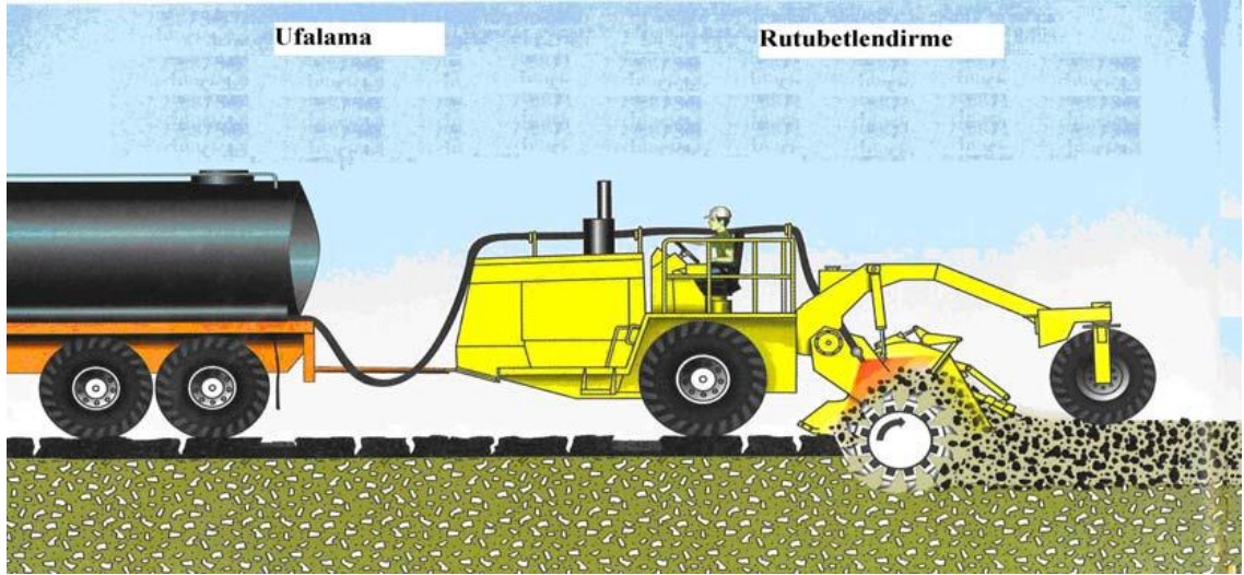
Şekil 1.13. Tam derinlikli geri dönüşümün ufalanma ve rutubetlendirme [42].
