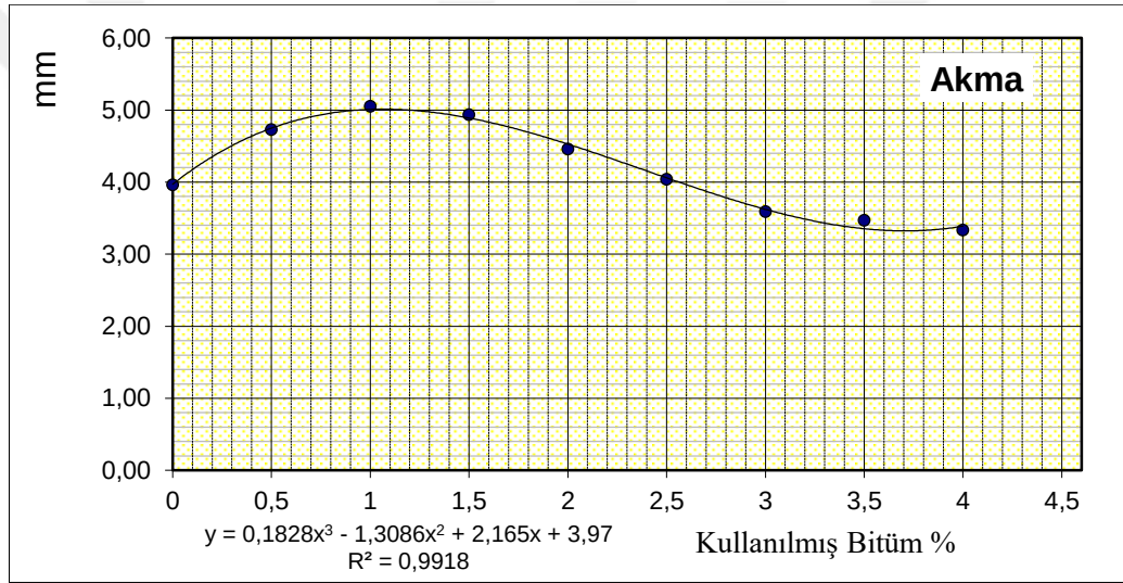
Şekil 4.12. Akmanın bitüm yüzdesi ile değişimi.
