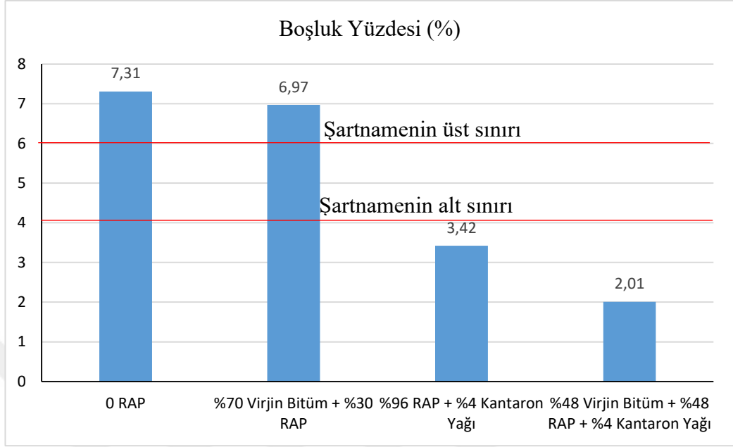
Şekil 4.27. Karşılaştırılmalı boşluk yüzdesi değerleri.
