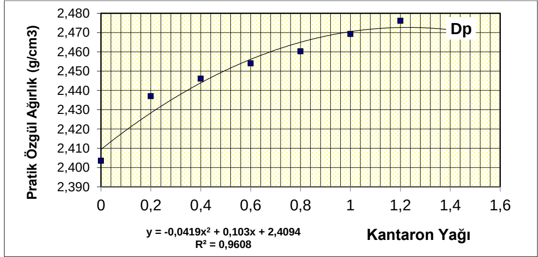
Şekil 4.19. Pratik özgül ağırlığın bitüm yüzdesi ile değişimi.
