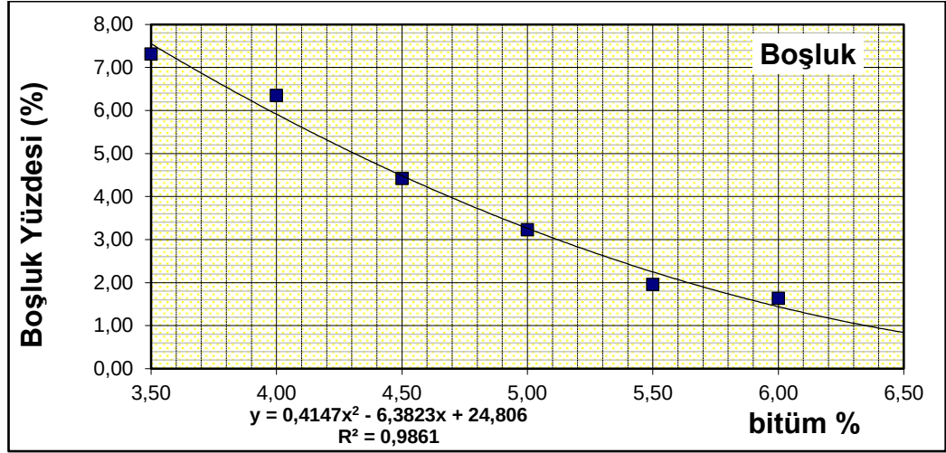
Şekil 4.2. Boşluk yüzdesinin bitüm yüzdesi ile değişimi.
