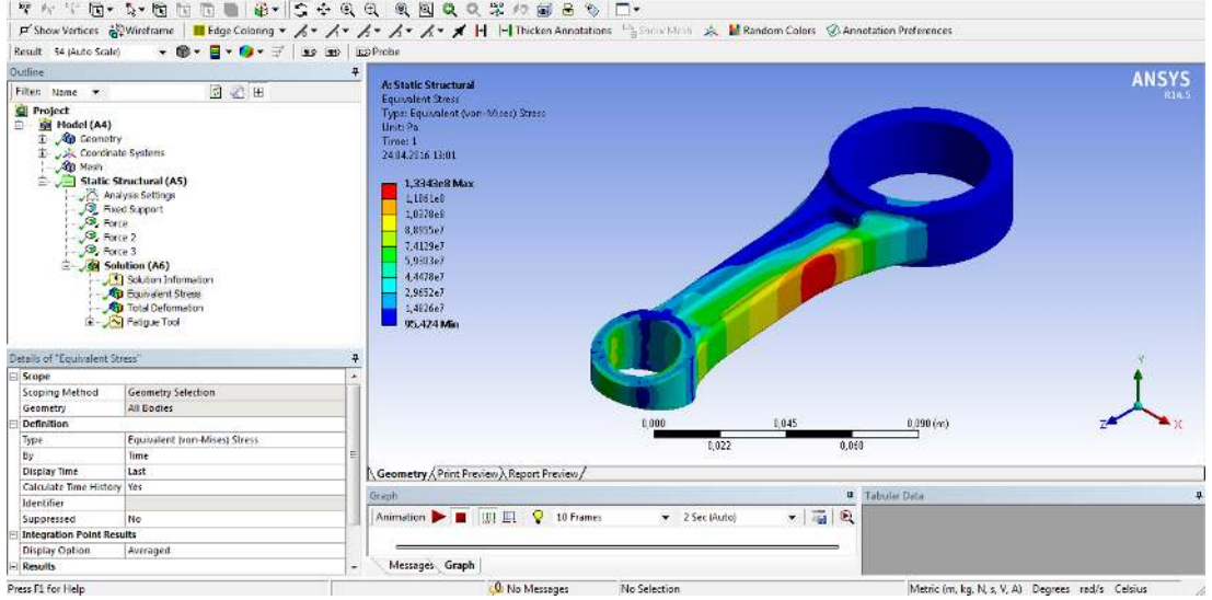
Şekil 7.10 Statik analiz sonrası oluşan maksimum eşdeğer gerilmeler
