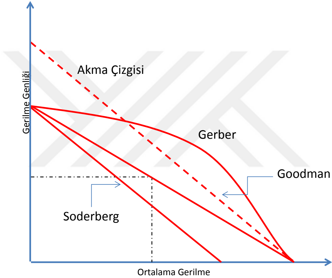
Şekil 3.5 Soderberg, Goodman, Gerber eğrileri [21]
