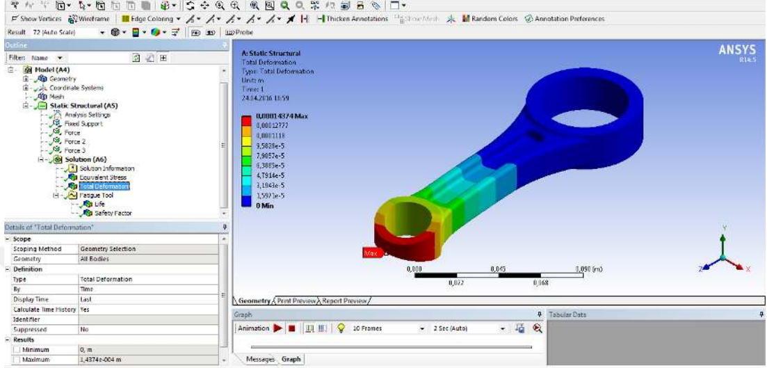
Şekil 7.17 Optimizasyon sonrası oluşan tasarımın maksimum yer değıştirmesi
