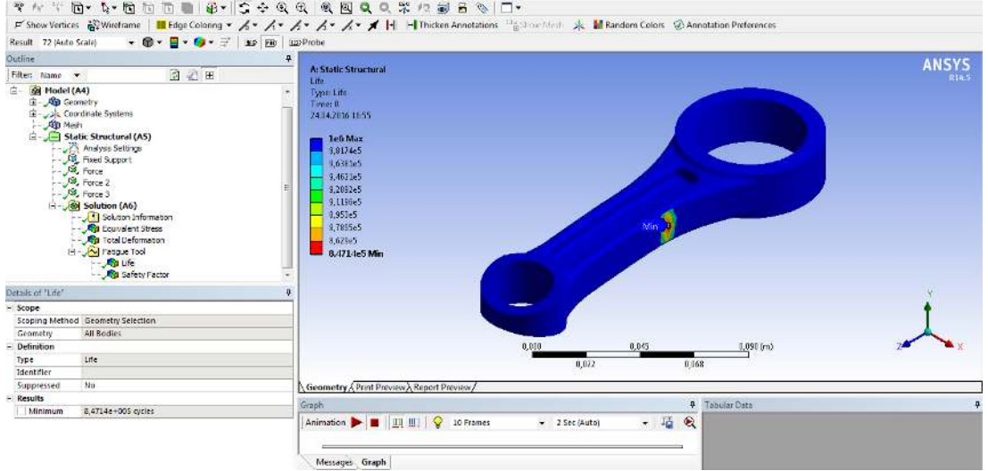
Şekil 7.19 Optimizasyon sonrası oluşan tasarımın ömür dayanımı
