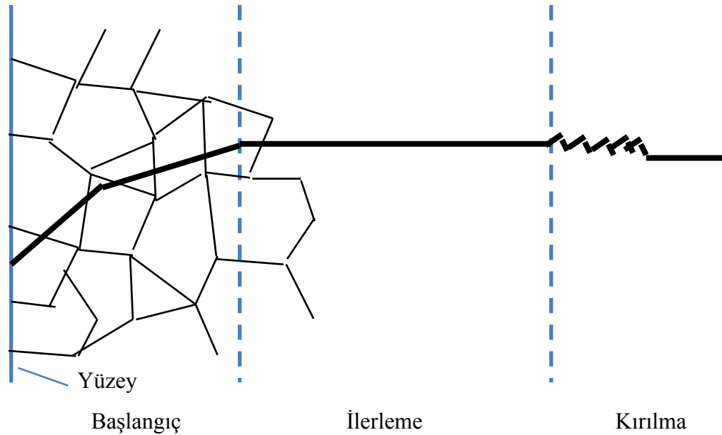
Şekil 3.6 Yorulma kırılmasının üç aşaması [24]
