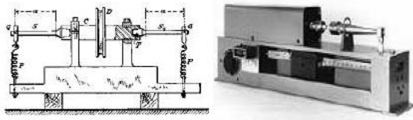
Şekil 3.1 1850'lerde geliştirilen Wöhler (a) ve 2000'li yıllarda kullanılan (b) yorulma test düzenekleri [15]
