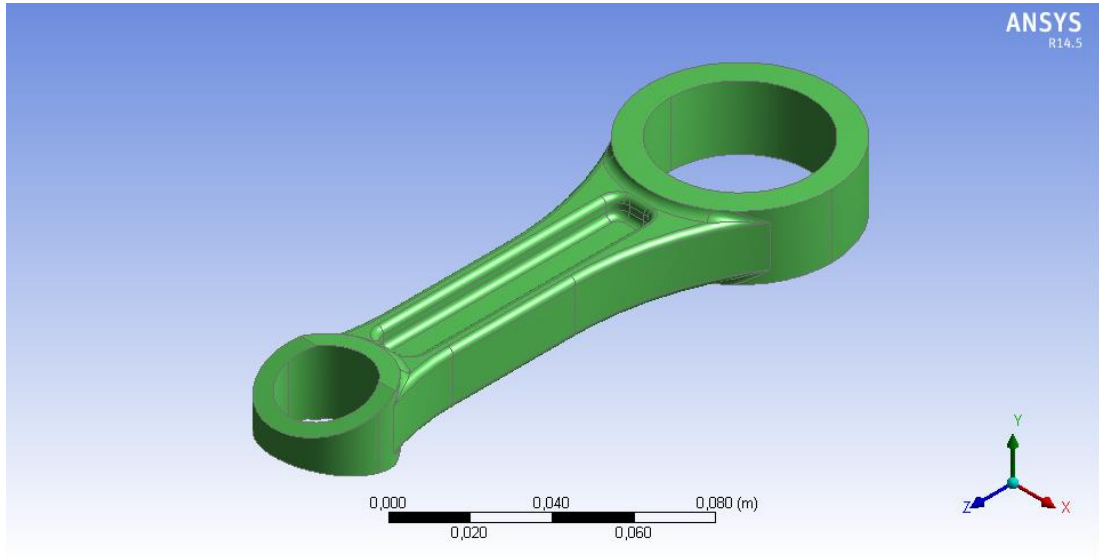
Şekil 7.16 Optimizasyon sonrası belirlenen değişkenlerle oluşan tasarım
