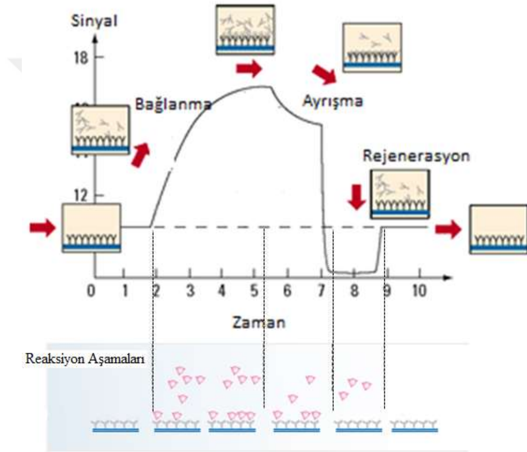
Şekil 2.14. Reaksiyon aşamalarının RIfS yüzeyindeki değişiklikleri ve sensogramdaki karşılığı
