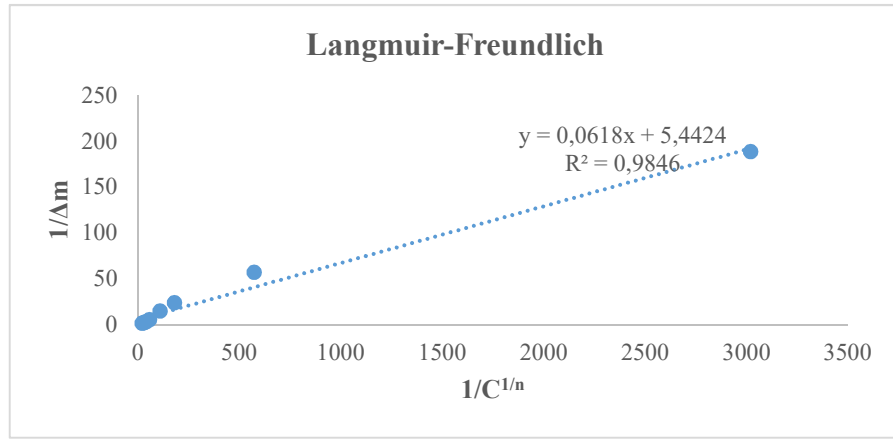
Şekil 4.31. ZnO nanolifi için Langmuir-Freundlich izotermi
