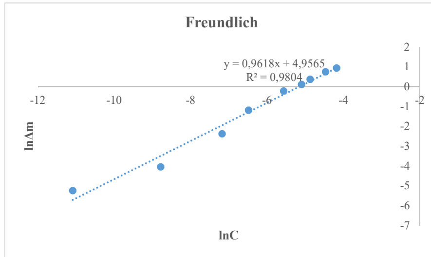
Şekil 4.33. ZnO-APBA nanolifi için Freundlich izotermi
