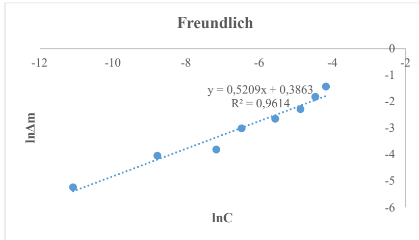
Şekil 4.24. CuO nanolifi için Freundlich izotermi
