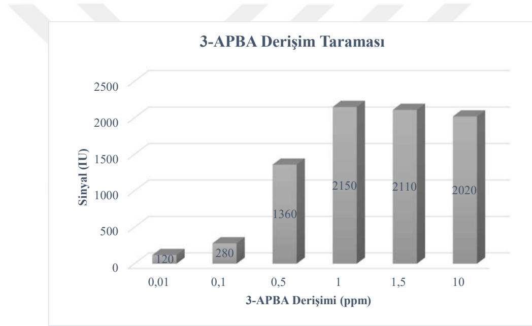
Şekil 4.47. 3-APBA için derişim taraması
