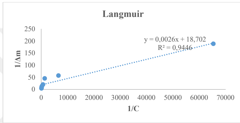
Şekil 4.23. CuO nanolifi için Langmuir izotermi
