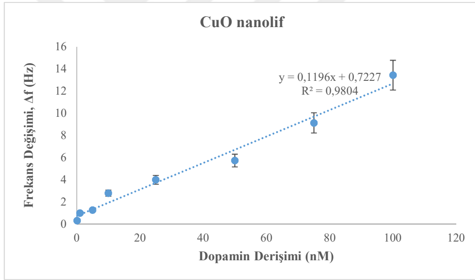
Şekil 4.19. QCM sensörde ZnO içeren nanolifin dopamin çözeltilerine ait kalibrasyon grafiğı
