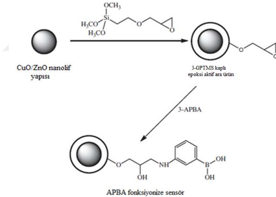
Şekil 3.2. Nanoliflerin modifikasyon şeması
