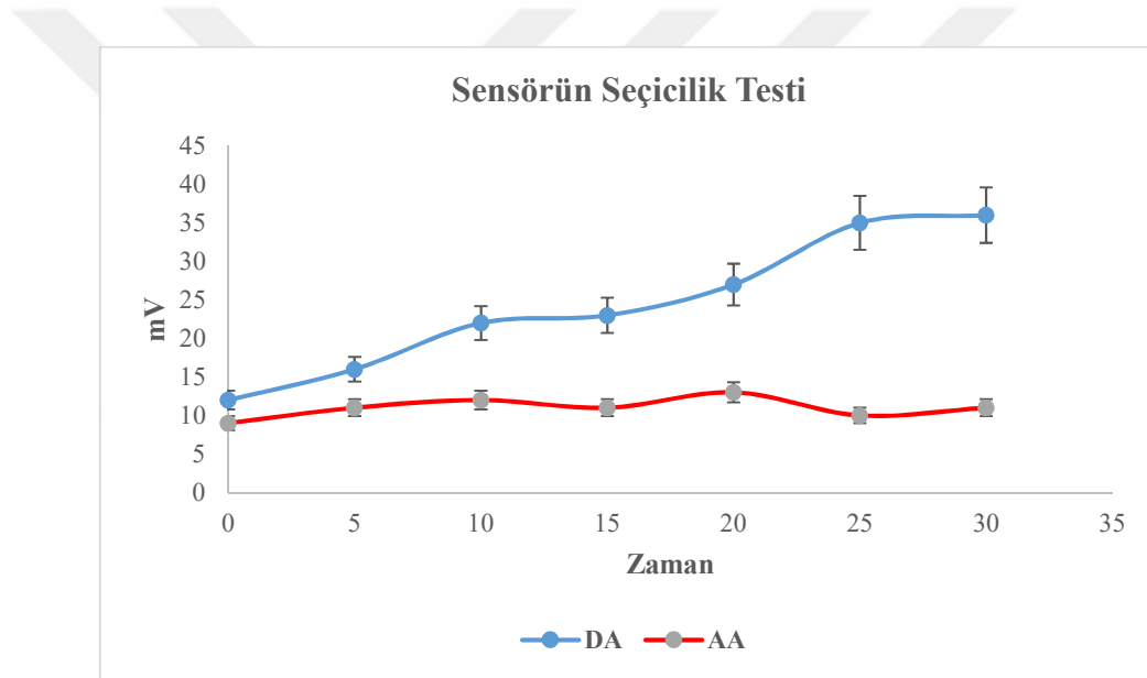
Şekil 4.46. Potansiyometrik sensörün seçicilik testi
