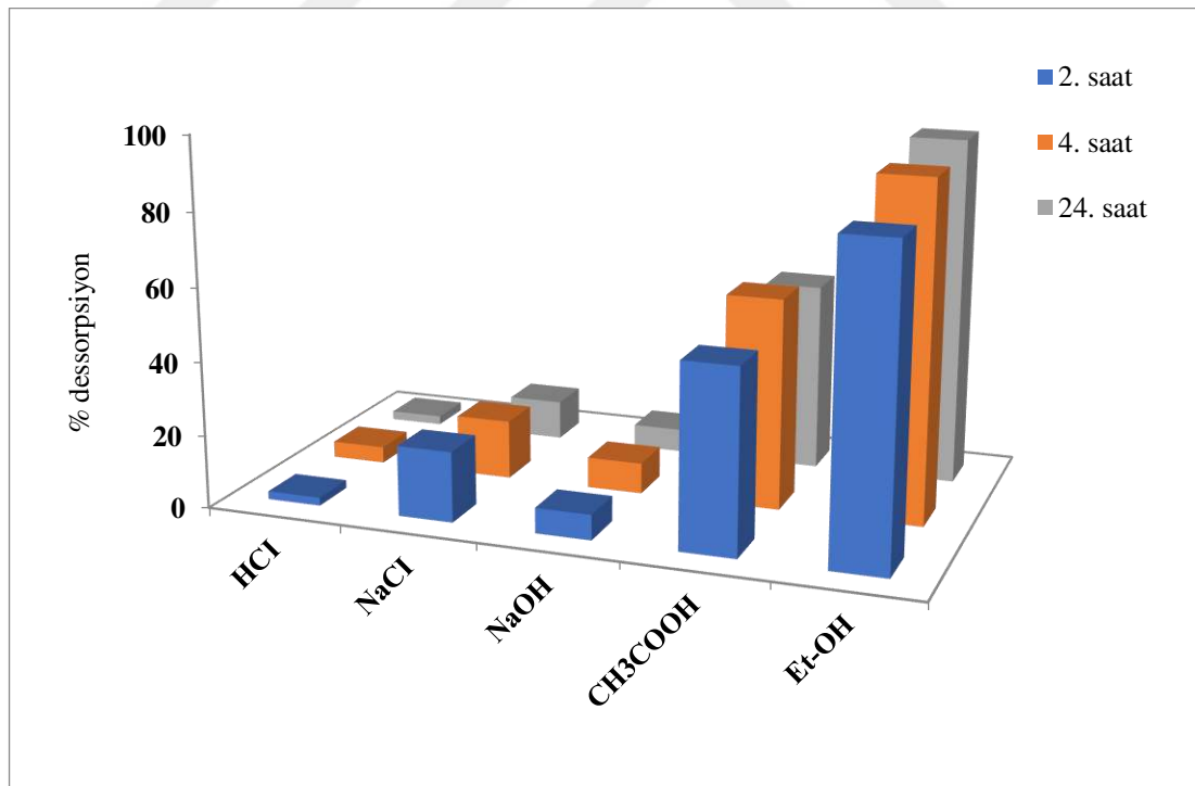
Şekil 4.17 Desorpsiyon çalışması garfiği
