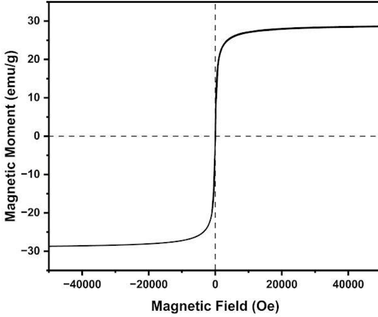
Şekil 4.7 Z-MNP için VSM manyetizasyon eğrisi
