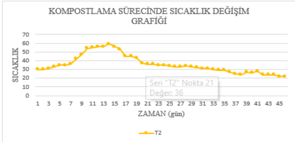
Şekil 4.19. Kompostlama sırasında T2 grubunun sıcaklık değişimi.
