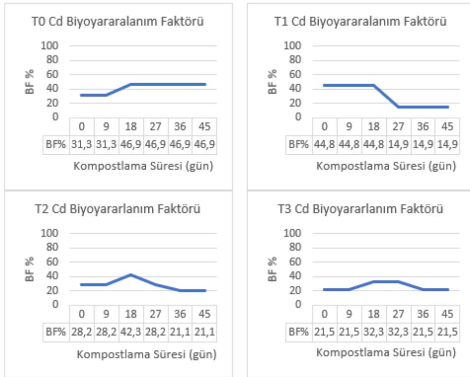
Şekil 4.47. Kompostlama sürecinde Cd fraksiyonlarındaki biyoyararlanım faktörü değişimler.
