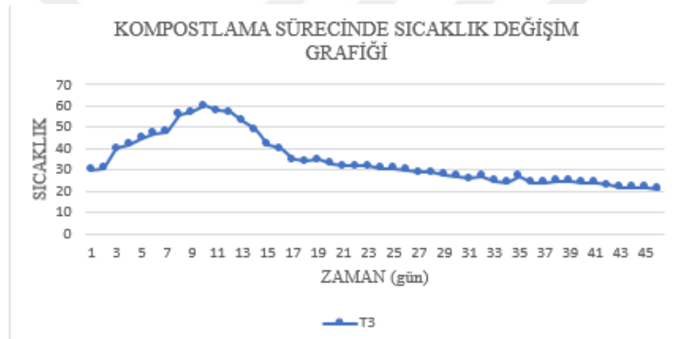
Şekil 4.20. Kompostlama sırasında T3 grubunun sıcaklık değişimi.
