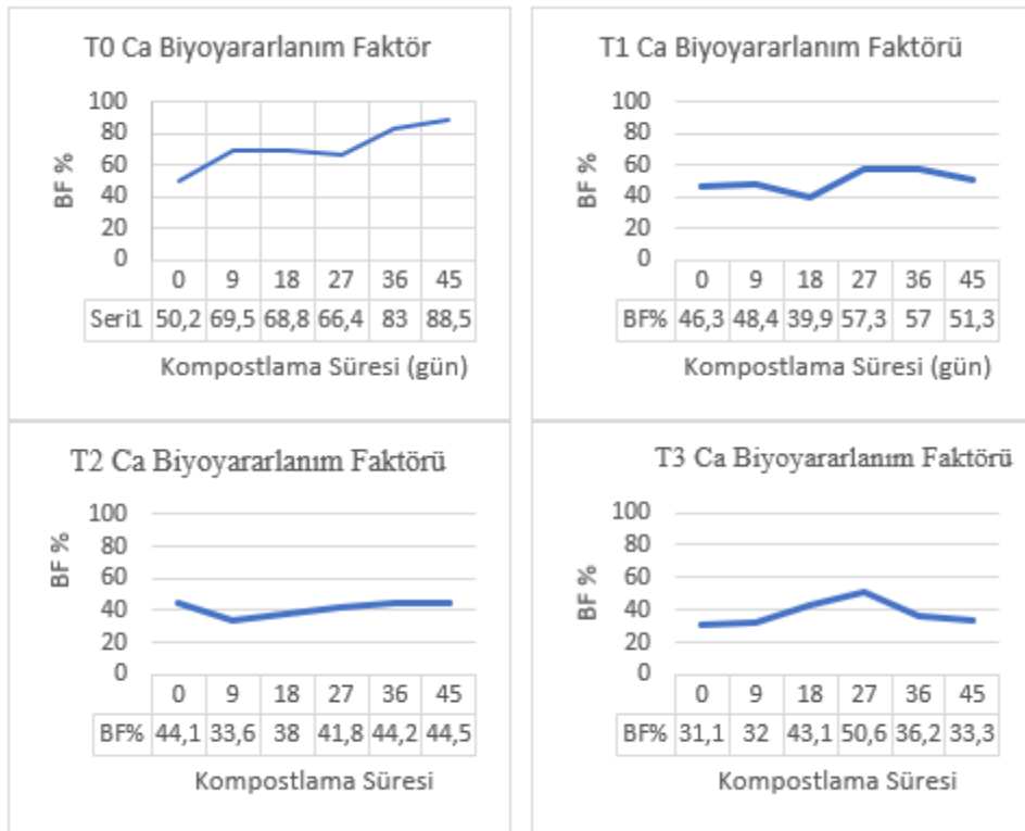
Şekil 4.37. Kompostlama sürecinde Ca fraksiyonlarındaki Biyoyararlanım faktörü değişimler.
