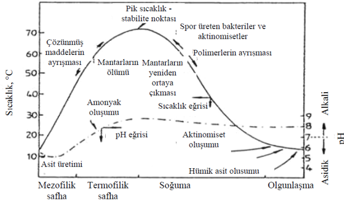
Şekil 2.4. Kompostlaştırma sürecinde zamana karşı sıcaklık ve pH değişim grafiği. (Öztürk ve ark., (2016).
