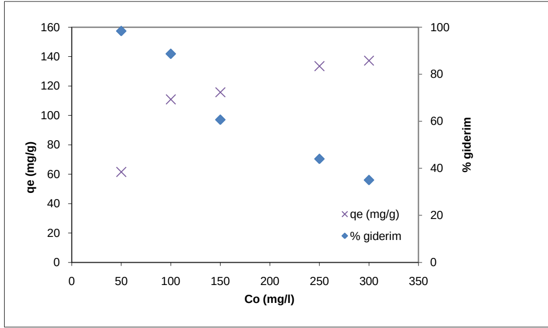
Şekil 7.1. Pb^{+2} iyonu adsorpsiyonu için 50 °C’de, farklı başlangıç derişimlerinde adsorpsiyon kapasitesinin ve % giderim veriminin değışimi (0,8 g/l karbon derişimi)
