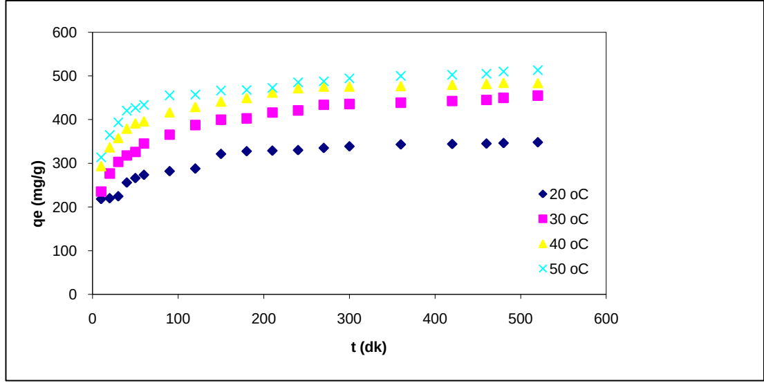
Şekil 7.7. BT adsorpsiyonu için 350 mg/l başlangıç derişiminde adsorpsiyon kapasitesinin zamana ve sıcaklığa bağlı olarak değişimi (0,4 g/l aktif karbon derişimi)
