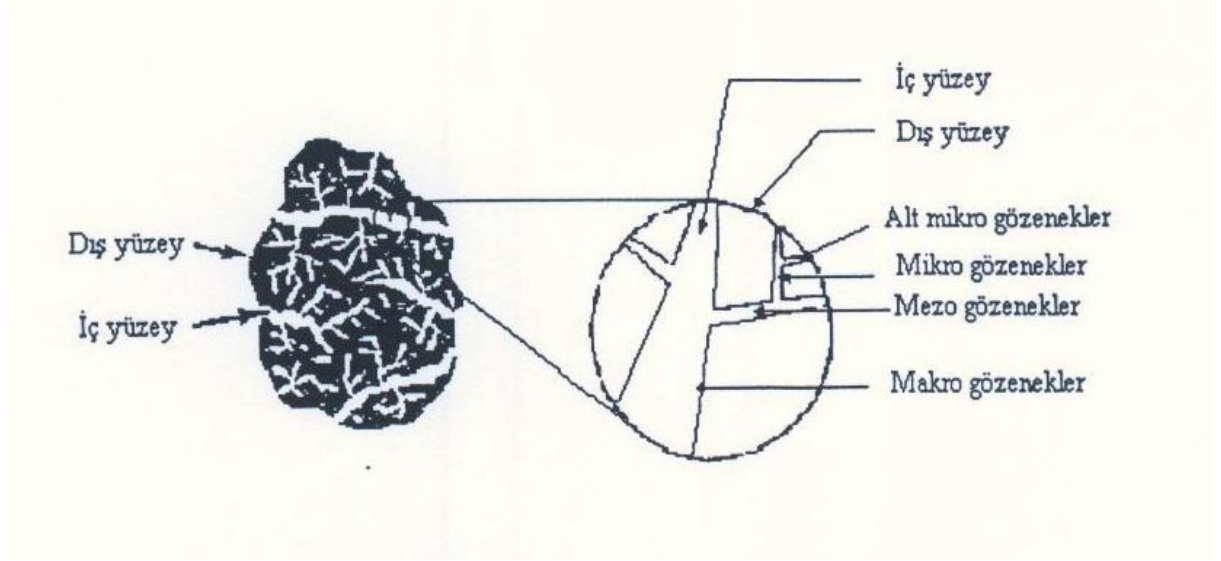
Şekil 4.6. Aktif karbonun gözenek yapısı [47]
