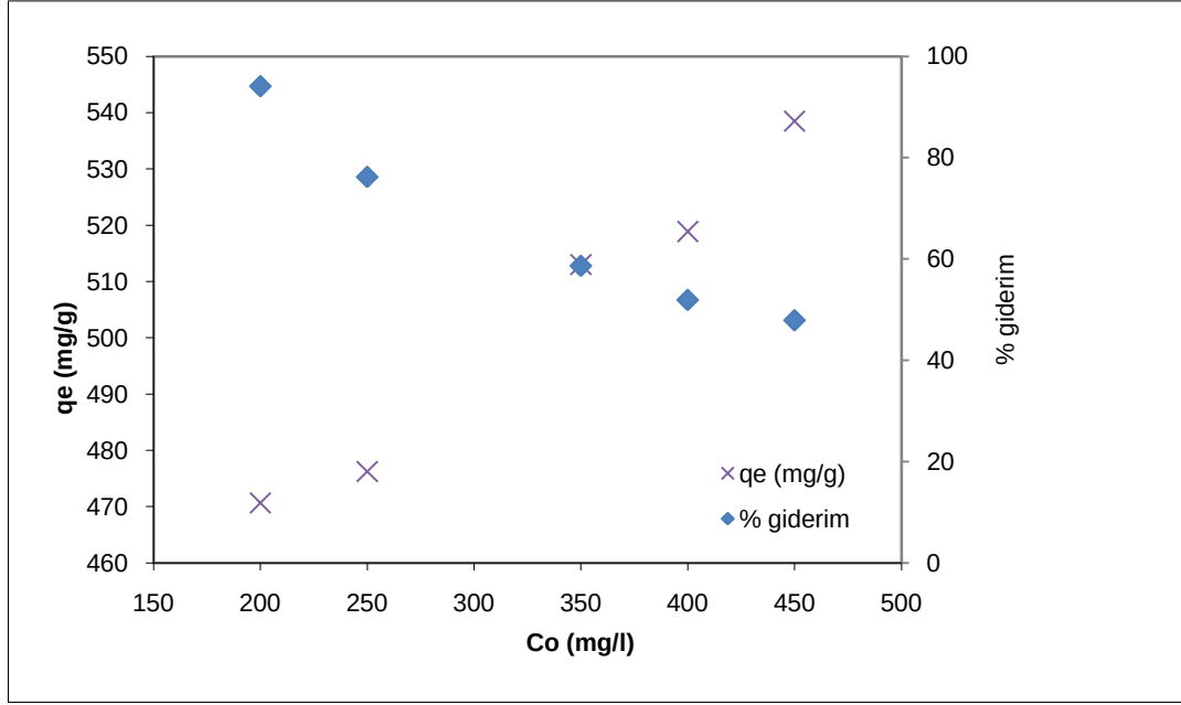
Şekil 7.6. BT adsorpsiyonu için 50 °C’de, farklı başlangıç derişimlerinde adsorpsiyon kapasitesinin ve % giderim veriminin değışimi (0,4 g/l aktif karbon derişimi)
