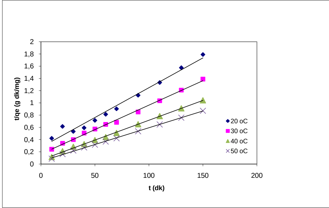
Şekil 7.5. 200 mg/l derişime sahip Pb +2 iyonu adsorpsiyonu için sözde ikinci mertbe kinetik modeline göre elde edilen grafik
