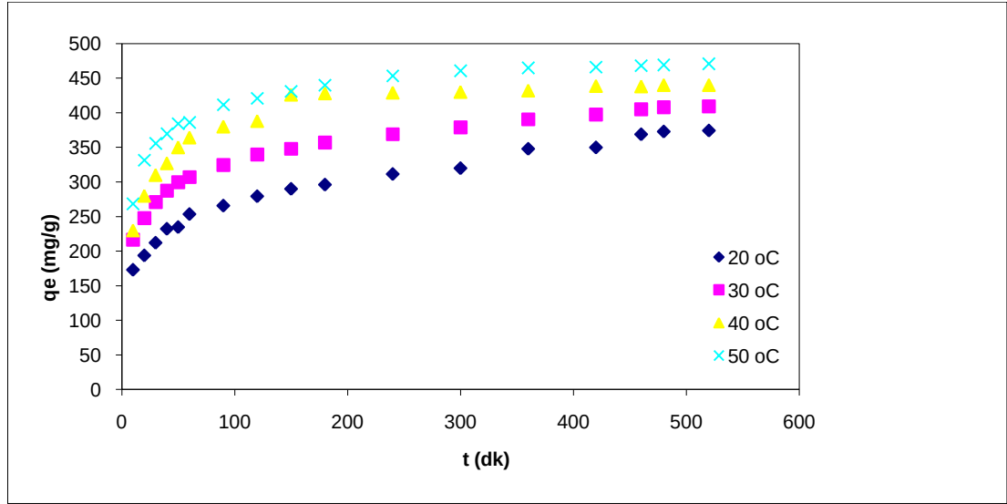
Şekil 7.8. BT adsorpsiyonu için 200 mg/l başlangıç derişiminde adsorpsiyon kapasitesinin zamana ve sıcaklığa bağlı olarak değişimi (0,4 g/l aktif karbon derişimi)
