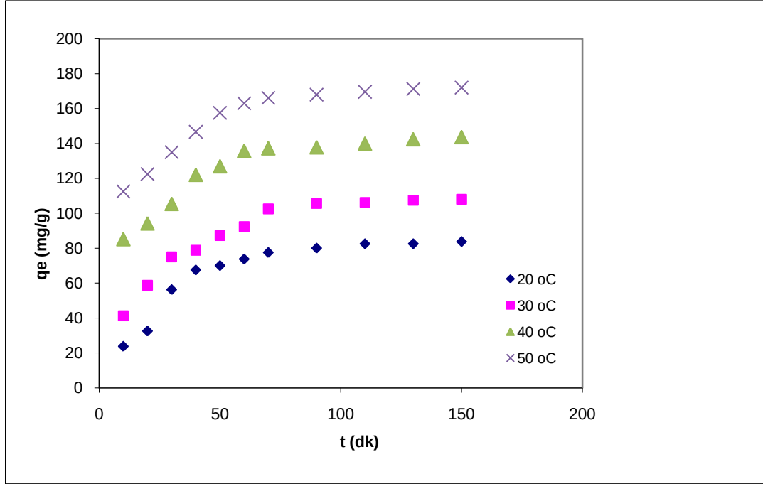
Şekil 7.2. Pb 2+ iyonu adsorpsiyonu için 200 mg/l başlangıç derişiminde adsorpsiyon kapasitesinin zamana ve sıcaklığa bağlı olarak değışimi (0,8 g/l karbon derişimi)
