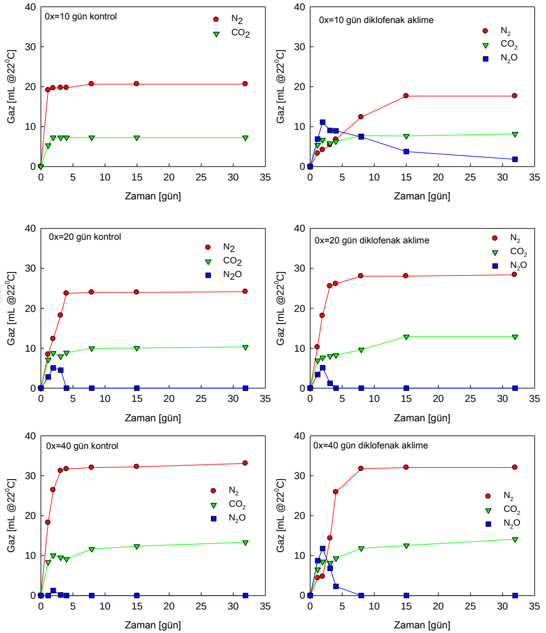
Şekil 4.21 : Kontrol ve Diklofenak’a aklime olan ve çamur yaşları 10 gün; 20 gün ve 40 gün olarak işletilen reaktörlerde gözlenen gaz üretim profilleri.
