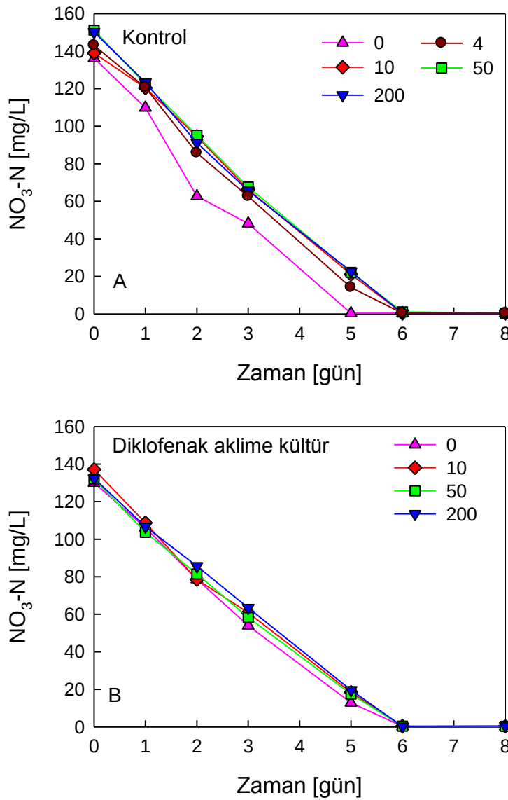
Şekil 4.14 : Başlangıç Diklofenak konsantrasyonunun Kontrol kültüründe (A) ve Diklofenak'a aklime olmuş kültürde (B) denitrifikasyona etkisi.
