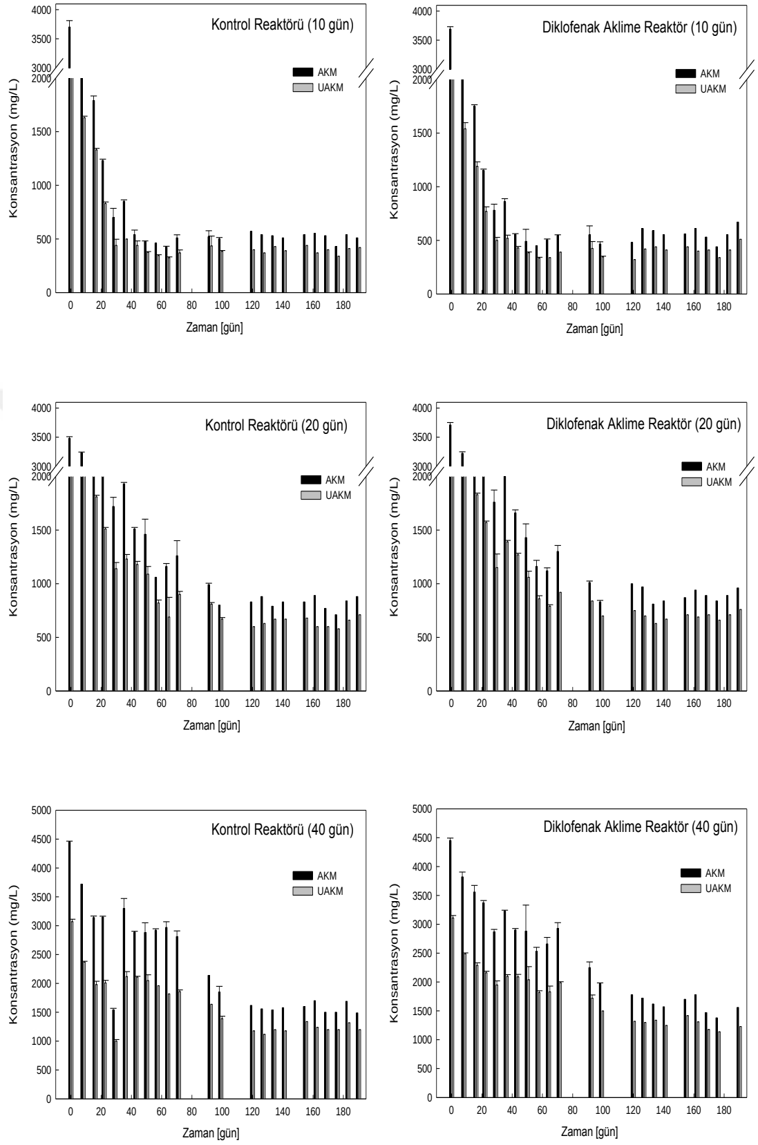
Şekil 4.10 : Farklı çamur yaşlarında işletilen anoksik reaktörlerde AKM ve UAKM profilleri.
