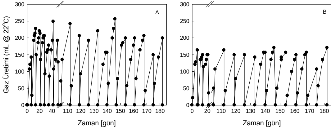
Şekil 4.8 : Denitrifikasyon yapan kontrol reaktörü (A) ve Diklofenak'a aklimasyon yapılan reaktörde (B) gaz üretim profilleri.
