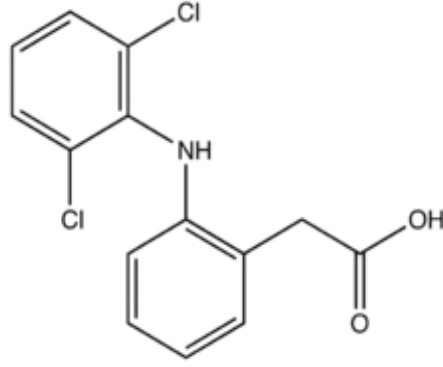
Şekil 2.1 : Diklofenak'ın kimyasal yapısı.
