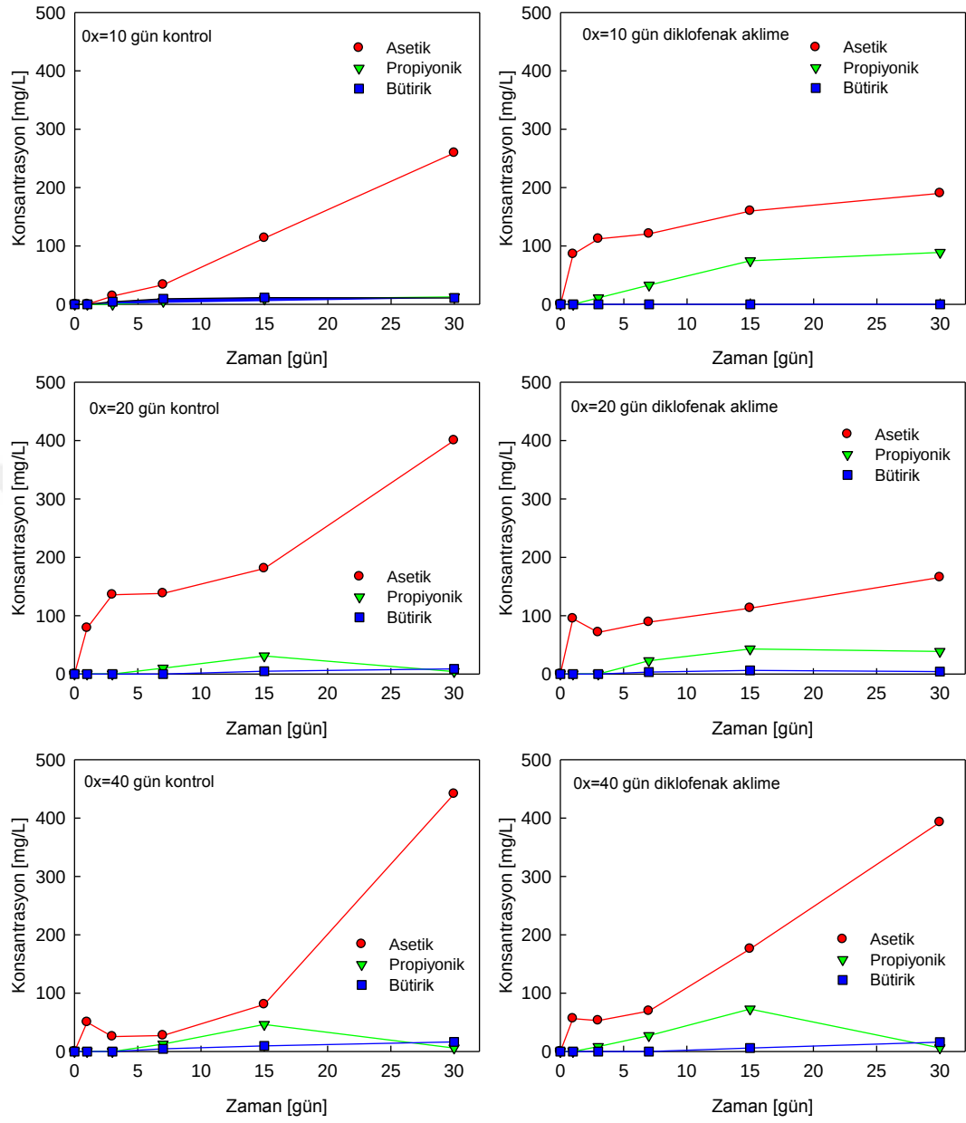
Şekil 4.23 : Kontrol ve Diklofenak’a aklime olan ve çamur yaşları 10 gün; 20 gün ve 40 gün olarak işletilen anoksik reaktörlerde gözlenen UYA değişimleri.
