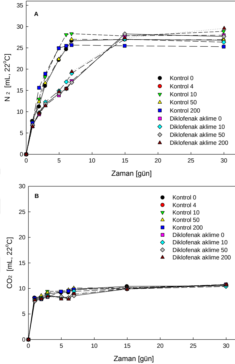
Şekil 4.17 : Kontrol reaktörü ve Diklofenak’a aklime olan kültürde farklı konsantrasyonlarda Diklofenak ilavesi sonucu gözlenen N 2 (A) ve CO 2 (B) üretim profilleri.
