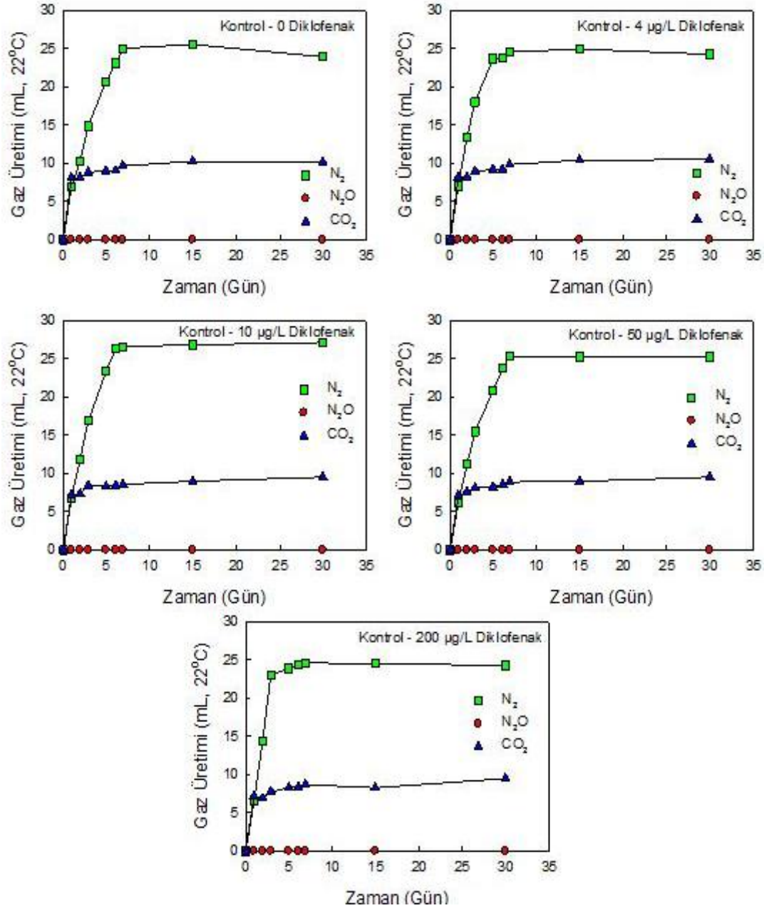
Şekil 4.15 : Denitrifikasyon yapan kontrol reaktöründe farklı konsantrasyonlarda Diklofenak ilavesi sonucu gözlenen gaz üretim profilleri.
