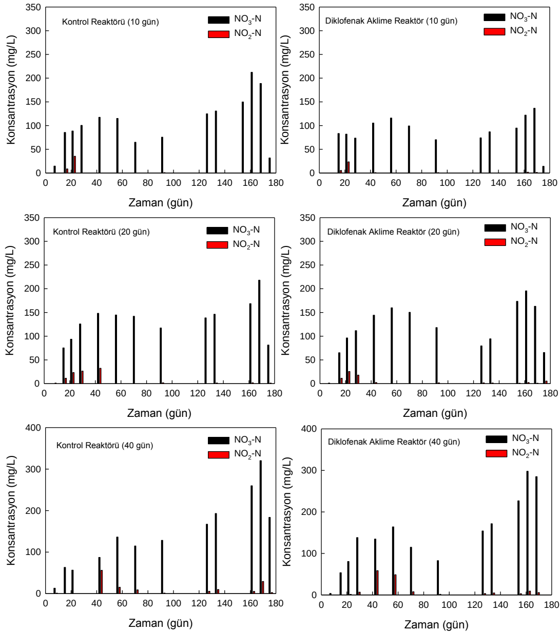
Şekil 4.12 : Farklı çamur yaşlarında işletilen anoksik reaktörlerde nitrit ve nitrat profilleri.
