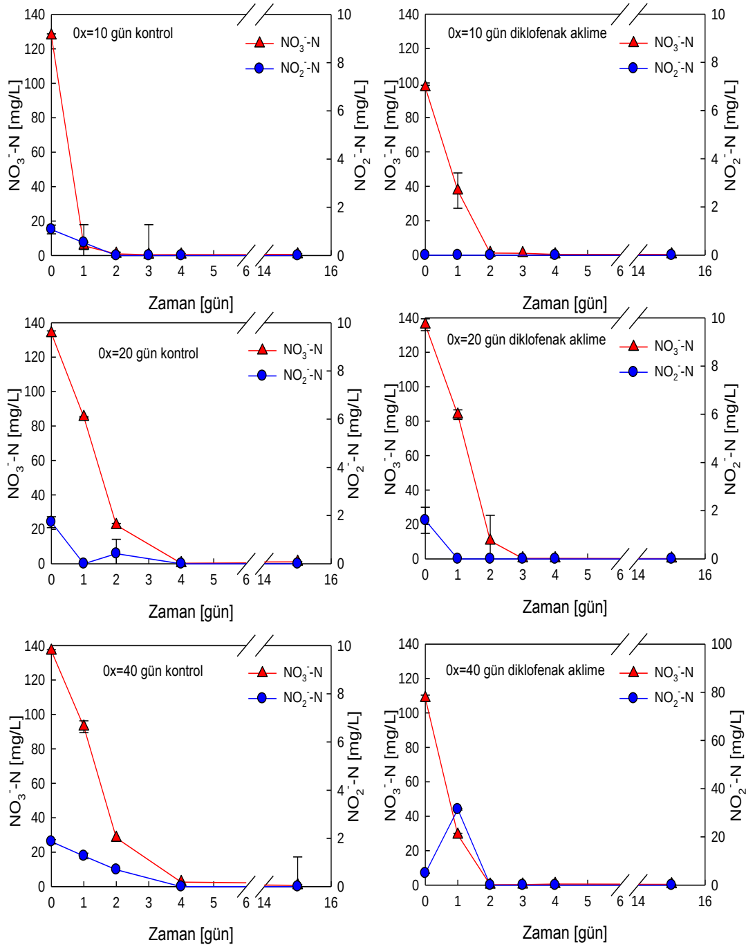
Şekil 4.20 : Kontrol ve Diklofenak'a aklime olan ve çamur yaşları 10 gün; 20 gün ve 40 gün olarak işletilen reaktörlerden alınan aşı ile kurulan reaktörde nitrat ve nitrit giderim profilleri.
