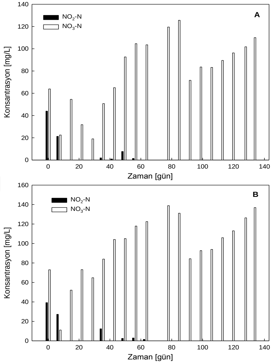
Şekil 4.7 : Denitrifikasyon yapan reaktörlerde nitrat ve nitrit profilleri; Kontrol reaktörü (A) ve Diklofenak'a aklime reaktör (B).
