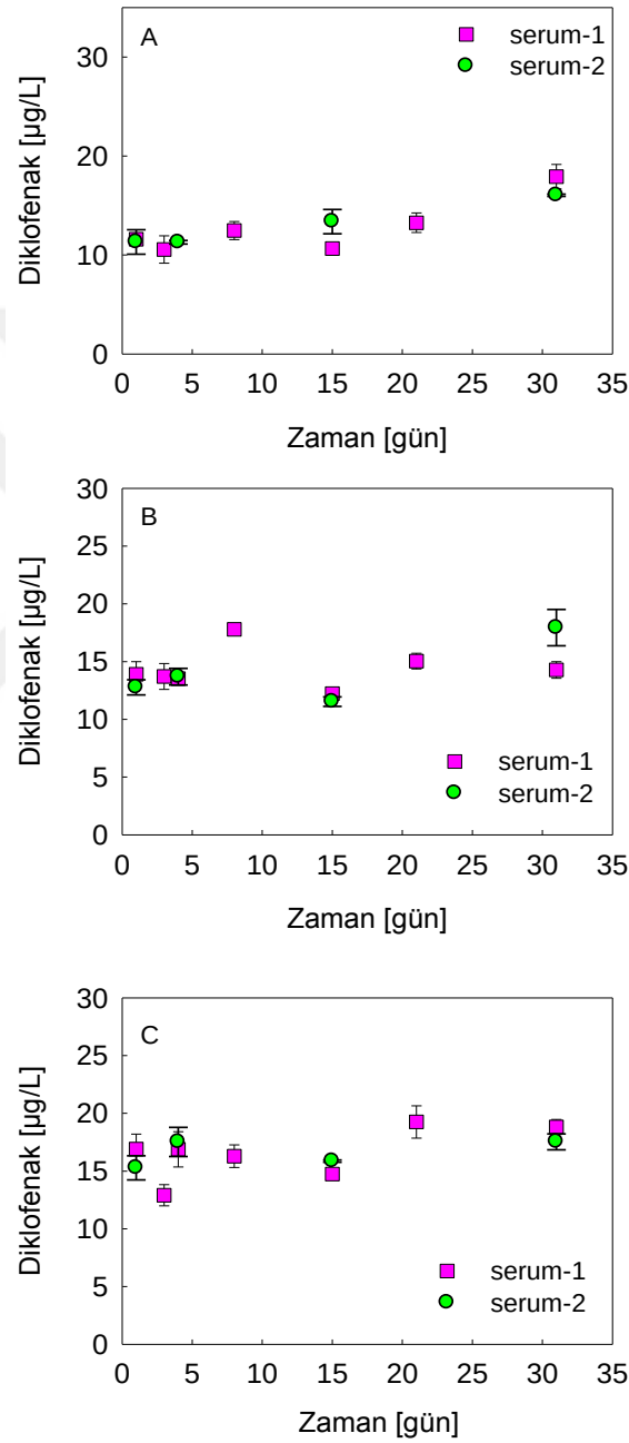
Şekil 4.22 : Diklofenak'a aklime olan ve çamur yaşı (A) 10 gün; (B) 20 gün ve (C) 40 gün için reaktörlerden alınan aşı ile aynı koşullarda kurulan iki kesikli reaktörde (serum-1 ve serum-2) Diklofenak giderim profilleri.
