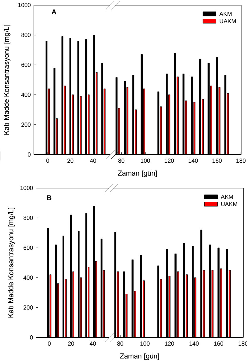
Şekil 4.6 : Denitrifikasyon yapan kontrol reaktörü (A) ve Diklofenak aklime reaktörde (B) AKM ve UAKM profilleri.
