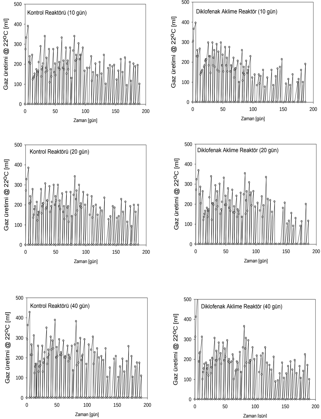
Şekil 4.11 : Farklı çamur yaşlarında işletilen anoksik reaktörlerde toplam gaz üretim profilleri.
