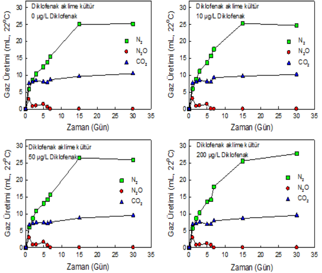
Şekil 4.16 : Diklofenak'a aklime olan kültürde farklı konsantrasyonlarda Diklofenak ilavesi sonucu gözlenen gaz üretim profilleri.
