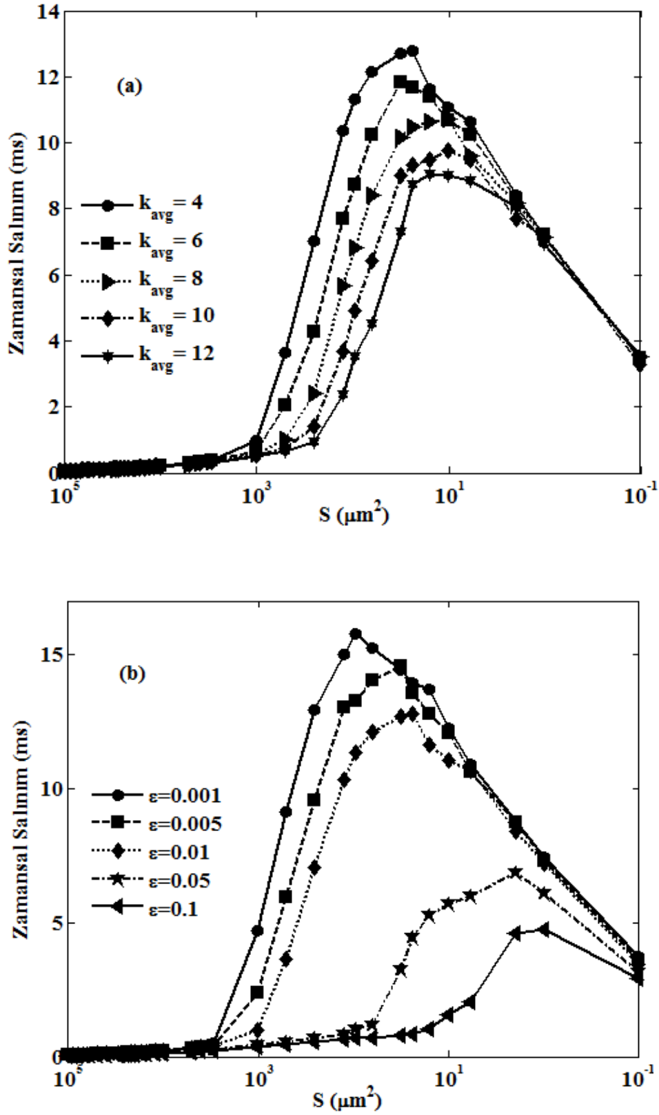
Şekil 4.28 \chi_K = 0.95 için membran alanına ( S ) bağlı olarak zamansal salınının ağ parametrelerine göre değişimi ( \chi_{Na} = 1 , A = 4 \mu A/cm^2 , f = 20 Hz , N = 200 , \varepsilon = 0.01 ): a) Ortalama bağlantı derecesi, k_{avg} 'ye bağlı değişimi, b) Kuplaj katsayısına, \varepsilon 'a bağlı değişimi.
