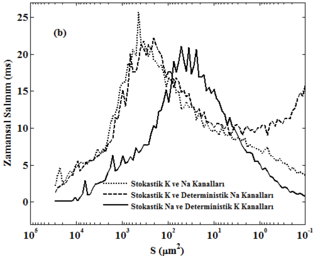
Şekil 4.6 142 Hz' lik bir uyarım frekansında membran alanına bağlı olarak her bir iyon kanalının latans istatistiklerindeki bağıl etkileri a) Ortalama latans b) Zamansal salınım.
