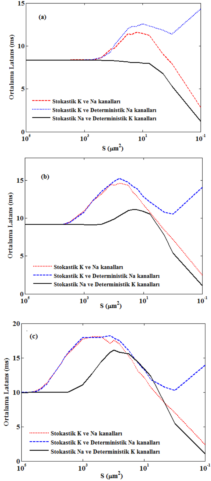
Şekil 4.31 Ölçeksiz bir nöral ağda iyon kanallarının latans istatistiklerine bağlı katkıları: membran alanına göre ortalama latansın değişimi ( A = 4 \mu\text{A}/\text{cm}^2 , f = 20 \text{ Hz} , N = 200 , \varepsilon = 0.01 , k_{\text{avg}} = 4 ) a) T = 4 °C, b) T = 6.3 °C, c) T = 7 °C.
