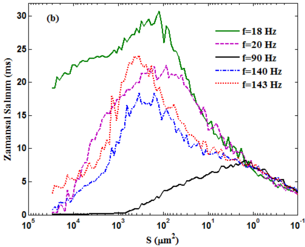
Şekil 4.1 Sabit genlikli eşik-üstü periyodik uyarımın frekansı ile latans dinamiklerinin membran alanına göre değişimi ( A = 4.0 \mu A/cm^2 ): a) Ortalama Latans, b) Zamansal salınım.
