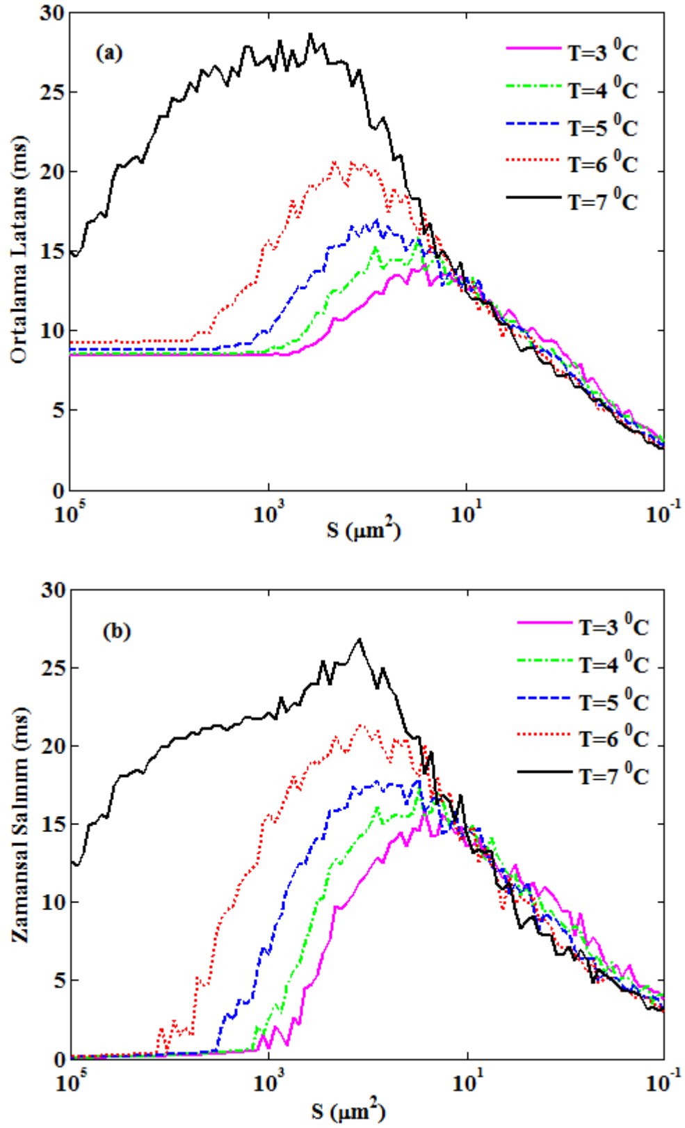
Şekil 4.12 Farklı sıcaklık değerleri için latans istatistiklerinin membran alanına göre değişimi ( A = 4 \mu\text{A}/\text{cm}^2 , f = 20 \text{ Hz} ): a) Ortalama Latans b) Zamansal salınım.
