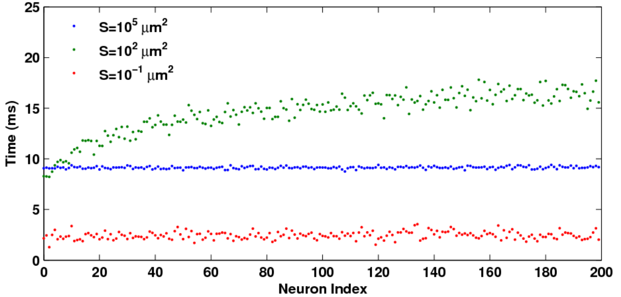
Şekil 4.19 Ölçeksiz ağda eşik-üstü periyodik bir uyartıma maruz kalmış 200 nöron tarafından üretilen ilk spaykların zaman-uzamsal dağılımı ( A = 4 \mu\text{A}/\text{cm}^2 , f = 20 \text{ Hz} , k_{avg} = 4 , \varepsilon = 0.01 ).
