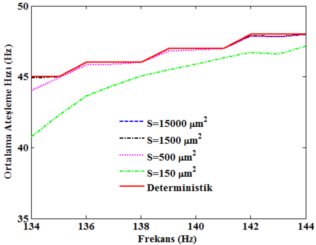
Şekil 4.16 Yarı stokastik nöron modelinde (deterministik potasyum ve stokastik sodyum kanalı) uyartım frekansına karşılık ateşleme frekansının değişimi ( A = 4 \mu A/cm^2 ): a) Alt sınır eşik değeri yakınında b) Üst eşik değeri yakınında.
