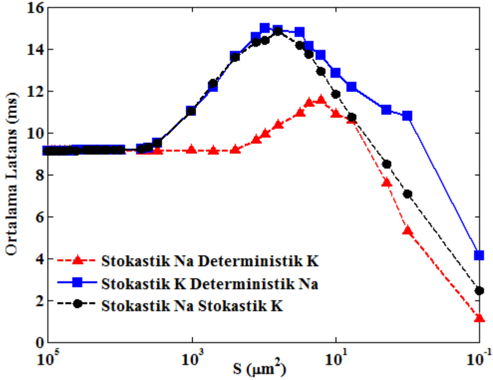
Şekil 4.25 Ölçeksiz nöral ağda potasyum ve sodyum iyon kanallarının NDD üzerindeki bağıl etkileri ( A = 4 \mu A/cm^2 , f = 20 \text{ Hz} , N=200 , \varepsilon=0.01 , k_{avg}=4 ).
