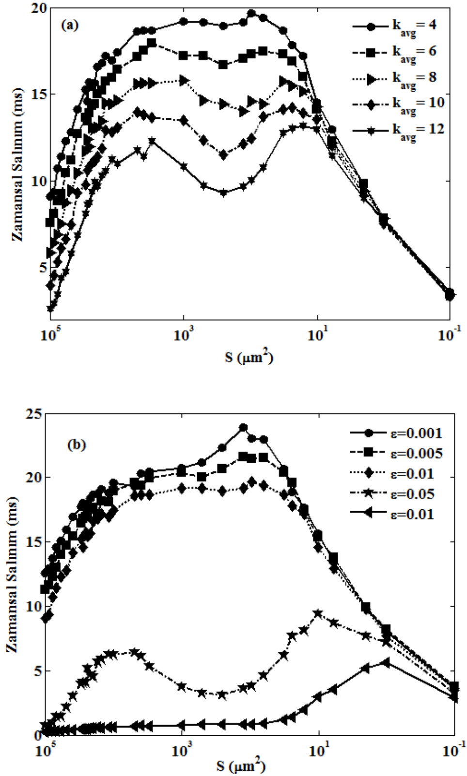
Şekil 4.29 \chi_{Na} = 0.95 için membran alanına ( S ) bağlı olarak zamansal salınının ağ parametrelerine göre değişimi ( \chi_K = 1 , A = 4 \mu\text{A}/\text{cm}^2 , f = 20 \text{ Hz} , N = 200 , \epsilon = 0.01 ): a) Ortalama bağlantı derecesi, k_{\text{avg}} 'ye bağlı değişimi, b) Kuplaj katsayısına, \epsilon 'a bağlı değişimi.
