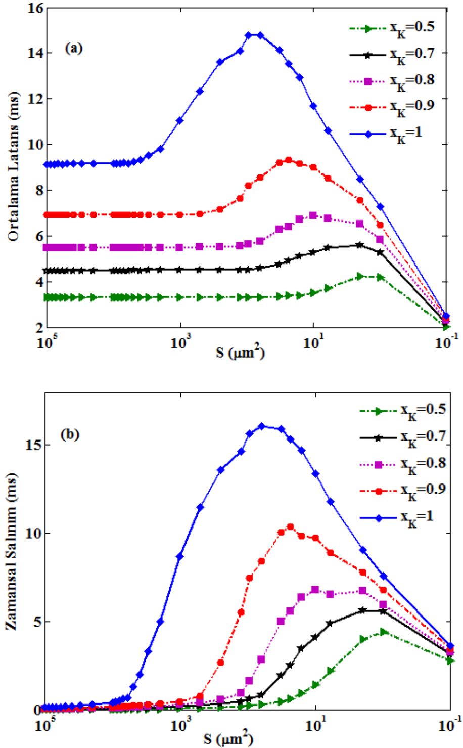
Şekil 4.26 Farklı potasyum kanal blokaması değerleri için ağın latans istatistiklerinin membran alanına bağlı olarak değişimi ( A = 4 \mu A/cm^2 , f = 20 Hz , N=200 , \epsilon=0.01 , k_{avg}=4 , \chi_{Na} = 1 ): a) Ortalama Latans, b) Zamansal Salınım.
