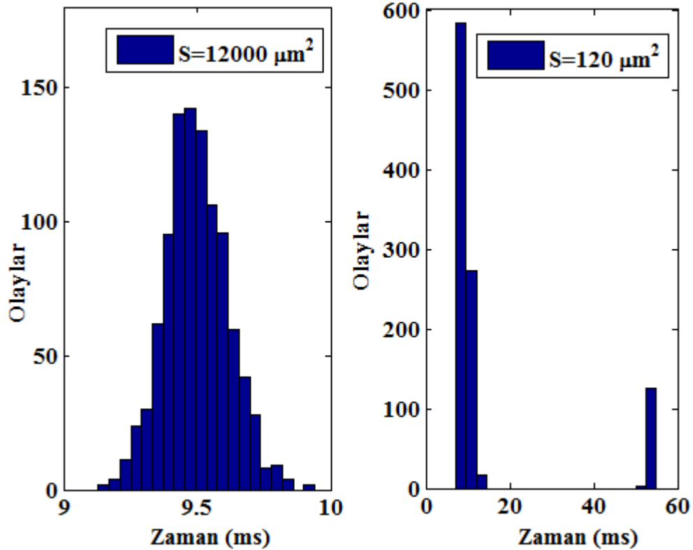
Şekil 4.7 Sadece sodyum iyon kanal gürültüsü yarı stokastik modelde iki farklı membran alanı için elde edilen ilk spayk zaman histogramları ( A = 4 \mu\text{A}/\text{cm}^2 , f = 20 \text{ Hz} ) a) S = 12000 \mu\text{m}^2 b) S = 120 \mu\text{m}^2 .
