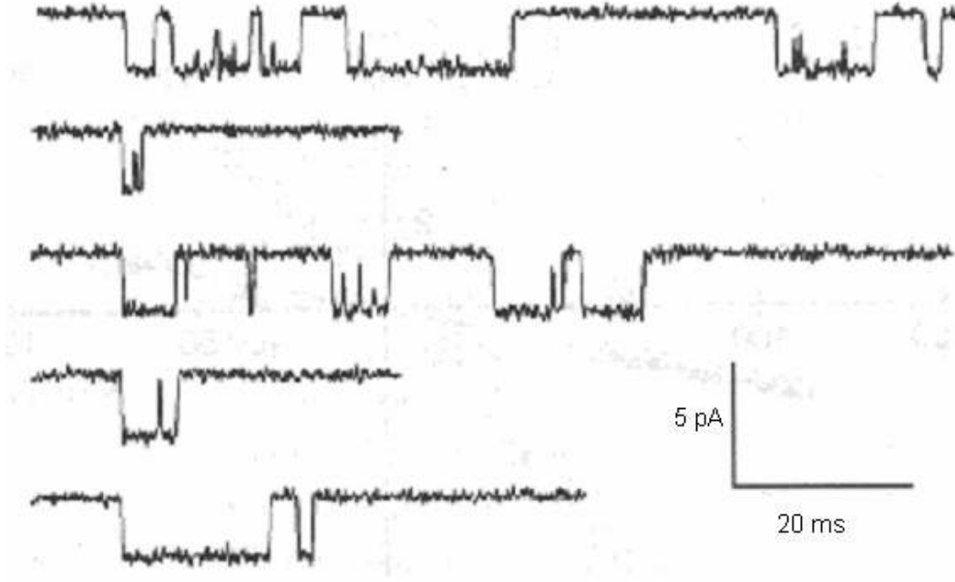
Şekil 2.5 Tek bir iyon kanalından kaydedilen akımın zamanla değişimi: Patch kenetleme tekniği kullanılarak hücre zar gerilimi 0 mV' a sabitlenmiştir. Kanal açık olduğunda yaklaşık 3 nA lik bir akım oluşmaktadır (aşağı yönlü). Eğrilerdeki küçük dalgalanmalar termal gürültüden kaynaklanmaktadır (Koch 1998).
