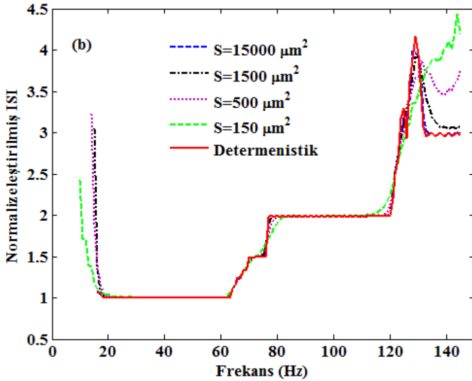
Şekil 4.14 Stokastik Hodgkin-Huxley nöron modelinin ateşleme karakteristikleri. Uyarım frekansına karşılık ( A = 4 \mu\text{A}/\text{cm}^2 ) a) Ortalama ateşleme hızının değişimi b) Spyaklar arası zaman aralığının (ISI) değişimi.
