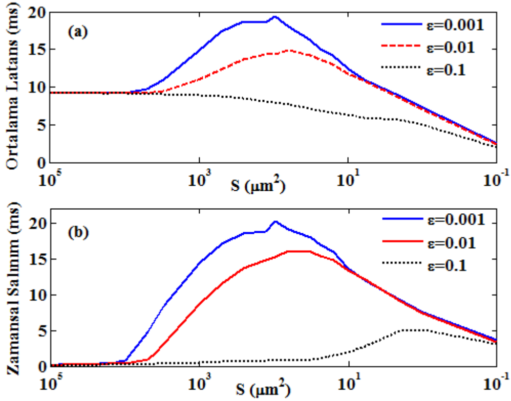
Şekil 4.23 Farklı kuplaj şiddetleri ( \epsilon ) için ölçeşiz nöral ağı latans istatistiklerinin membran alanına ( S ) bağlı olarak değişimi: a) Ortalama Latans, b) Zamansal Salınım ( A = 4 \mu A/cm^2 , f = 20 Hz , N = 200 , k_{avg} = 4 ).
