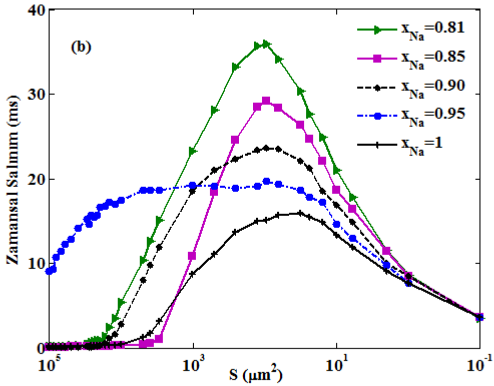
Şekil 4.27 Farklı sodyum kanal bloklaması değerleri için ağın ortalama latansının membran alanına bağlı olarak değişimi ( A = 4 \mu\text{A}/\text{cm}^2 , f = 20 \text{ Hz} , N=200 , \varepsilon = 0.01 , k_{avg} = 4 , \chi_K = 1 ).
