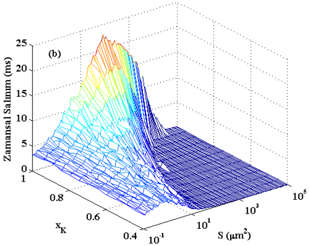
Şekil 4.10 Farklı potasyum kanal bloklama oranları için membran alanına karşın latans istatistiklerinin değişimi ( A = 4 \mu A/cm^2 , f = 20 Hz , \chi_{Na} = 1 ): a) Ortalama Latans b) Zamansal salınım.
