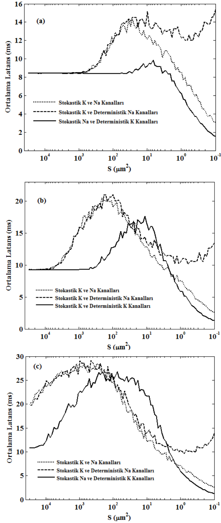
Şekil 4.13 İyon kanallarının latans istatistiklerine bağlı katkıları: membran alanına göre ortalama latansın değişimi ( A = 4 \mu A/cm^2 , f = 20 Hz ) a) T = 3 ^\circ C , b) T = 6 ^\circ C , c) T = 7 ^\circ C .
