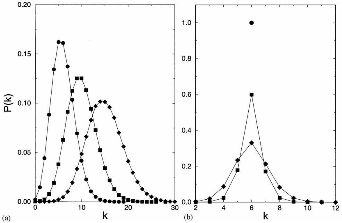
Şekil 3.3 Erdős-Rényi ve Watts-Strogatz modellerinin bağlanabilirlik dağılımları. a) 10000 adet düğümden oluşan Erdős-Rényi ağ modeli için farklı p_{ER} değerlerinde bağlanabilirlik dağılımı P(k) 'nin değişimi. p_{ER} = 0.0006 (yuvarlak), p_{ER} = 0.001 (kare), p_{ER} = 0.0015 (baklava şekli) b) 10000 adet düğümden oluşan Watts-Strogatz modeli için farklı p_{WS} değerlerinde bağlanabilirlik dağılımı P(k) 'nin değişimi ( \langle k \rangle = 6 ). p_{WS} = 0 (yuvarlak), p_{WS} = 0.1 (kare), p_{WS} = 0.3 (baklava şekli) (Barabási et al. 1999).
