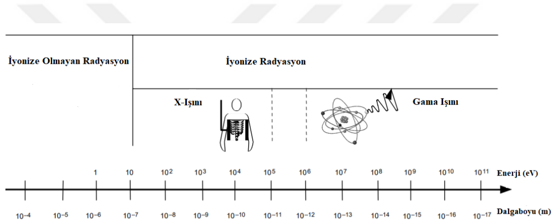
Şekil 2.4. X ve \gamma -ışınlarının elektromanyetik spektrumdaki yerleri [14]
