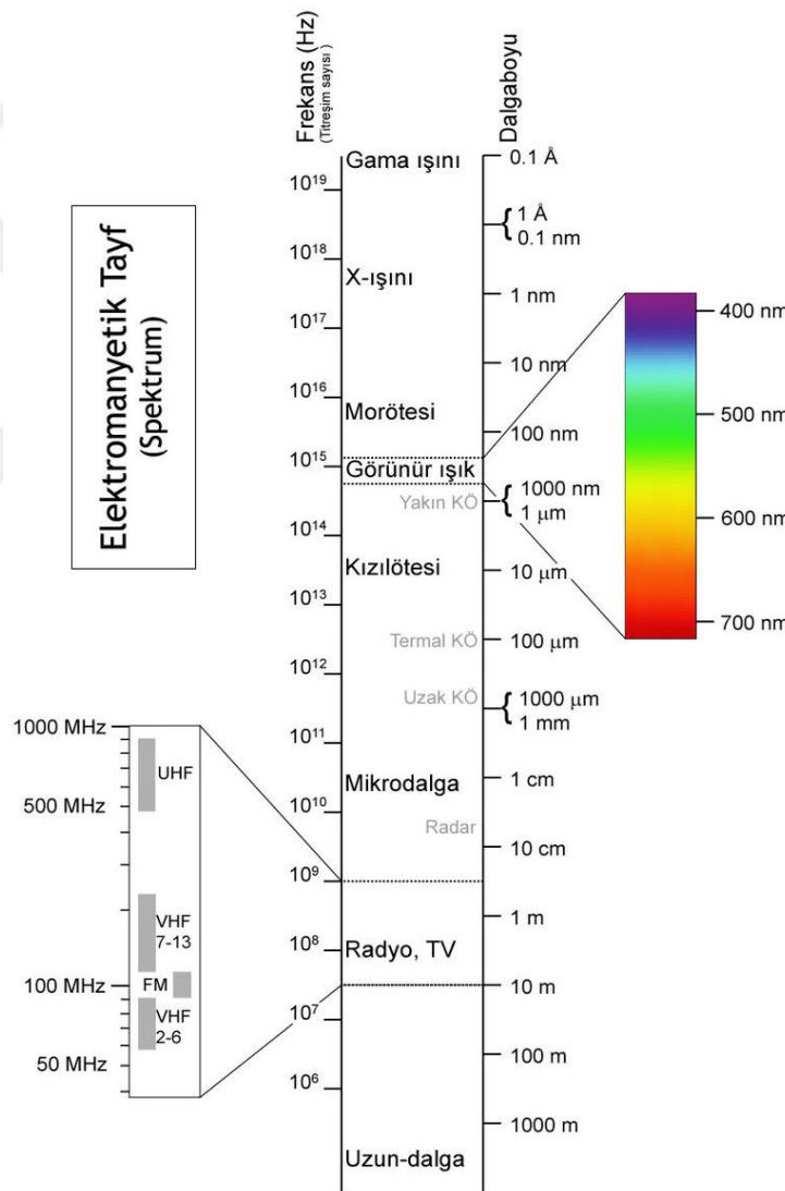
Şekil 2.3. Elektromanyetik spektrum [11]
