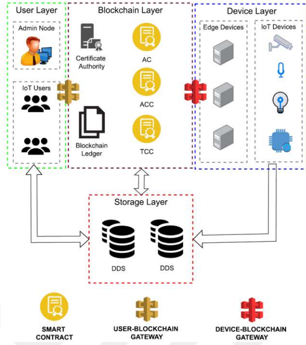
Şekil 2.1. TABI mimarisi [52]
