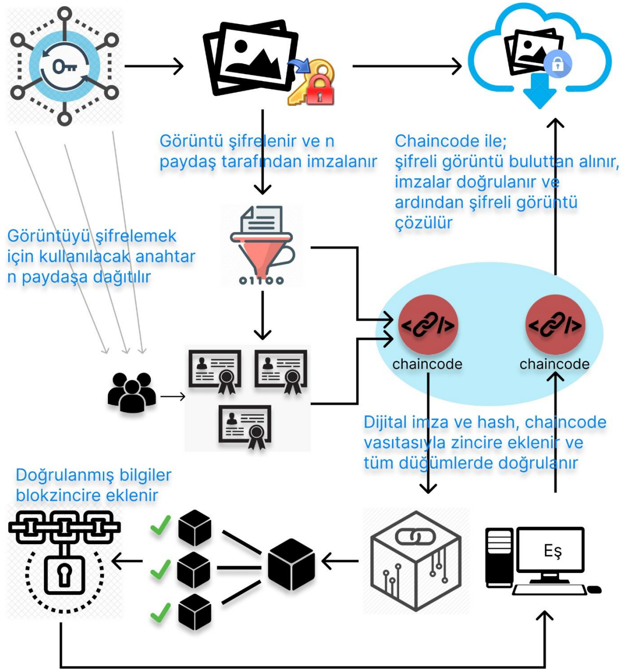
Şekil 4.1. Önerilen şemanın blok yapısı
