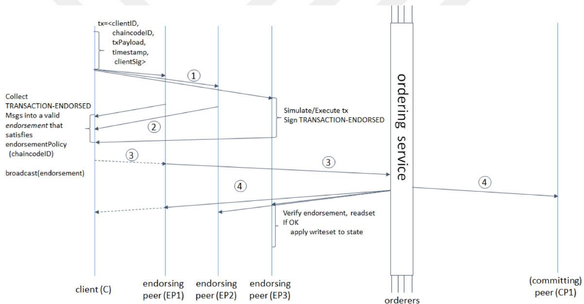
Şekil 4.7. Hyperledger Fabric'in işlem akış şeması.
