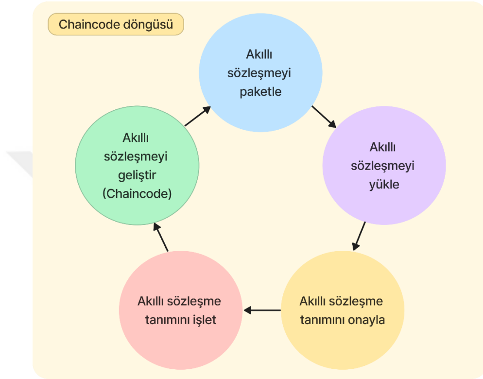
Şekil 3.6. Chaincode yaşam döngüsü
