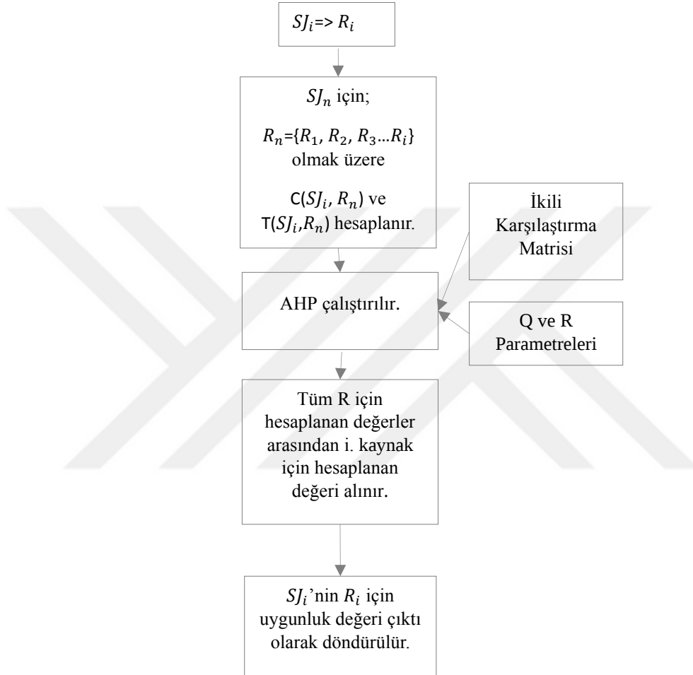
Şekil 4.36. İş parçası-kaynak ataması değerlendirme diyagramı.
