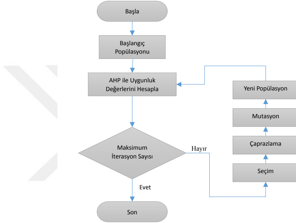
Şekil 4.42. Genetik algoritma akış diyagramı.
