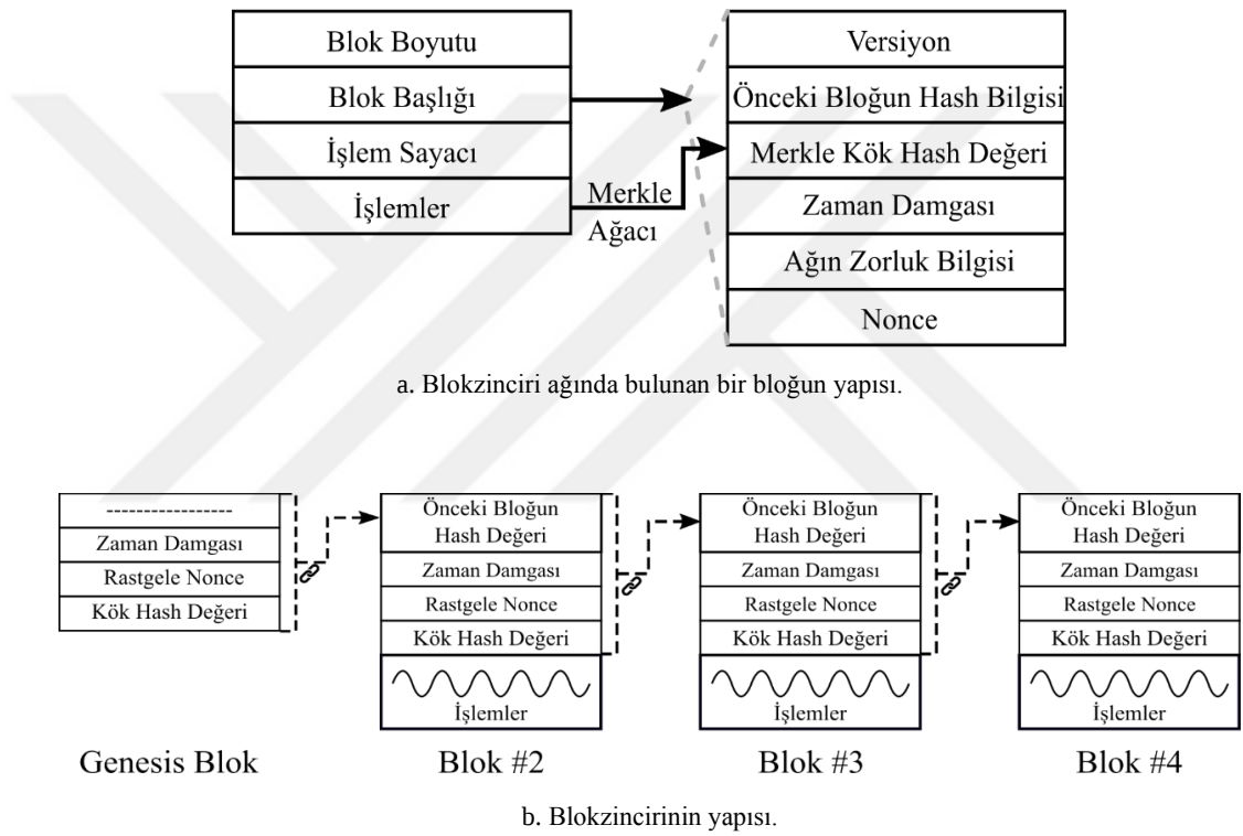
Şekil 3.2. Blokzinciri ağ yapısı.
