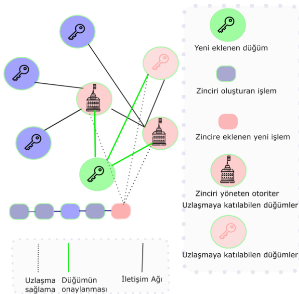
Şekil 3.8. Konsorsiyum blokzinciri ağ yapısı.
