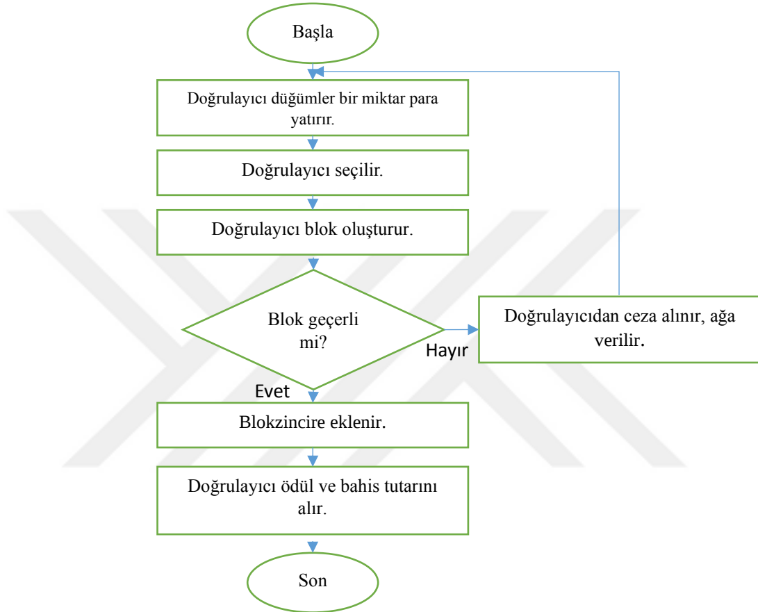
Şekil 3.4. PoS protokolünün çalışma işleyişi.
