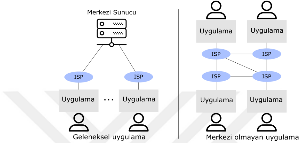
Şekil 3.10. Geleneksel ve merkezi olmayan uygulama.
