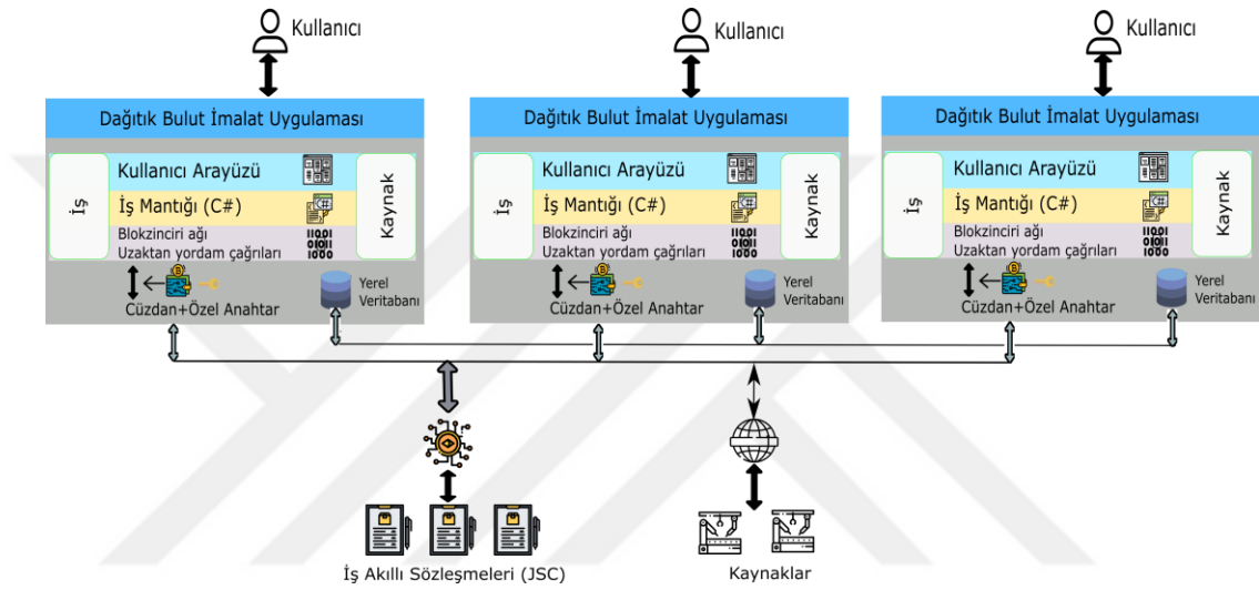
Şekil 4.10. DCMAApp uygulama diyagramı.
