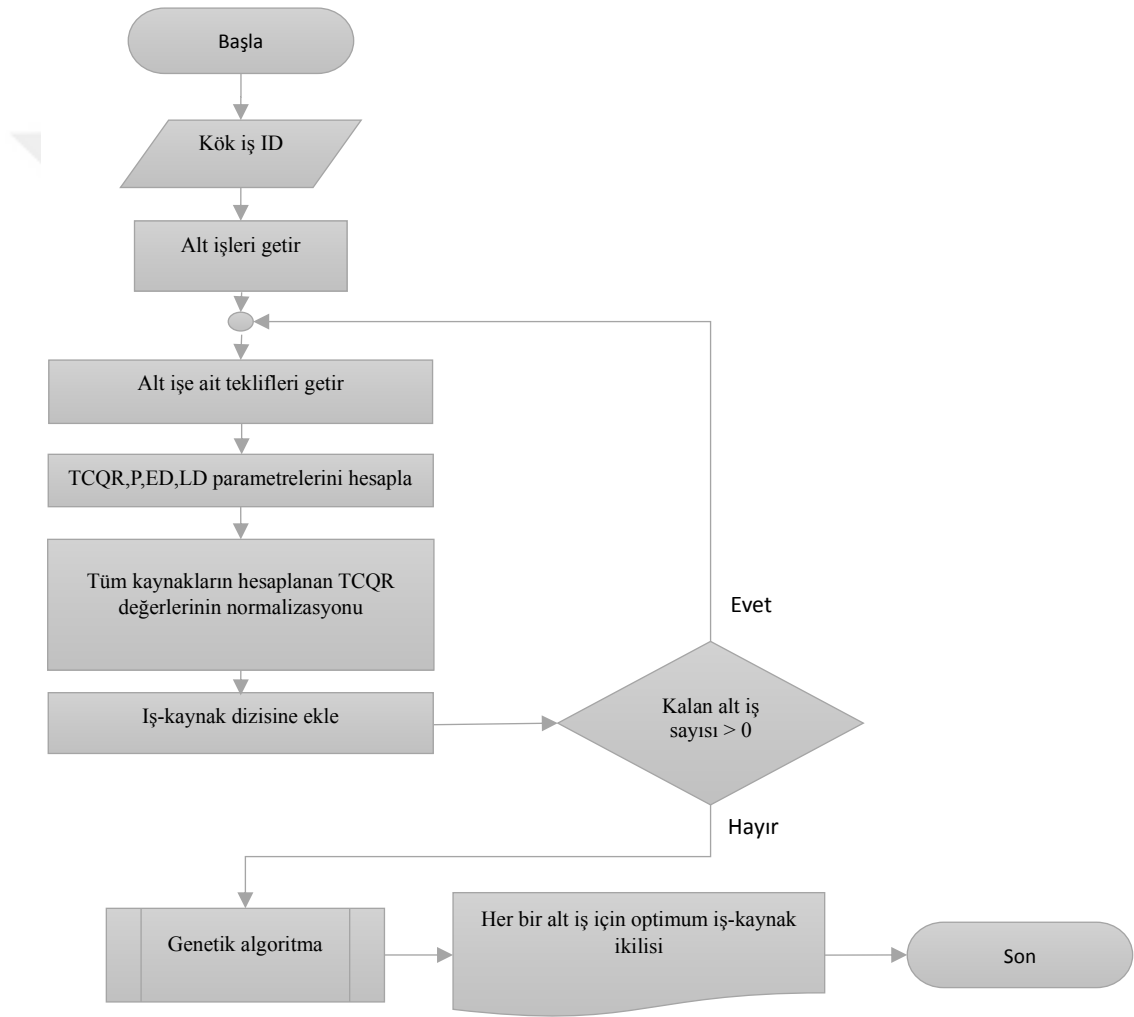
Şekil 4.41. DCMAApp kaynak planlama algoritması.
