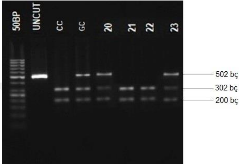
Şekil 7. rs4796793 (502 bç) MwoI restriksiyon endonükleaz enzimi ile kesim paternlerinin görüntüsü. (Uncut kesilmemiş PZR ürünü (502 bç), CC genotipi (302, 200 bç), GC genotipi (502, 302, 200 bç) bç:baz çifti
