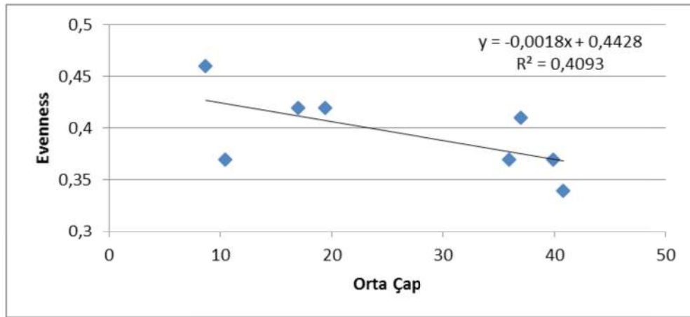
Şekil 3.10. Sarıçamda meşcere orta çapına bağlı olarak evenness (homojenlik) değeri.
