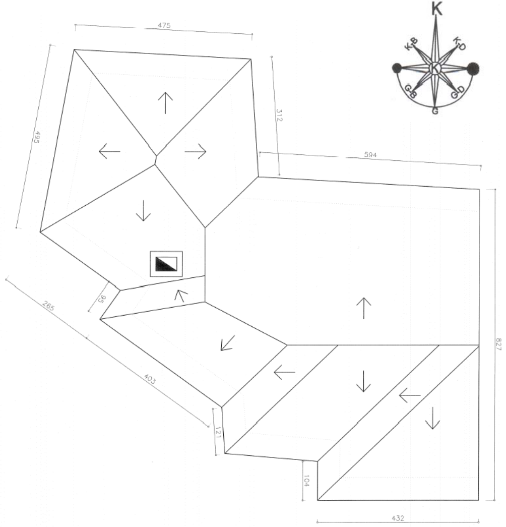
Plan 14: Çatı planı (Ankara Kültür ve Tabiat Varlıklarını Koruma Bölge Kurulu arşivinden alınmıştır.)
