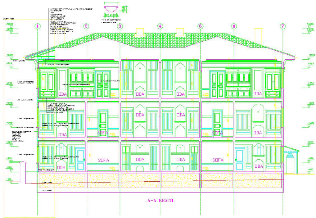
Kesit 8: A-A Kesiti(Bolu Belediyesi arşivinden alınmıştır.)
