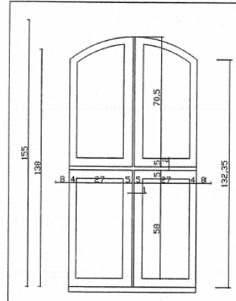
Çizim 44-45: Zemin Kat Pencere Çizimleri(Ankara Kültür ve Tabiat Varlıklarını Koruma Bölge Kurulu arşivinden alınmıştır.)
