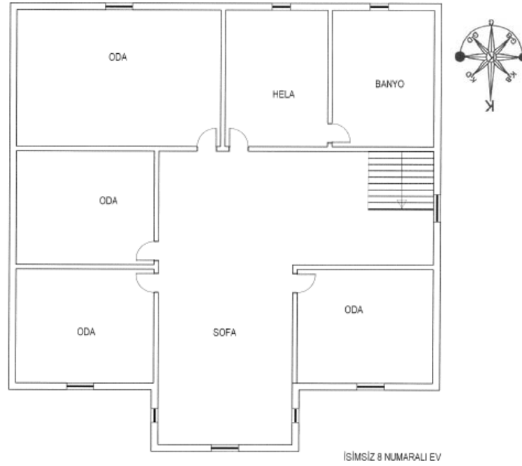
Plan 63: 8 Numaralı Ev birinci kat planı(Hazırlayan Ebru Eroğlu)
