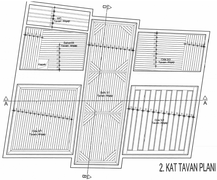
Plan 5: İkinci kat tavan planı(Ankara Kültür ve Tabiat Varlıklarını Koruma Bölge Kurulu arşivinden alınmıştır.)
