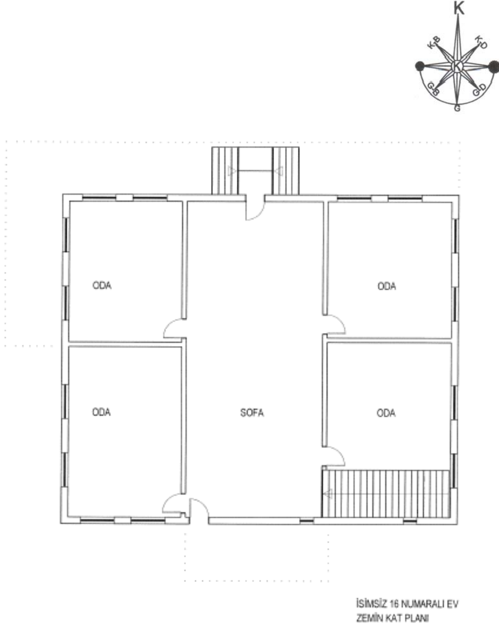
Plan 21: 16 Numaralı Ev Zemin Kat Planı(Hazırlayan Ebru Eroğlu)
