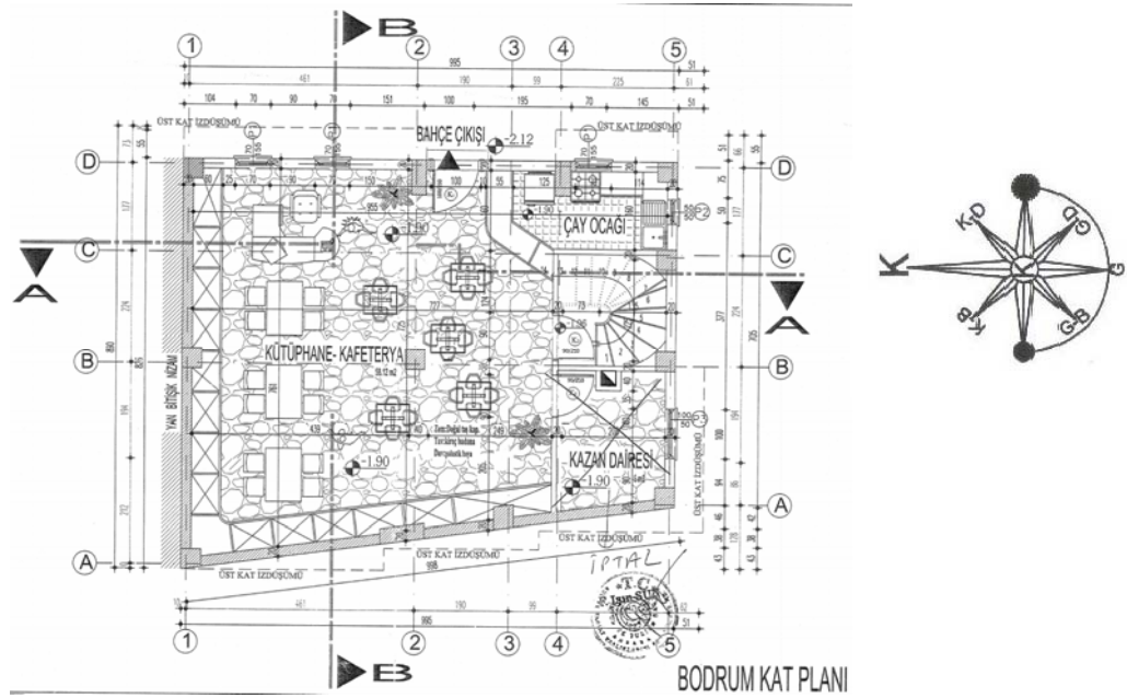
Plan 57: Bodrum Kat Planı (Bolu Belediye'si arşivinden alınmıştır.)
