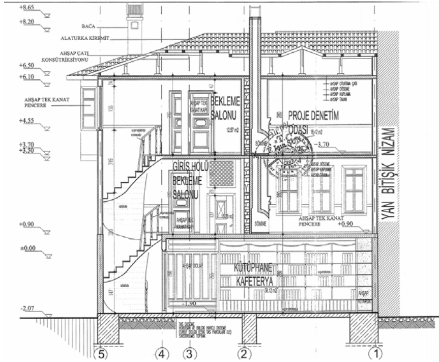
Kesit 12: A-A Kesiti (Bolu Belediye'si arşivinden alınmıştır.)
