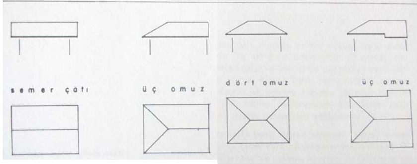
Çizim 48: Doğu Karadeniz evlerine ait çatı çizimleri(Orhan Özgüner'den)
