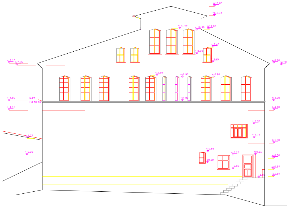
Çizim 21: Yapıdan kuzey cephe(Bolu Belediye'si arşivinden alınmıştır.)
