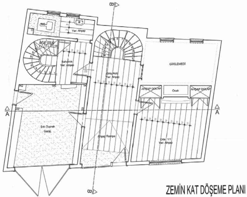
Plan 10: Zemin kat döşeme planı(Ankara Kültür ve Tabiat Varlıklarını Koruma Bölge Kurulu arşivinden alınmıştır.)
