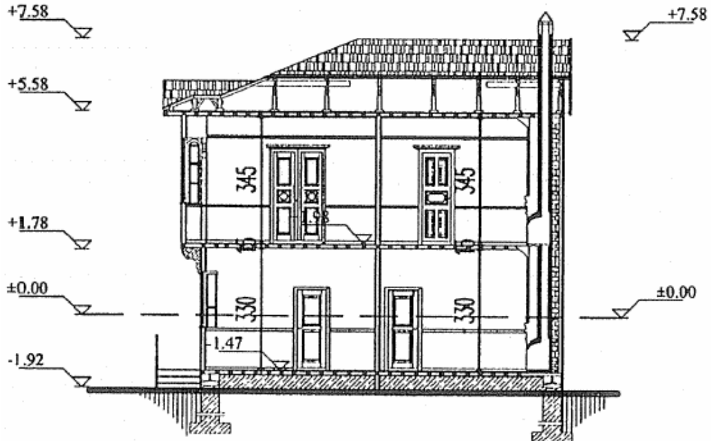
Kesit 11: B-B Kesiti(Bolu Belediyesi arşivinden alınmıştır.)
