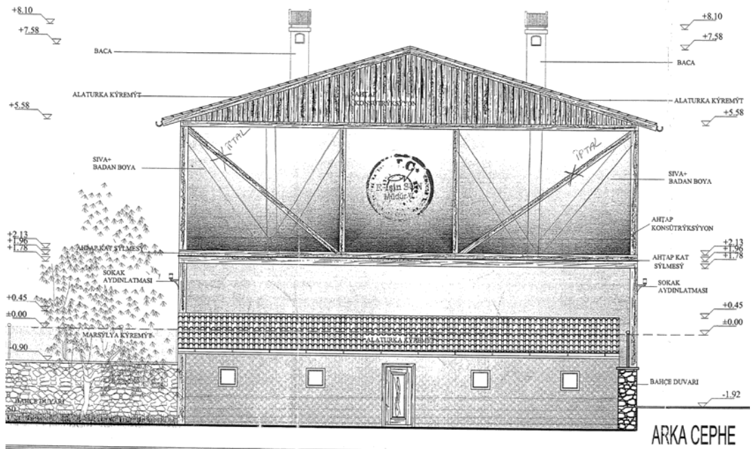
Çizim 30: Kuzeydoğu cephe(Bolu Belediyesi arşivinden alınmıştır.)
