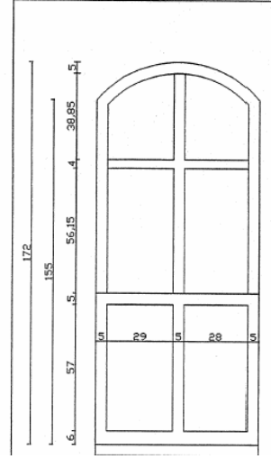
Çizim 42-43: Birinci Kat Pencere Çizimleri(Ankara Kültür ve Tabiat Varlıklarını Koruma Bölge Kurulu arşivinden alınmıştır.)
