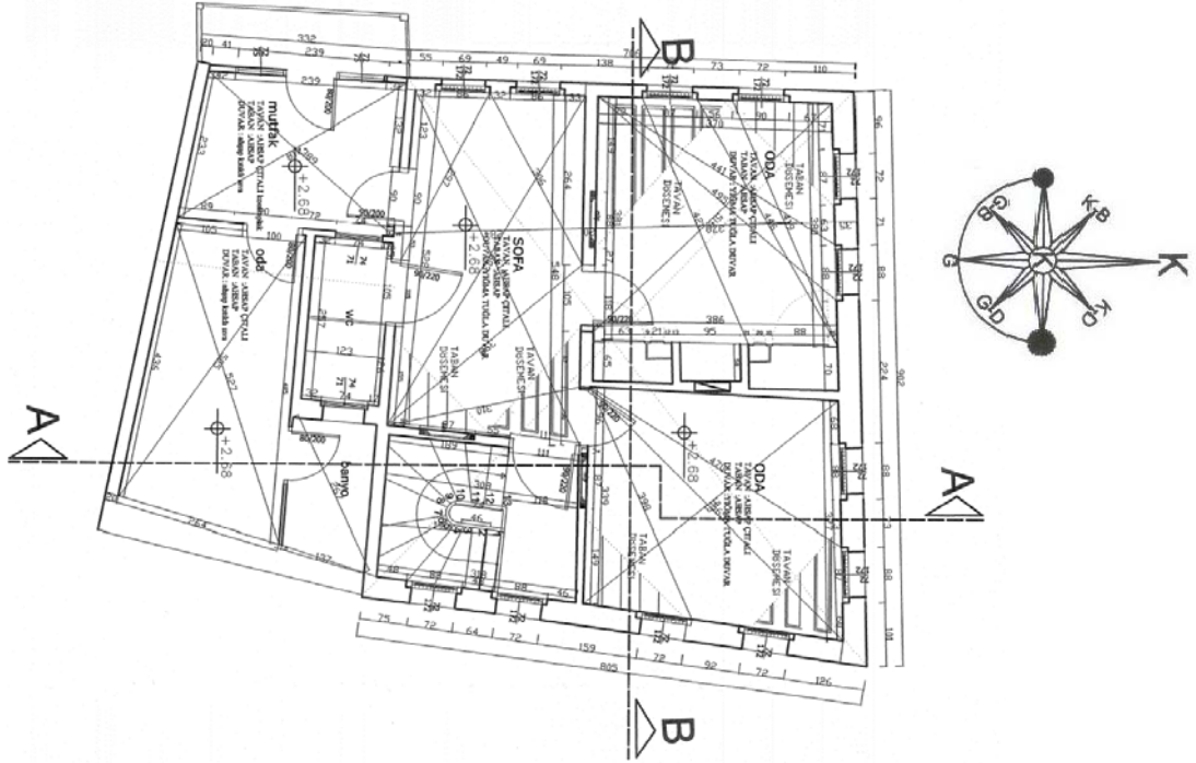
Plan 58: Birinci Kat Planı (Ankara Kültür ve Tabiat Varlıklarını Koruma Bölge Kurulu arşivinden alınmıştır.)
