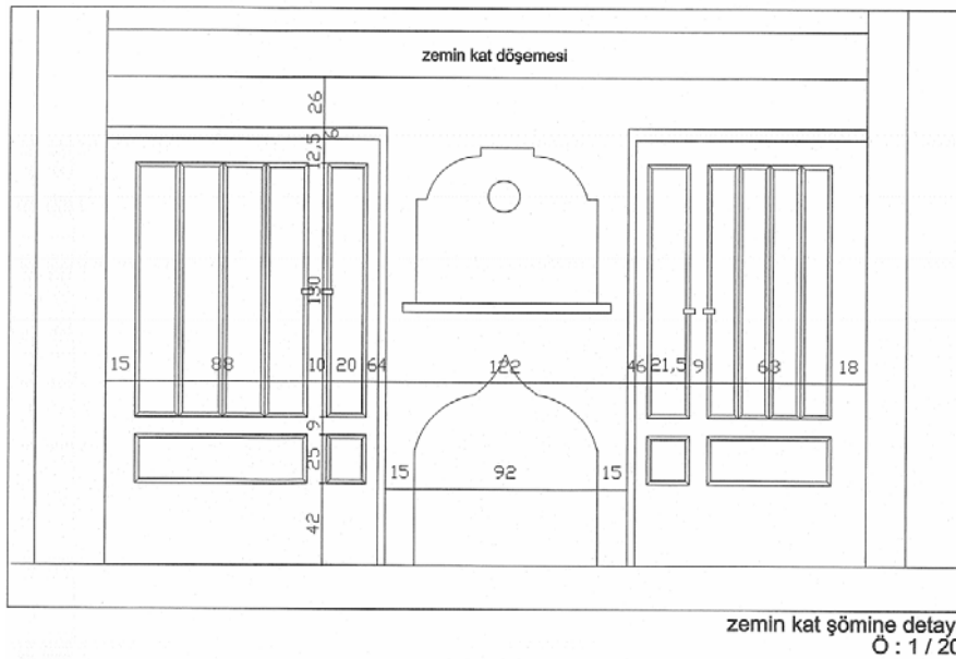
Çizim 38: Zemin kat ocak detayı(Ankara Kültür ve Tabiat Varlıklarını Koruma Bölge Kurulu arşivinden alınmıştır.)
