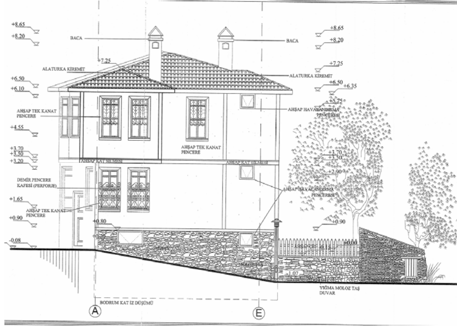
Çizim 34: Güney cephe (Bolu Belediye'si arşivinden alınmıştır.)
