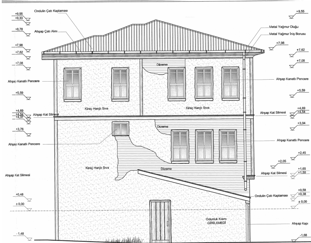
Çizim 5: Yapıdan kuzeybatı cephe(Ankara Kültür ve Tabiat Varlıklarını Koruma Bölge Kurulu arşivinden alınmıştır.)
