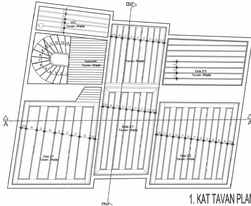
Plan 6: Birinci kat tavan planı (Ankara Kültür ve Tabiat Varlıklarını Koruma Bölge Kurulu arşivinden alınmıştır.)
