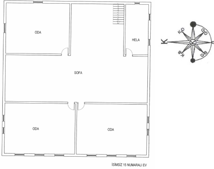
Plan 18: 15 Numaralı Ev Birinci Kat Planı(Hazırlayan Ebru Eroğlu)
