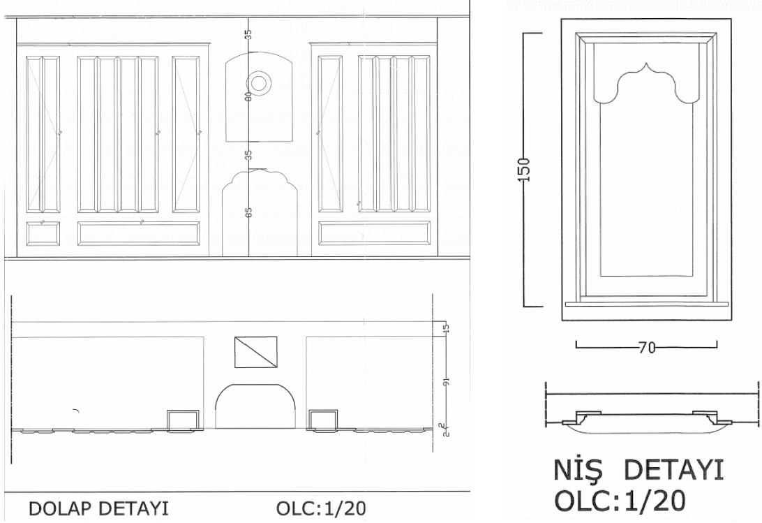
Çizim 14-15: Ocak, yüklük ve çiçeklik (Ankara Kültür ve Tabiat Varlıklarını Koruma Bölge Kurulu arşivinden alınmıştır).
