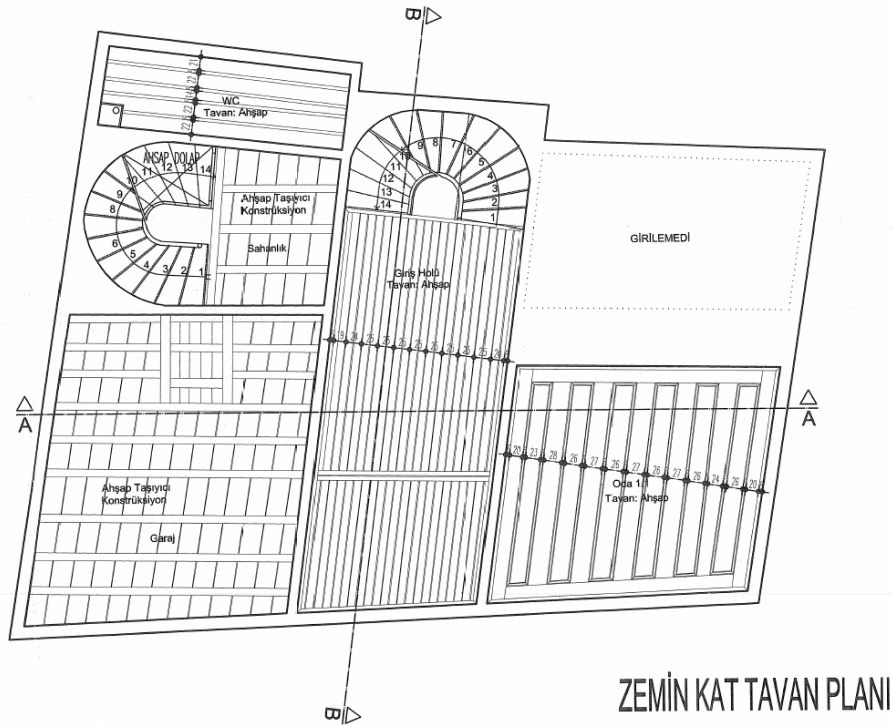
Plan 7: Zemin kat tavan planı (Ankara Kültür ve Tabiat Varlıklarını Koruma Bölge Kurulu arşivinden alınmıştır.)
