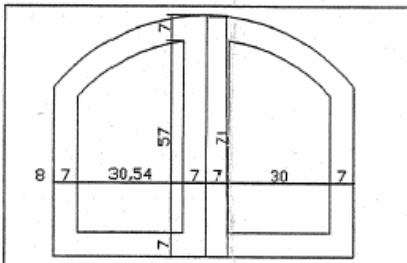
Çizim 44-45: Zemin Kat Pencere Çizimleri(Ankara Kültür ve Tabiat Varlıklarını Koruma Bölge Kurulu arşivinden alınmıştır.)
