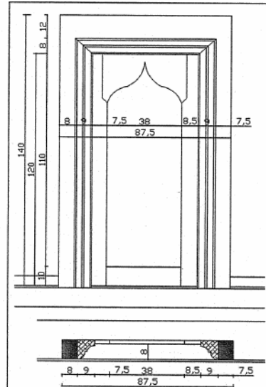
Fotoğraf 302: Çiçeklik örneği Çizim 40–41: Zemin ve birinci kat çiçeklik çizimi (Ankara Kültür ve Tabiat Varlıklarını Koruma Bölge Kurulu arşivinden alınmıştır.)
