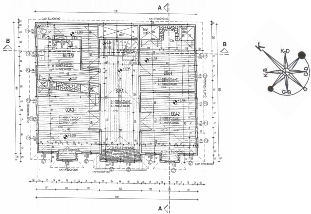
Plan 52: Birinci Kat Planı(Bolu Belediyesi arşivinden alınmıştır.)
