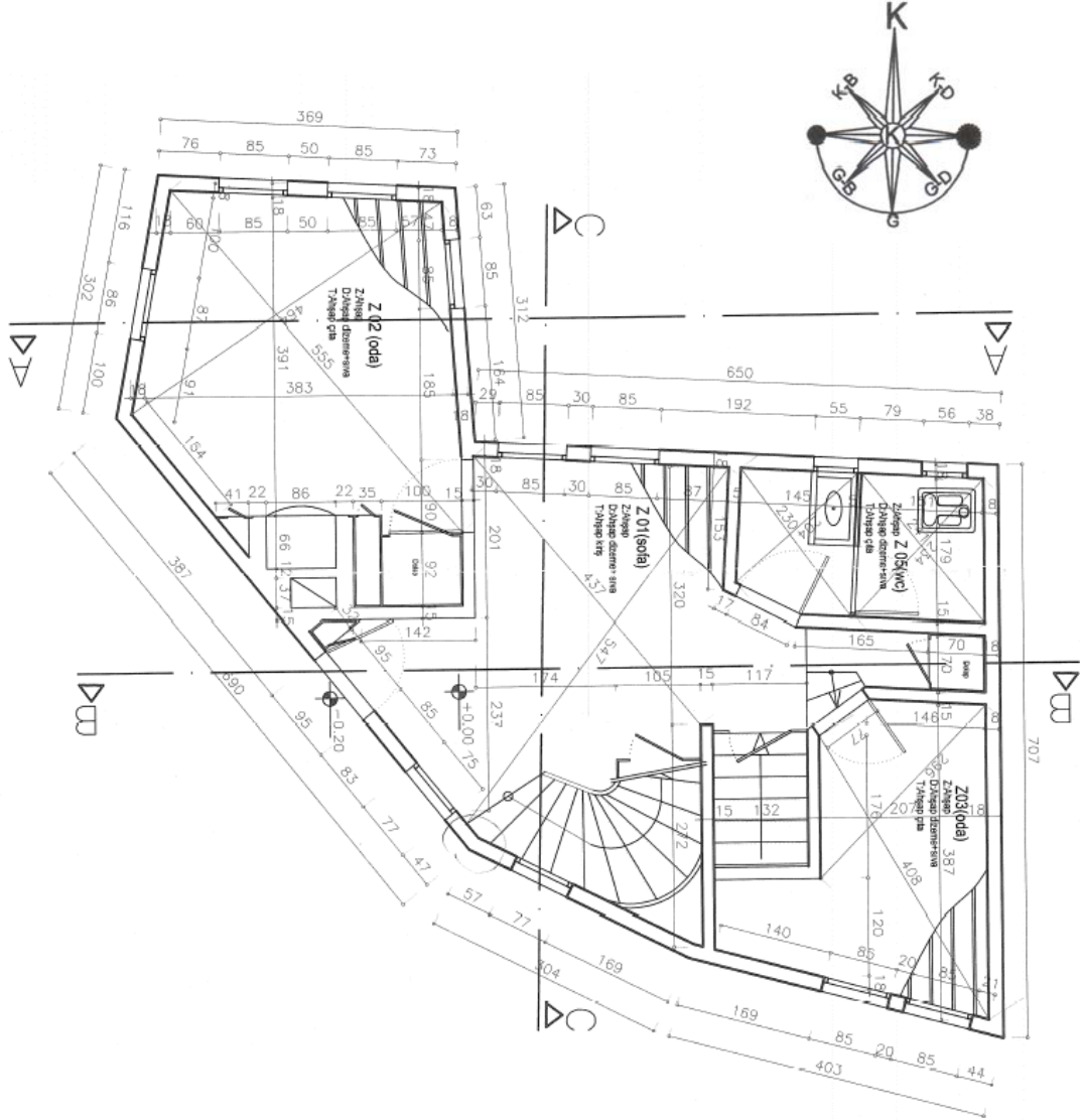
Plan 16: Zemin kat planı(Ankara Kültür ve Tabiat Varlıklarını Koruma Bölge Kurulu arşivinden alınmıştır.)
