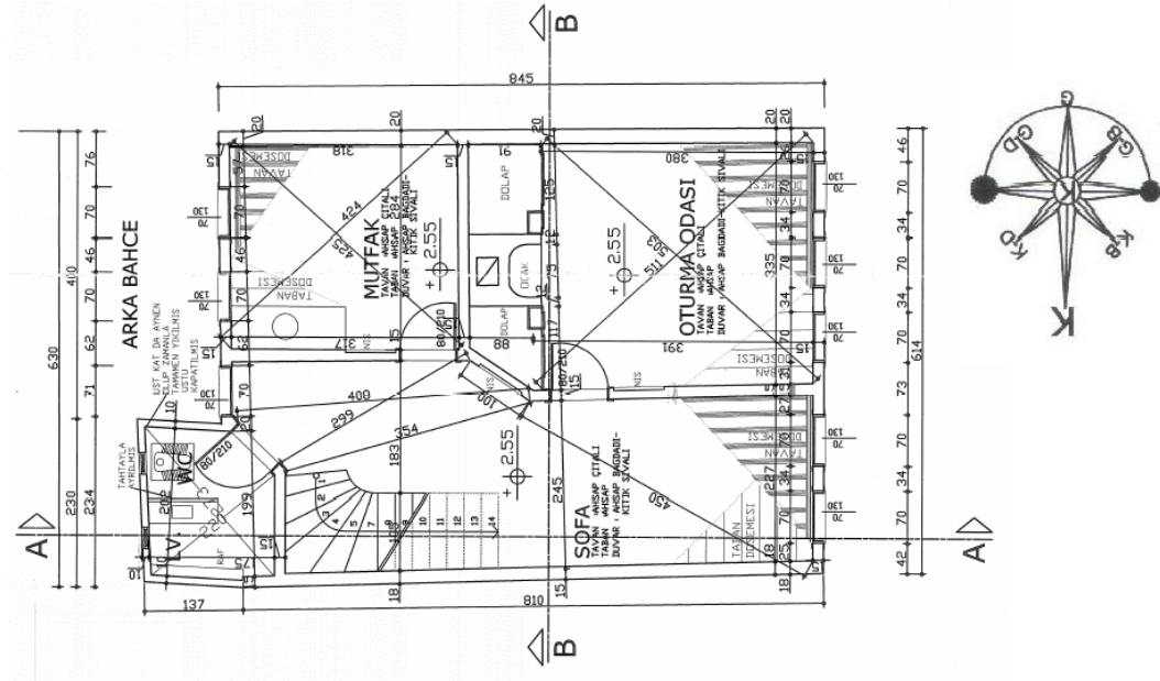
Plan 24: Birinci Kat Planı (Ankara Kültür ve Tabiat Varlıklarını Koruma Bölge Kurulu arşivinden alınmıştır).
