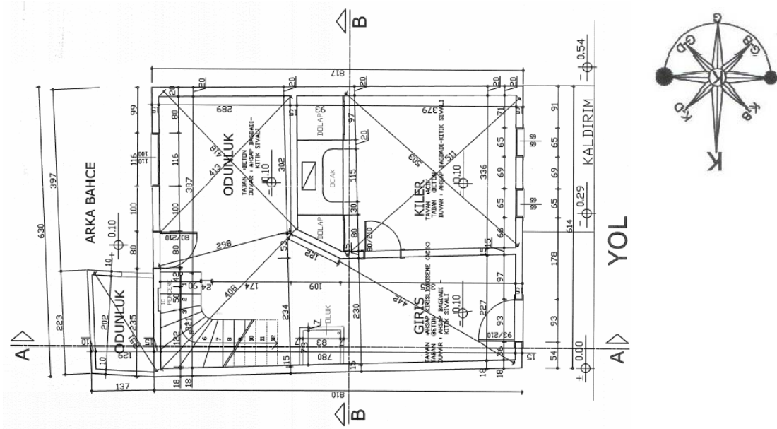
Plan 25: Zemin Kat Planı (Ankara Kültür ve Tabiat Varlıklarını Koruma Bölge Kurulu arşivinden alınmıştır).
