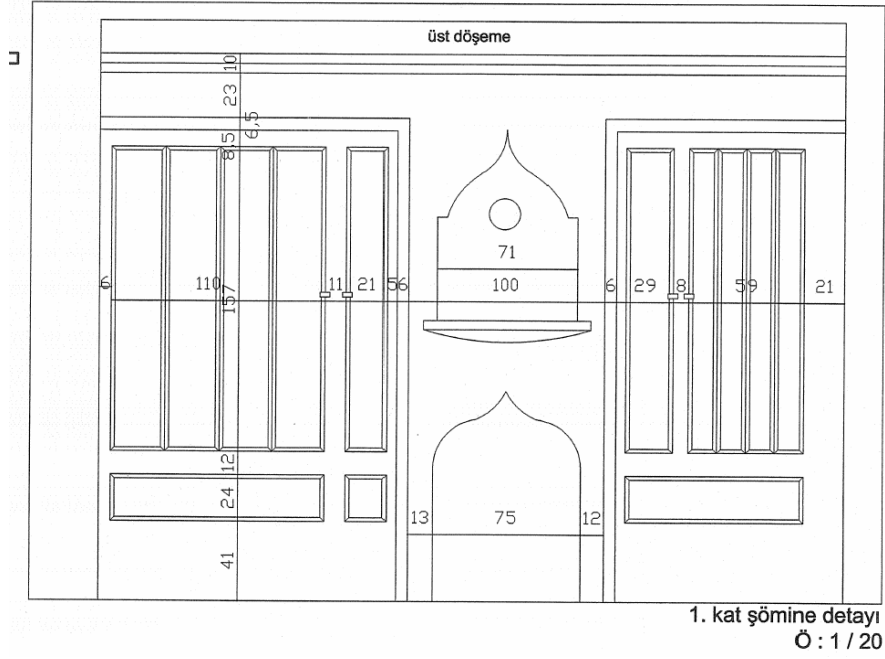
Çizim 39: Birinci kat ocak detayı (Ankara Kültür ve Tabiat Varlıklarını Koruma Bölge Kurulu arşivinden alınmıştır.)
