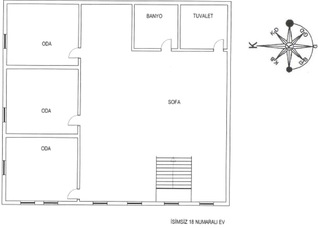
Plan 26: 18 Numaralı Ev Birinci Kat Planı(Hazırlayan Ebru Eroğlu)
