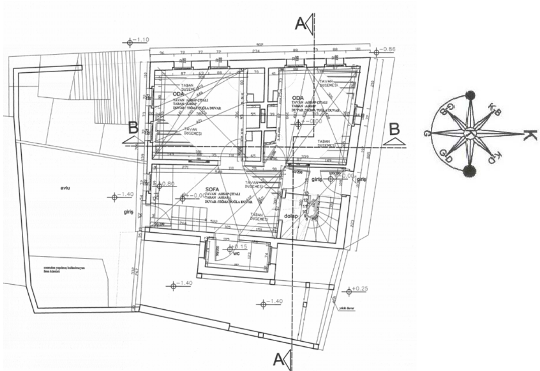
Plan 59: Zemin Kat Planı (Ankara Kültür ve Tabiat Varlıklarını Koruma Bölge Kurulu arşivinden alınmıştır.)
