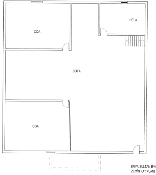
Plan 46: Zemin Kat Planı(Hazırlayan Ebru Eroğlu)
