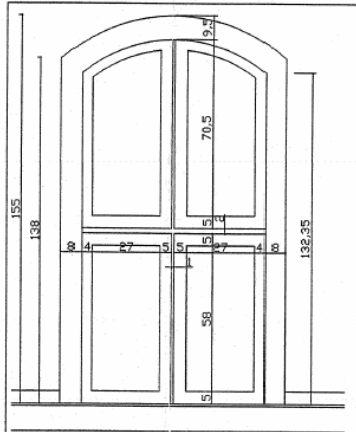
Çizim 44-45: Zemin Kat Pencere Çizimleri(Ankara Kültür ve Tabiat Varlıklarını Koruma Bölge Kurulu arşivinden alınmıştır.)
