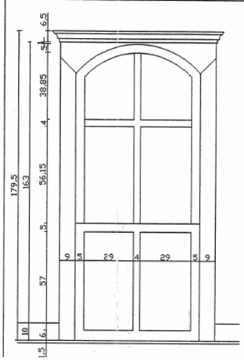
Çizim 42-43: Birinci Kat Pencere Çizimleri(Ankara Kültür ve Tabiat Varlıklarını Koruma Bölge Kurulu arşivinden alınmıştır.)
