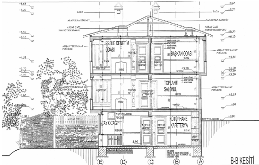
Kesit 13: B-B Kesiti (Bolu Belediye'si arşivinden alınmıştır.)
