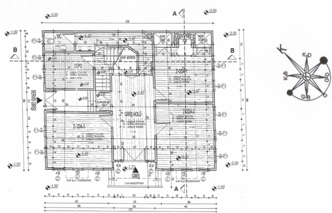
Plan 53: Zemin Kat Planı(Bolu Belediyesi arşivinden alınmıştır.)
