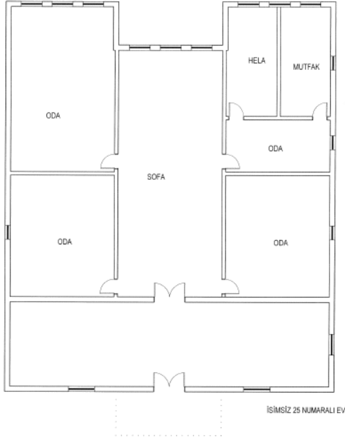
Plan 35: 25 Numaralı Ev Birinci Kat Planı(Hazırlayan Ebru Eroğlu)
