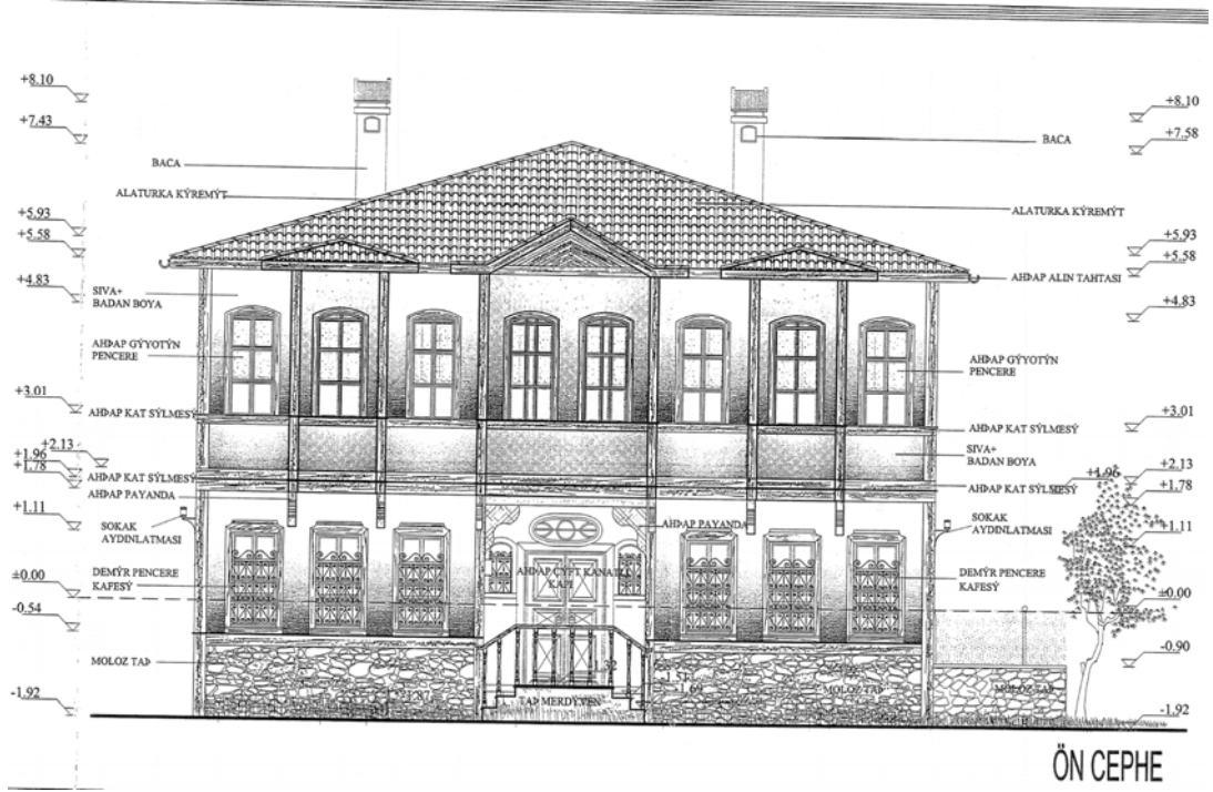
Çizim 27: Güneybatı cephe(Bolu Belediyesi arşivinden alınmıştır.)
