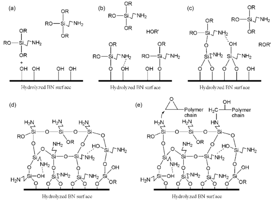
Şekil 1.3.1.a) Takviye malzemesine bağlanmış olan siloksanların polimer ile kombinasyonu şematik olarak gösterimi [29].
