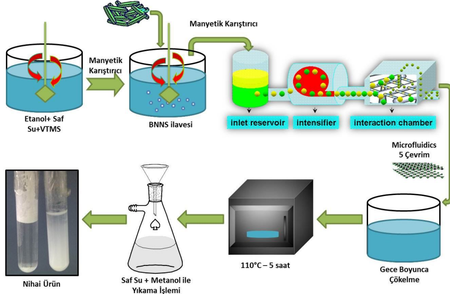
Şekil 2.2.4.b. Silanlama süreci akım şeması
