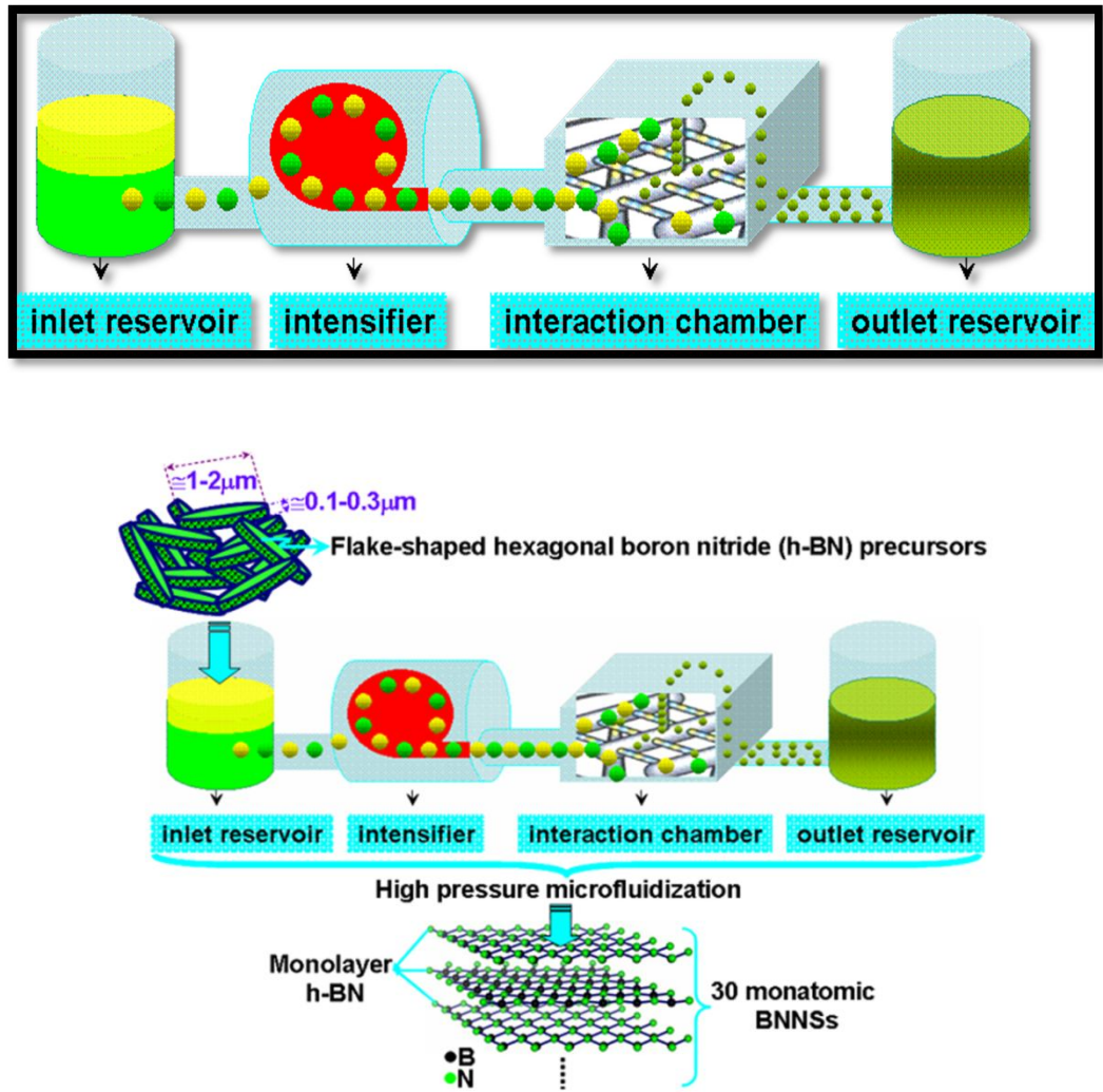
Şekil 2.2.3.a Yüksek Kayma Hızlı Sıvı Mikro İşlemci (Microfluidizier)
