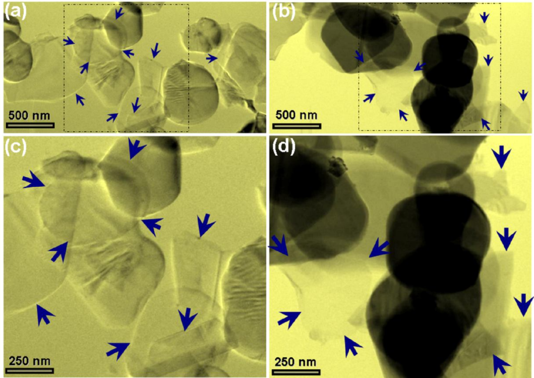
Şekil 3.1.2.b.(a, c)Microfluidics tekniği ile üretilmiş BNNS' lerin farklı numunelerden elde edilen düşük büyütmelerdeki bright field (BF)-TEM görüntüleri. Mavi oklar ile gösterilen şeffaf bölgeler BNNS' lere karşılık gelmektedir.
