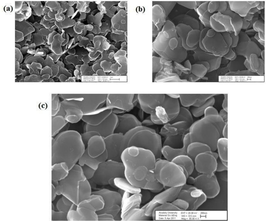
Şekil 3.1.1.b.(a, b, c). Yüksek kayma hızlı sıvı mikro işlemcide 20 çevrim işlem görmüş tabakalarına ayrılmış hekzagonal bor nitrür SEM görüntüleri
