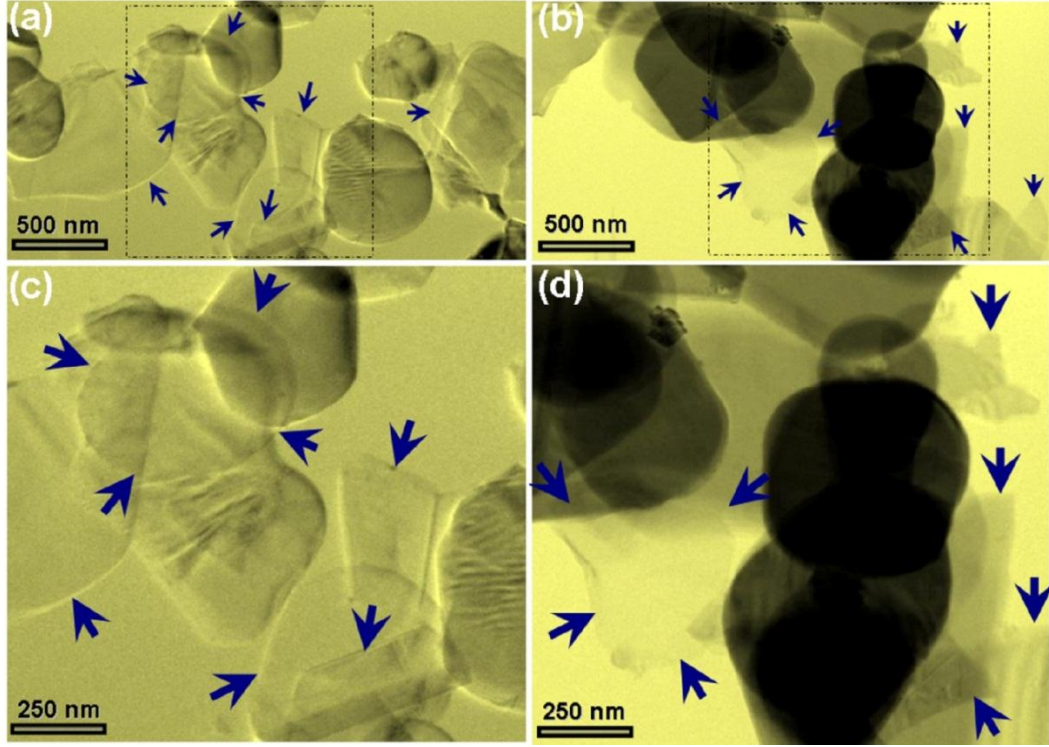
Şekil 4.20. Yüksek kayma hızlı sıvı mikro işlemci tekniği ile üretilmiş BNNS’ lerin farklı numunelerden elde edilen düşük büyütmeledeki bright field (BF)-TEM görüntüleri
