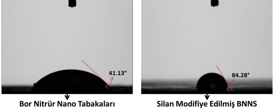
Şekil 4.37. Statik temas açısı anlık BNNS ve silanlı BNNS yüzeyi görüntüsü
