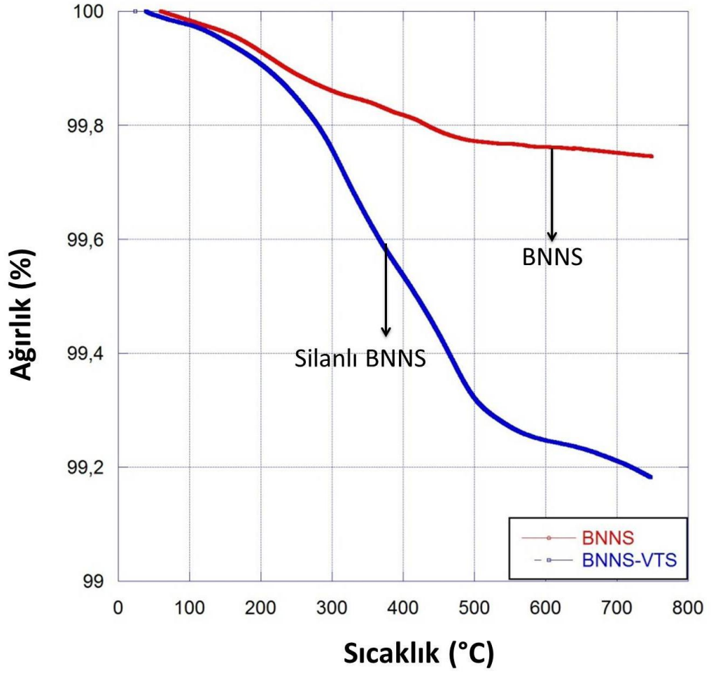
Şekil 4.34. Silanlı ve silansız BNNS'e ait TGA sonuçları
